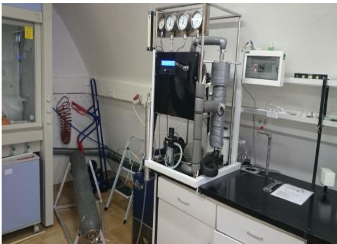
Slika 20. Uređaj za ekstrakciju superkričnim CO 2 (Aladić, 2015)
