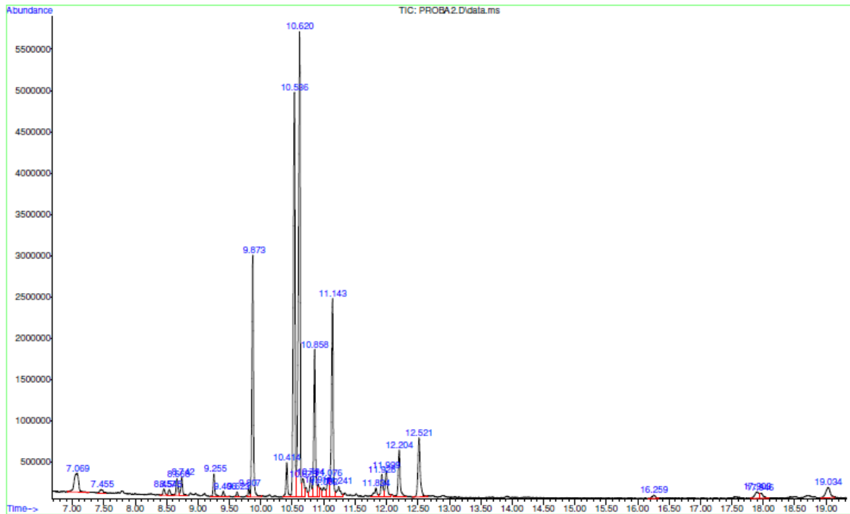
Slika 29. Primjer kromatograma za eterično ulje konopljike
