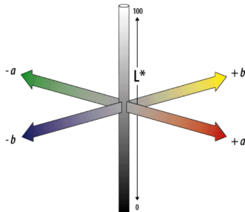
Slika 3. Prikaz boja u L^*a^*b prostoru boja ( http://...cielab.html )
