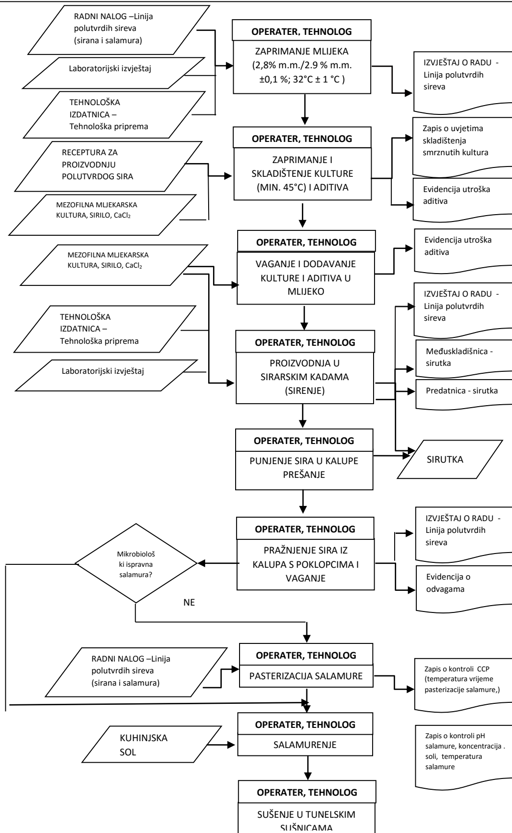
Slika 9 Proizvodnja polutvrđog sira –proizvodnja u sirarskim kadama i prešanje
