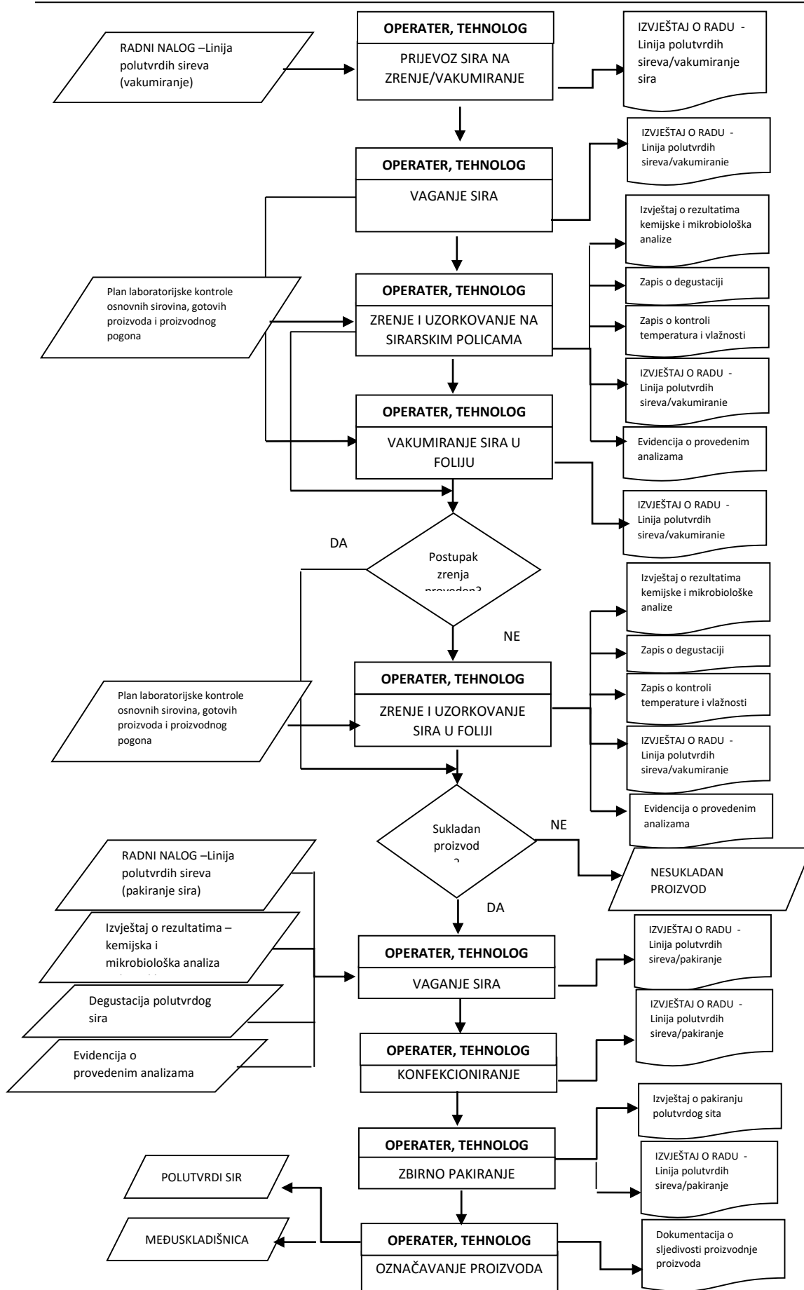
Slika 10 Dijagram toka procesa proizvodnje polutvrđih sireva – skladištenje i zrenje
