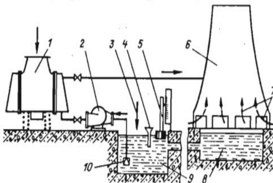
Slika 3 Zatvoreni rashladni sustav s rashladnim tornjem: 1-kondenzator, 2-pumpa za rashladnu vodu, 3-dodavanje vode, 4-uvođenje klorinacije, 5-pokazivač razine, 6-rashladni toranj, 7-ulaz atmosferskog zraka u rashladni toranj, 8-sabirni bazen, 9-sabirni kanal, 10-nepovratni ventil pumpe (Guzović, 1996).
