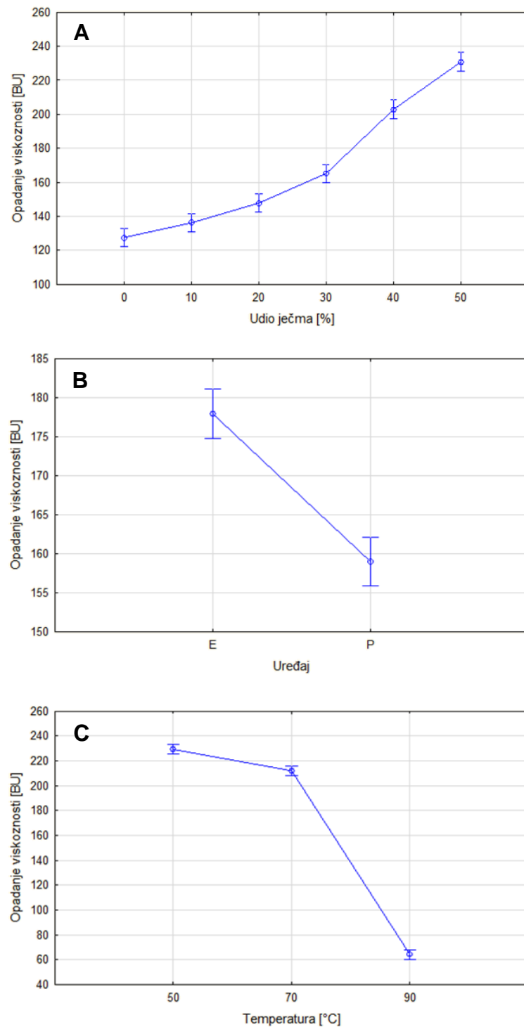
Slika 67 Grafički prikaz rezultata statističke obrade utjecaja udjela ječma (A), vrste uređaja (B) i temperature sušenja (C) na opadanje viskoznosti uzoraka sušene tjestenine proizvedene na ekstruderu (E) i preši (P) (raspon za svaku vrijednost predstavlja standardnu grešku)
