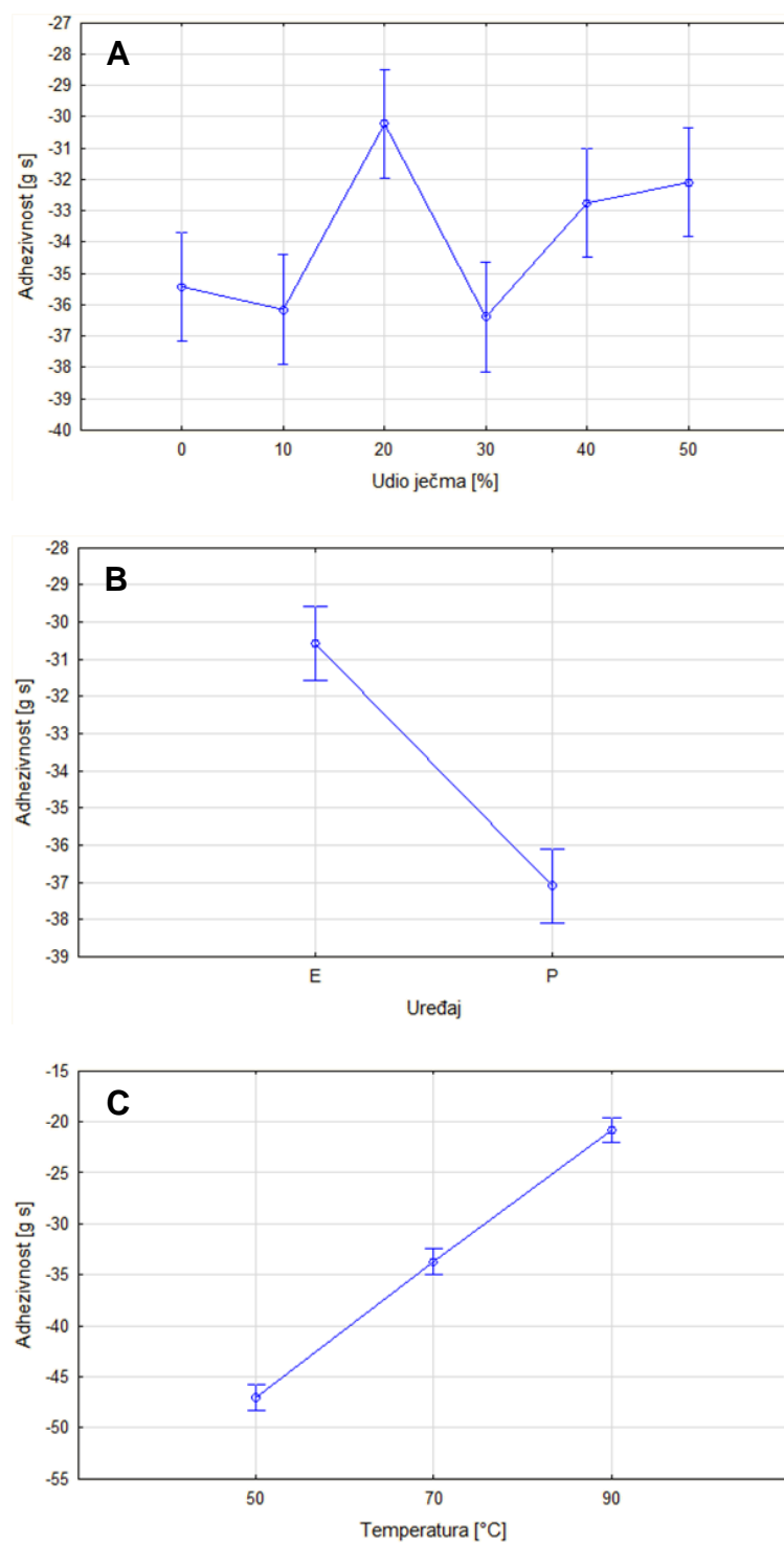
Slika 28 Grafički prikaz rezultata statističke obrade utjecaja udjela ječma (A), vrste uređaja (B) i temperature sušenja (C) na adhezivnost uzoraka tjestenine proizvedene na ekstruderu (E) i preši (P) (raspon za svaku vrijednost predstavlja standardnu grešku)
