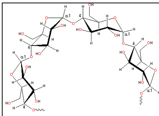
Slika 4 Amiloza (Chaplin, 2007)
