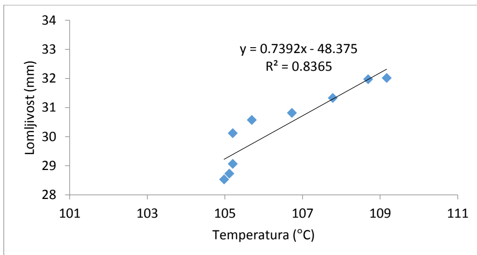
Slika 23 Rezultati usporedbe lomljivosti i temperature izmjerene u središtu čajnog peciva tijekom posljednje minute pečenja kod šećera granulacije manje od 800 \mu\text{m} (Pearsonov koeficijent korelacije: 0,915)
