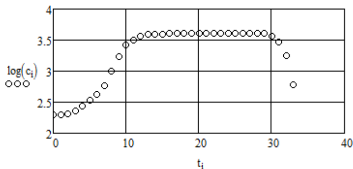
Slika 3. Grafički prikaz logaritmiranih vrijednosti simuliranih podataka.
