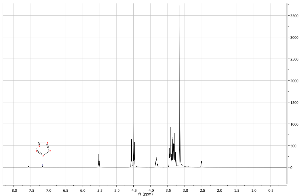
Slika 2. ^1\text{H} NMR spektar smjese tiofena, n -heksana i [kolin-klorid – glicerola] (1:2)
