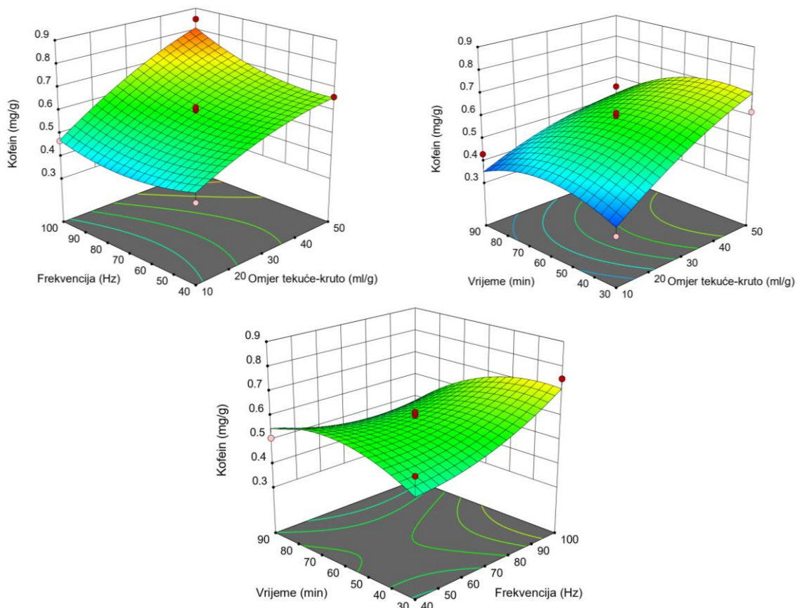
Slika 41 Trodimenzionalni dijagram odzivnih površina kofeina u ovisnosti o frekvenciji, omjeru tekuće/kruto i vremenu ekstrakcije pri ekstrakciji primjenom visokonaponskog električnog pražnjenja
