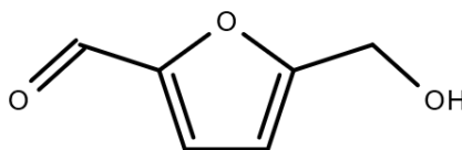
Slika 11 Struktura HMF-a
