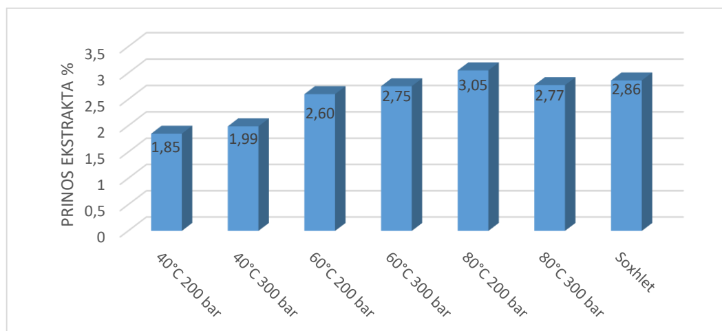
Slika 52 Usporedba prinosa ekstrakta dobiven superkričnom CO 2 ekstrakcijom pri različitim procesnim uvjetima i Soxhlet ekstrakcijom sa heksanom
