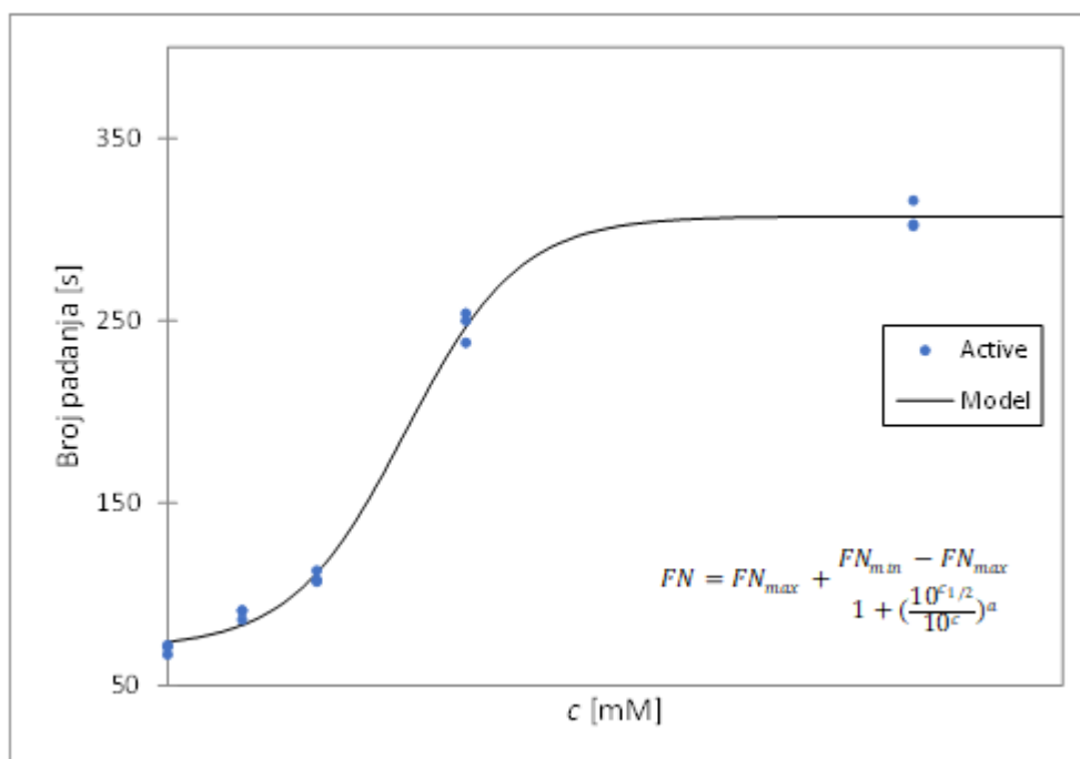
Slika 7 Primjer primjene sigmoidalnog modela ovisnosti broja padanja o promijeni koncentracije inhibicijske otopine
