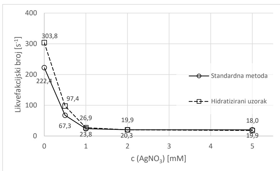
Slika 11 Utjecaj inaktivacije amilolitičkih enzima srebrovim nitratom na likvefakcijski broj
