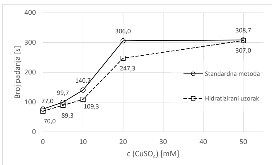
Slika 10 Utjecaj inaktivacije amilolitičkih enzima bakrovim sulfatom na broj padanja
