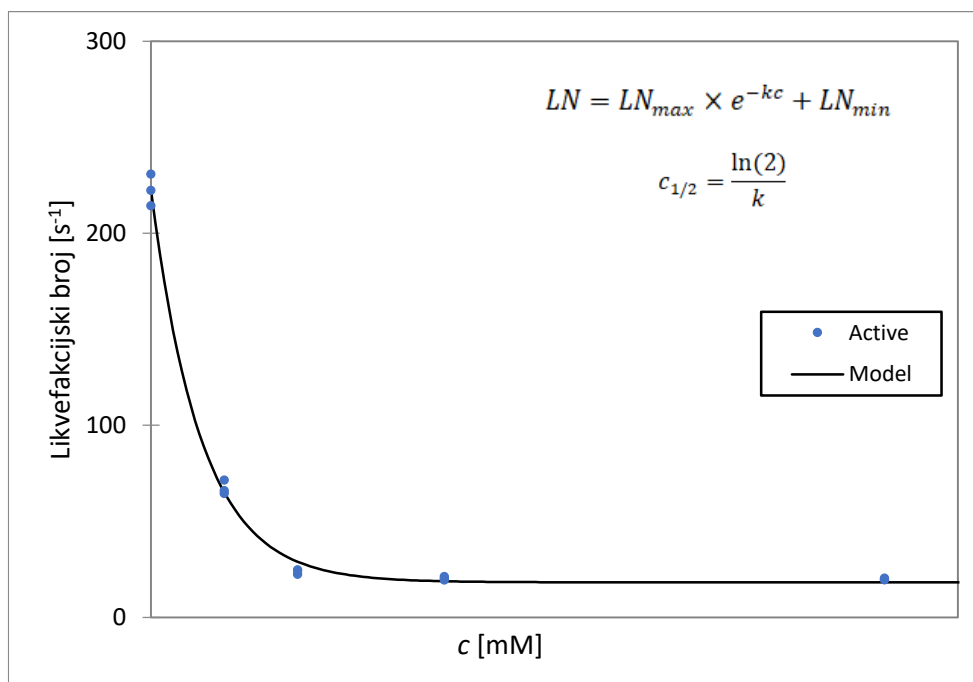
Slika 8 Primjer primjene modela eksponencijalnog pada ovisnosti likvefakcijskog broja o promijeni koncentracije inhibicijske otopine
