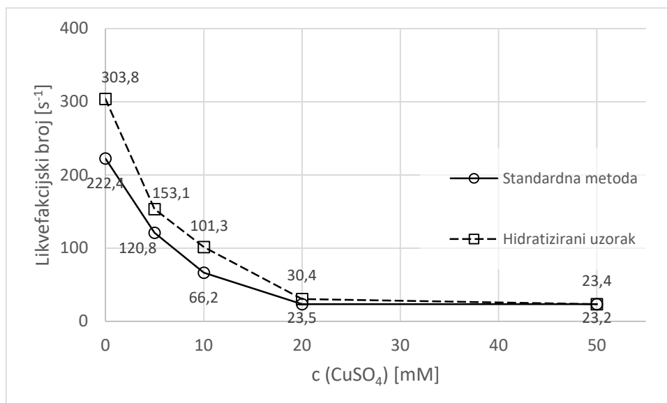
Slika 12 Utjecaj inaktivacije amilolitičkih enzima bakrovim sulfatom na likvefakcijski broj
