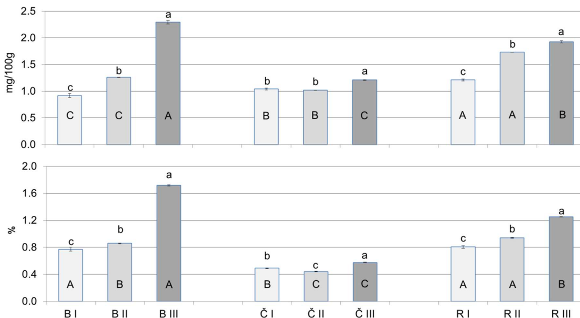
Slika 19 Koncentracije i relativni udjeli eritrodiole u djevičanskim maslinovim uljima proizvedenim od maslina sorti Buža (B), Črna (Č) i Rosinjola (R) ubranih u tri različita stupnja zrelosti (I-III) (mala slova – statistički značajne razlike između stupnjeva zrelosti iste sorte, velika slova - statistički značajne razlike između sorti istog stupnja zrelosti, LSD test, p < 0,05 )
