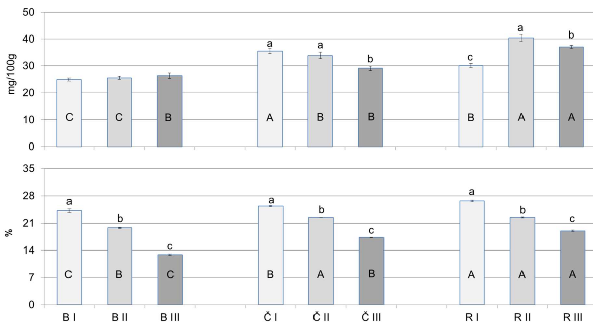
Slika 47 Prosječne koncentracije i relativni udjeli (n=2) ukupnih 4-monometil-sterola u djevičanskim maslinovim uljima proizvedenim od maslina sorti Buža (B), Črna (Č) i Rosinjola (R) ubranih u tri različita stupnja zrelosti (I-III) (mala slova – statistički značajne razlike između stupnjeva zrelosti iste sorte, velika slova - statistički značajne razlike između sorti istog stupnja zrelosti, LSD test, p < 0,05 )
