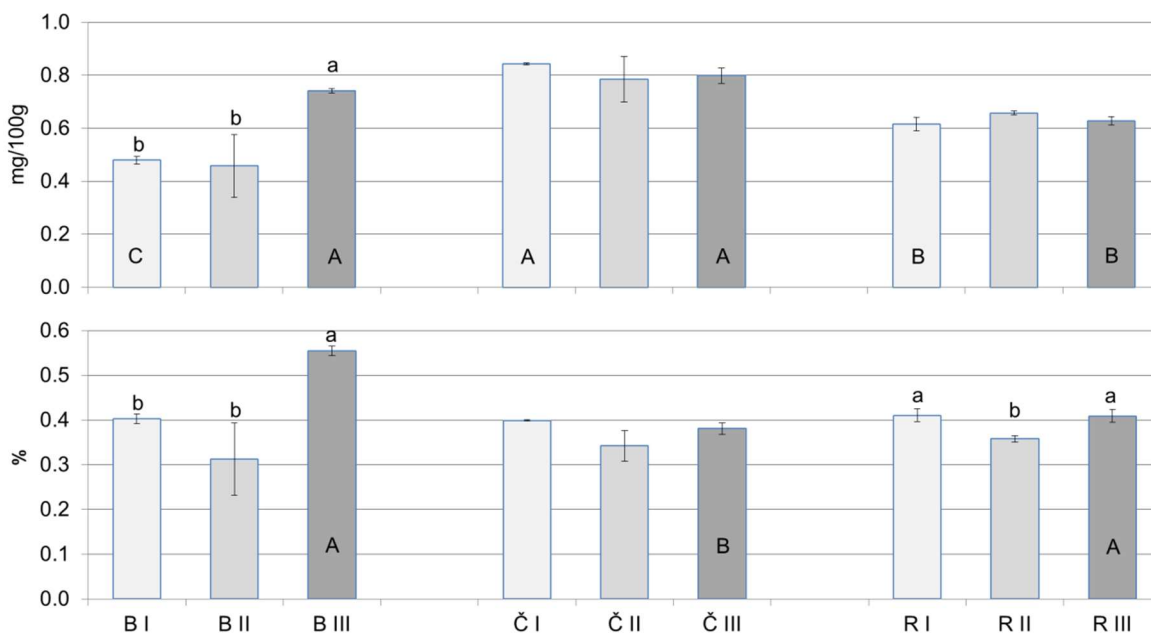
Slika 20 Koncentracije i relativni udjeli uvaole u djevičanskim maslinovim uljima proizvedenim od maslina sorti Buža (B), Črna (Č) i Rosinjola (R) ubranih u tri različita stupnja zrelosti (I-III) (mala slova – statistički značajne razlike između stupnjeva zrelosti iste sorte, velika slova - statistički značajne razlike između sorti istog stupnja zrelosti, LSD test, p < 0,05 )
