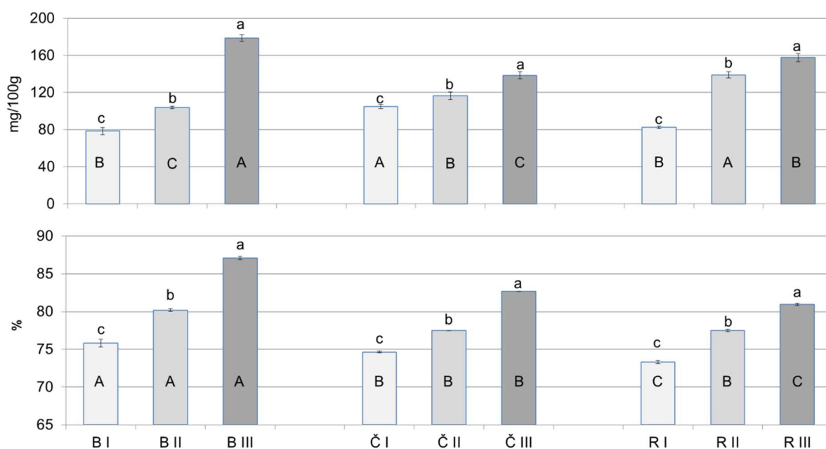
Slika 48 Prosječne koncentracije i relativni udjeli (n=2) ukupnih 4,4-dimetil-sterola u djevičanskim maslinovim uljima proizvedenim od maslina sorti Buža (B), Črna (Č) i Rosinjola (R) ubranih u tri različita stupnja zrelosti (I-III) (mala slova – statistički značajne razlike između stupnjeva zrelosti iste sorte, velika slova - statistički značajne razlike između sorti istog stupnja zrelosti, LSD test, p < 0,05 )
