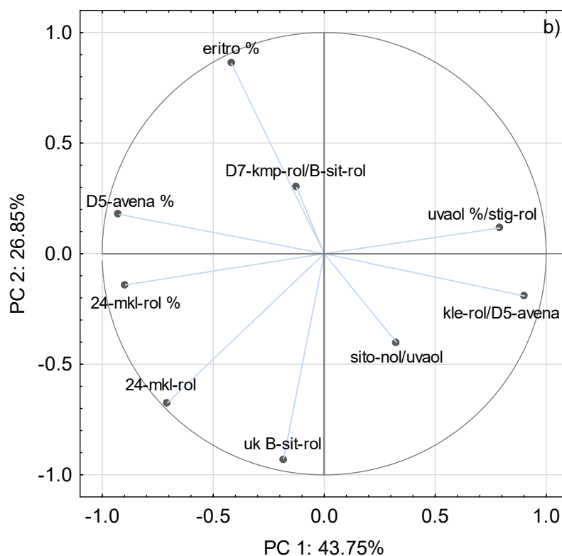
Slika 25 (a) Razdvajanje na osnovi stupnja zrelosti (nenadzirano, PCA) svježih maslinovih ulja sorti Buža, Črna i Rosinjola u dvodimenzionalnom prostoru definiranom s glavnim sastavnicama PC1 i PC2; (b) Projekcija faktorskih opterećenja odabranih varijabli (koncentracija sterola i triterpenskih diola u mg/kg, odnosno njihovih relativnih udjela označenih s „%“) uzduž smjerova PC 1 i PC 2
