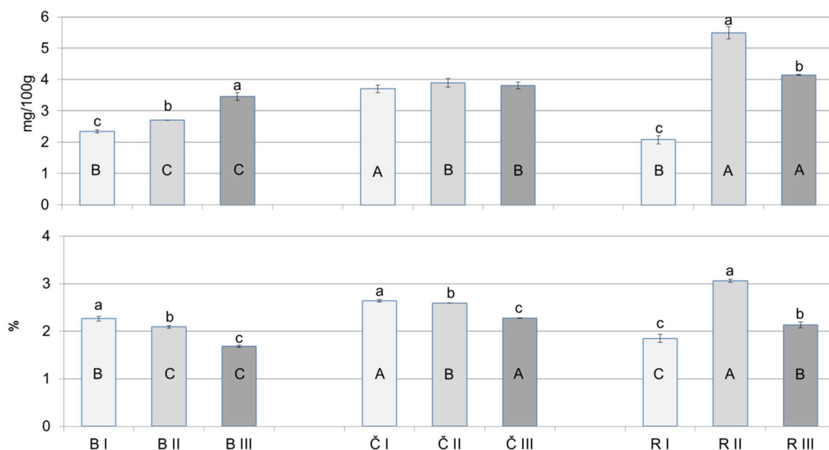
Slika 43 Prosječne koncentracije i relativni udjeli ( n=2 ) sume gramisterol + cikloelukalenol u djevičanskim maslinovim uljima proizvedenim od maslina sorti Buža (B), Črna (Č) i Rosinjola (R) ubranih u tri različita stupnja zrelosti (I-III) (mala slova – statistički značajne razlike između stupnjeva zrelosti iste sorte, velika slova - statistički značajne razlike između sorti istog stupnja zrelosti, LSD test, p < 0,05 )
