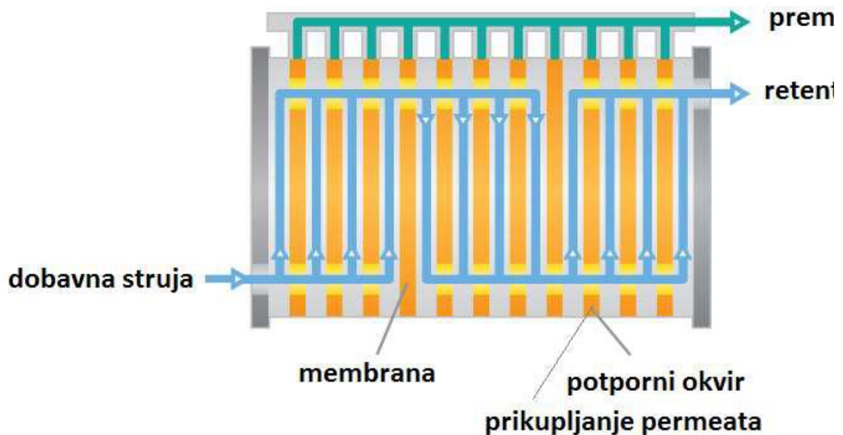
Slika 4 Princip rada filter - preše (Habuda - Stanić, 2021)
