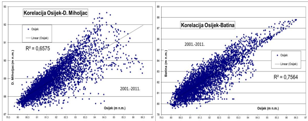
Slika 5. Korelacija vrijednosti zabilježenih istodnevnih vodostaja Drave kod Osijeka s uzvodnim vodostajima rijeke Drava i Dunav
