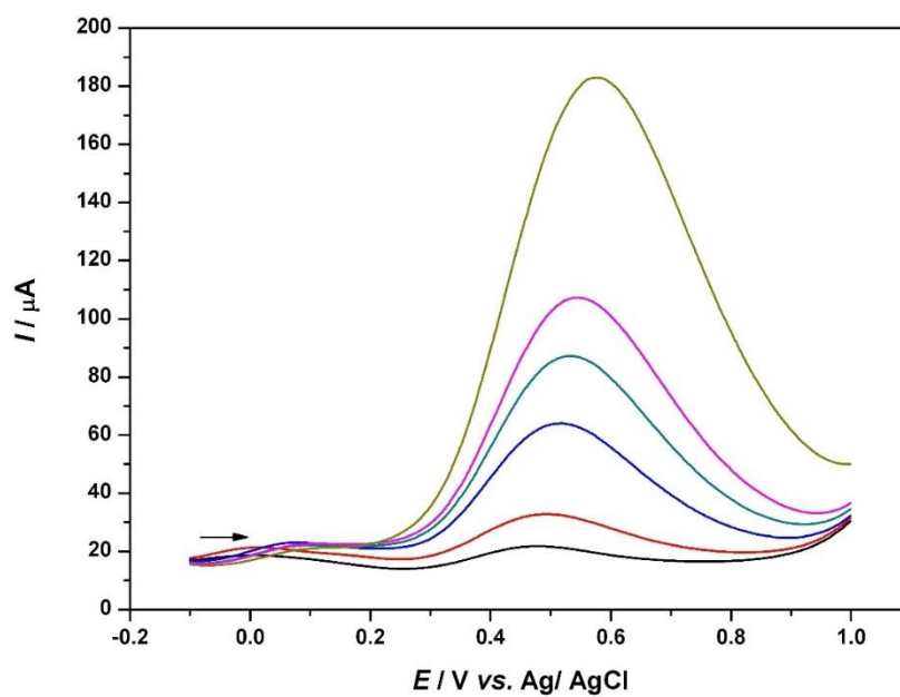
Slika 15 Pravokutnovalni voltamogrami vitamina C ( \gamma = 5 - 200 mg L -1 ) dobivena prema eksperimentalnim uvjetima iz Tablice 3
