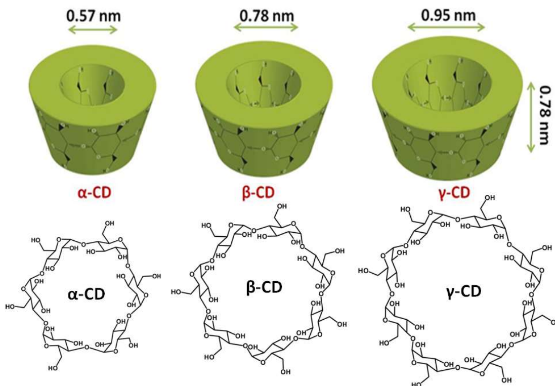
Slika 8. Prikaz strukture ciklodekstrina (web 2)
