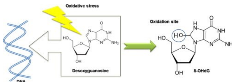
Slika 2 Formiranje 8-OHdG-a
