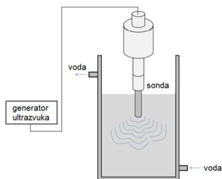
Slika 5 Diskontinuirani ultrazvučni ekstraktor sa sondom (Tiwari, 2015)
