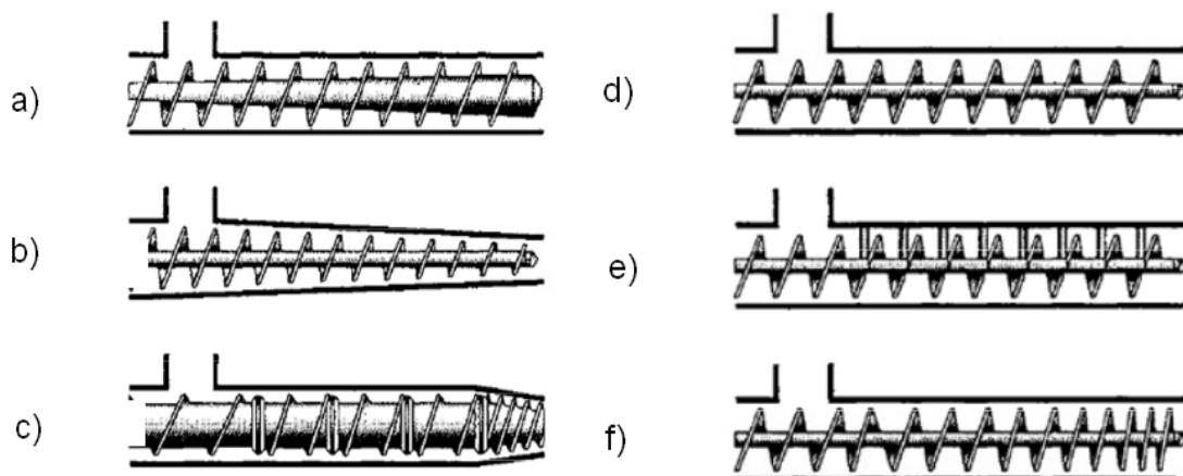
Slika 1 Tipovi puža i kućišta kod jednpužnih ekstrudera (Rokey, 2000.)
