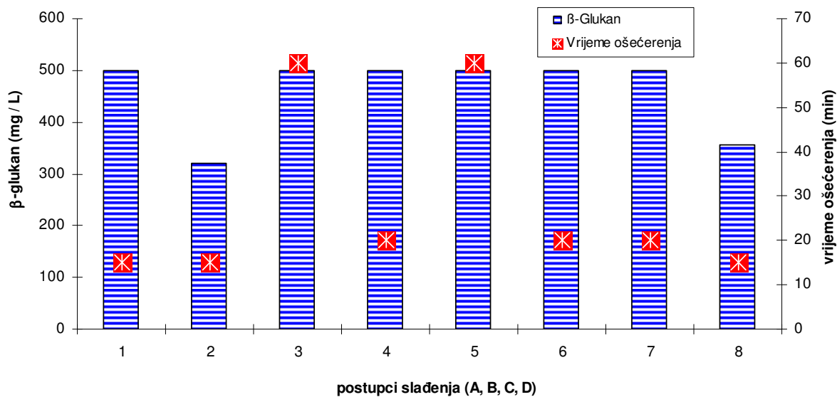
Slika 12 Međusobni odnos \beta -glukana i vremena ošećerenja sladovina po provedenim postupcima slađenja (A, B, C, D)
