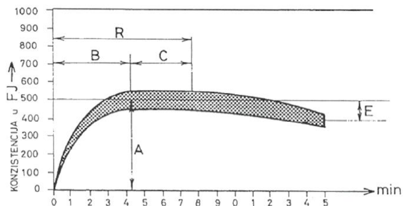
Slika 16 Farinogram (Đaković, 1980.)
