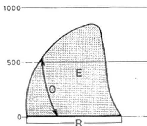
Slika 18 Ekstenzogram (Đaković, 1980.)
