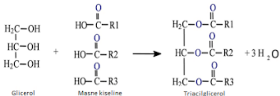
Slika 1 Primjer nastajanja molekule triacilglicerola
