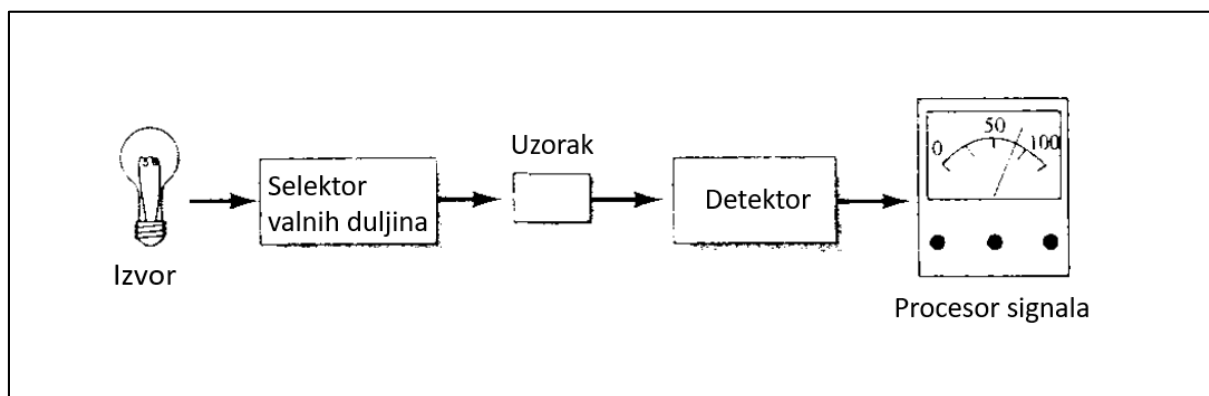
Slika 5 Jednostopni spektroskopski instrument (Skoog i sur., 2007)
