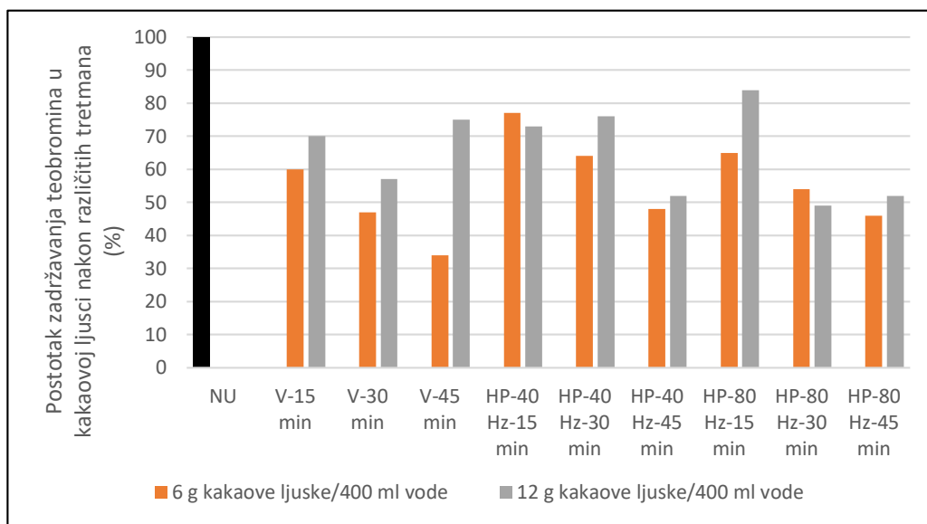
Slika 15 Zadržavanje teobromina u kakaovoj ljsuci nakon različitih tretmana u usporedbi s netretiranim uzorkom (NU)
