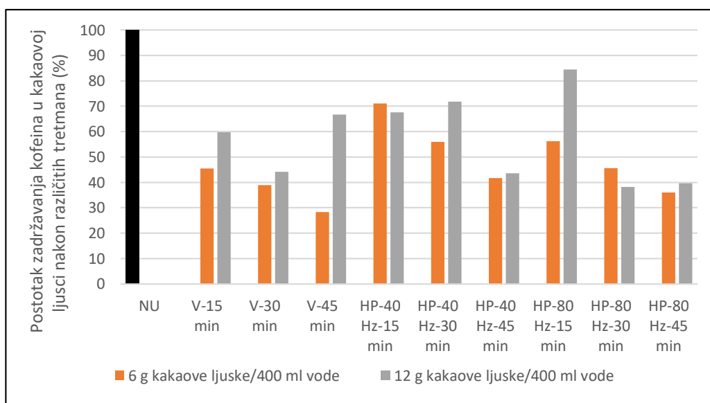
Slika 16 Zadržavanje kofeina u kakaovoj ljsuci nakon različitih tretmana u usporedbi s netretiranim uzorkom (NU)
