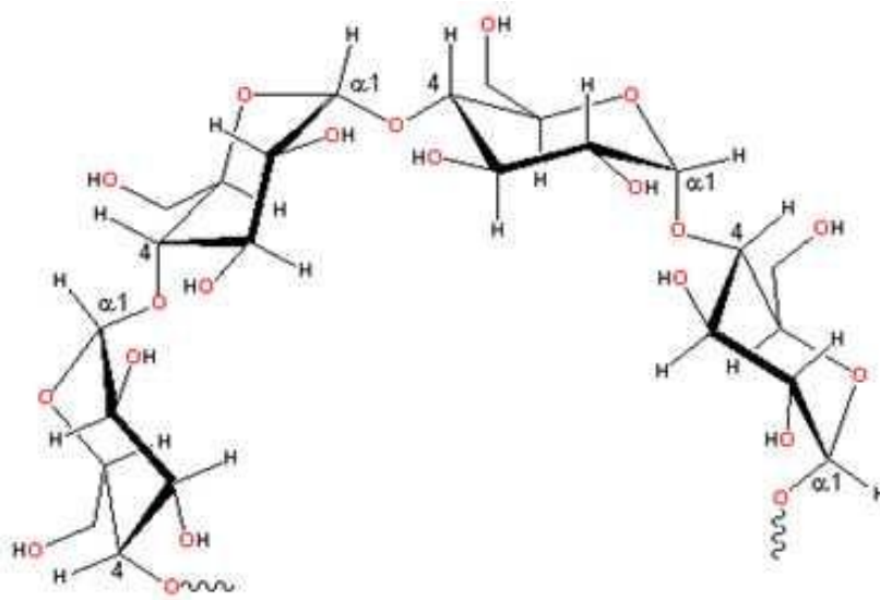
Slika 4 Struktura amiloze (web 4)
