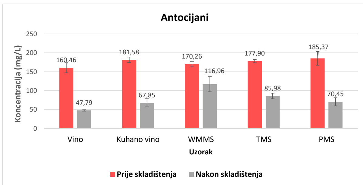
Slika 17 Sadržaj antocijana u početnom vinu, kuhanom vinu i kremama od vina s dodatkom modificiranih škrobova kukuruza (WMMS), tapioke (TMS) i krumpira (PMS) prije i nakon tromjesečnog skladištenja
