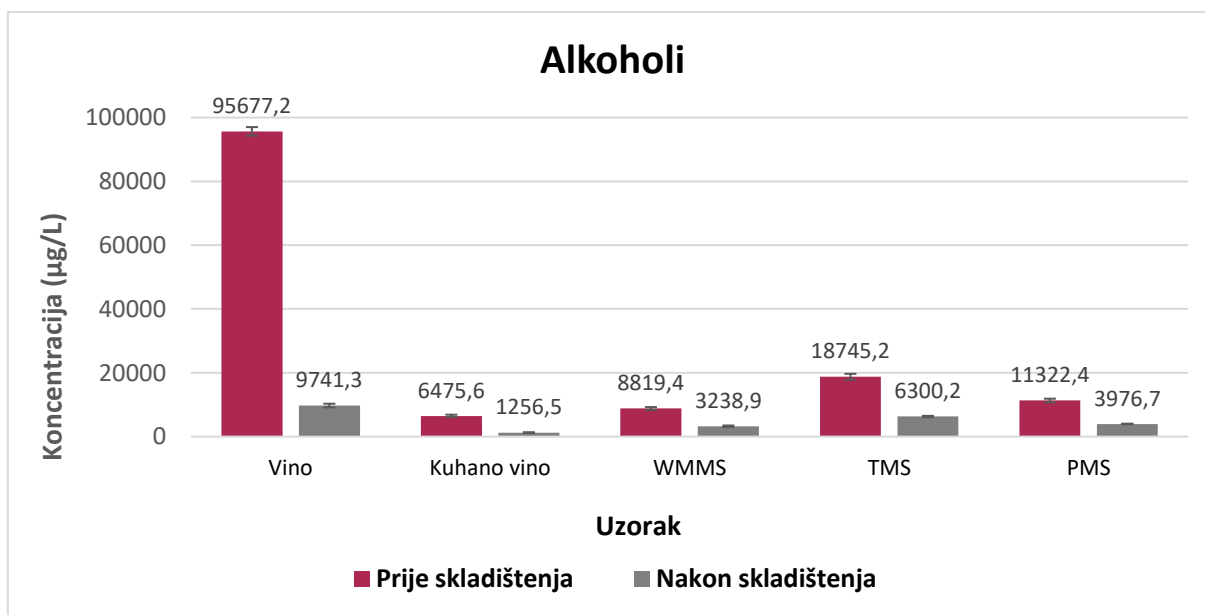
Slika 10 Sadržaj viših alkohola u početnom vinu, kuhanom vinu i kremama od vina s dodatkom modificiranih škrobova kukuruza (WMMS), tapioke (TMS) i krumpira (PMS) prije i nakon tromjesečnog skladištenja
