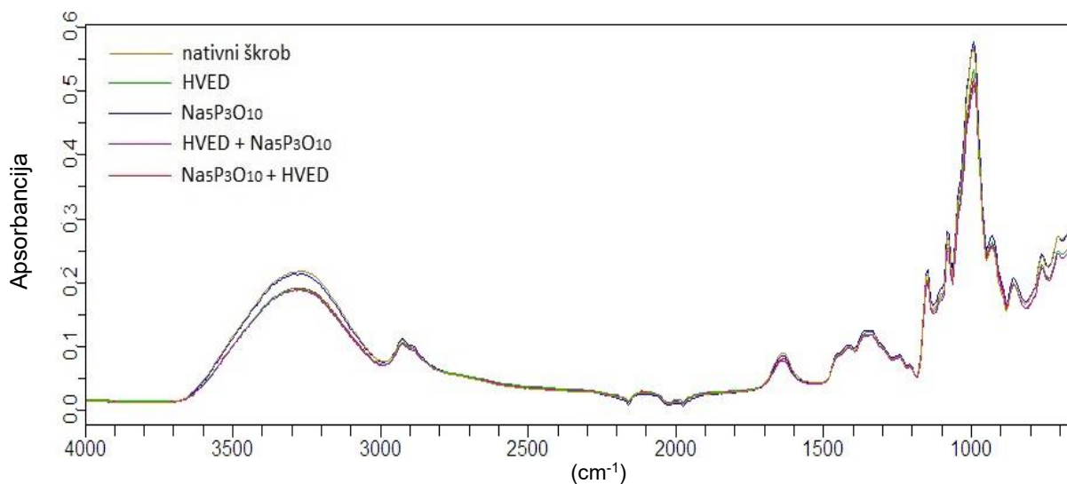
Slika 63 IR-spektar nativnog krumpirovog škroba, škroba modificiranog HVED-om i škroba modificiranog Na 5 P 3 O 10 sa i bez HVED-a
