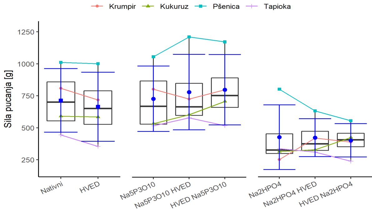
Slika 42 Sila pucanja nativnih škrobova, škrobova modificiranih HVED-om i škrobova modificiranih \text{Na}_5\text{P}_3\text{O}_{10} i \text{Na}_2\text{HPO}_4 sa i bez primjene HVED-a
