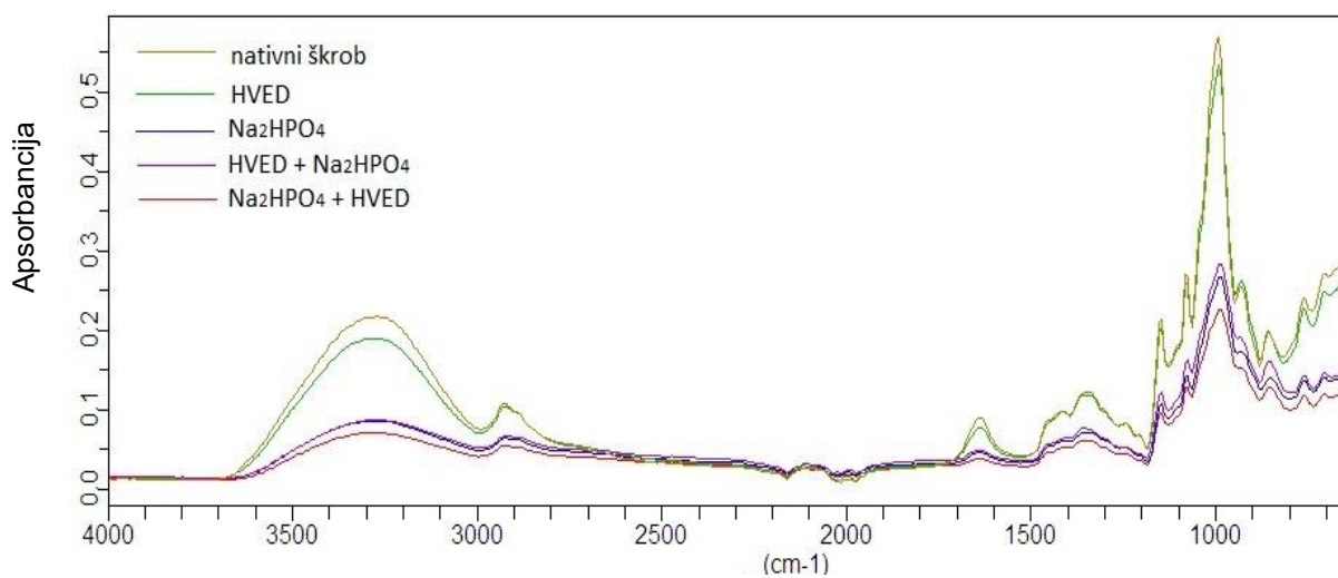
Slika 64 IR-spektar nativnog krumpirovog škroba, škroba modificiranog HVED-om i škroba modificiranog Na 2 HPO 4 sa i bez primjene HVED-a
