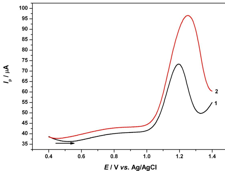
Slika 20 Pravokutnovalni voltamogram obogaćivanja uzorka dodatka prehrani (DF 10) (crno bez dodatka kafeina, crveno s dodatkom kafeina) snimljen pri eksperimentalnim uvjetima kao u Tablici 1
