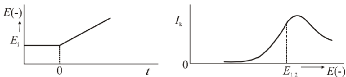
Slika 8 Signal pobude i odziva voltametrije (Piljac, 2010)
