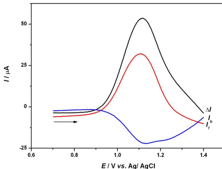
Slika 11 Pravokutnovalni voltamogram standarda kafeina ( c = 1,14 \cdot 10^{-2} \text{ mol L}^{-1} ) kafeina u 0,1 \text{ mol L}^{-1} acetatnom puferu pH 4 snimljen pri eksperimentalnim uvjetima kao u Tablici 1
