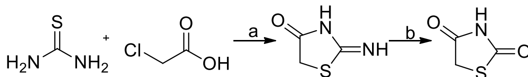
Slika 6 Sinteza tiazolidindiona potpomognuta mikrovalovima: (a) 0 – 5 °C, voda, miješanje; (b) MW-250 W, voda
