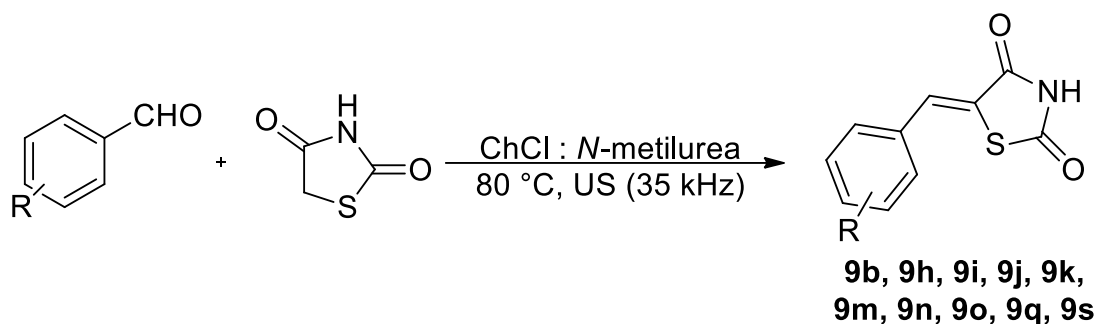
Slika 25 Sinteza derivata tiazolidindiona Knoevenagelovom kondenzacijom potpomognuta ultrazvukom
