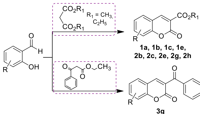
Slika 20 Sinteza derivata kumarina u otapalu \text{ChCl} : urea, potpomognuta mikrovalovima (1400 W) pri 80^\circ\text{C}
