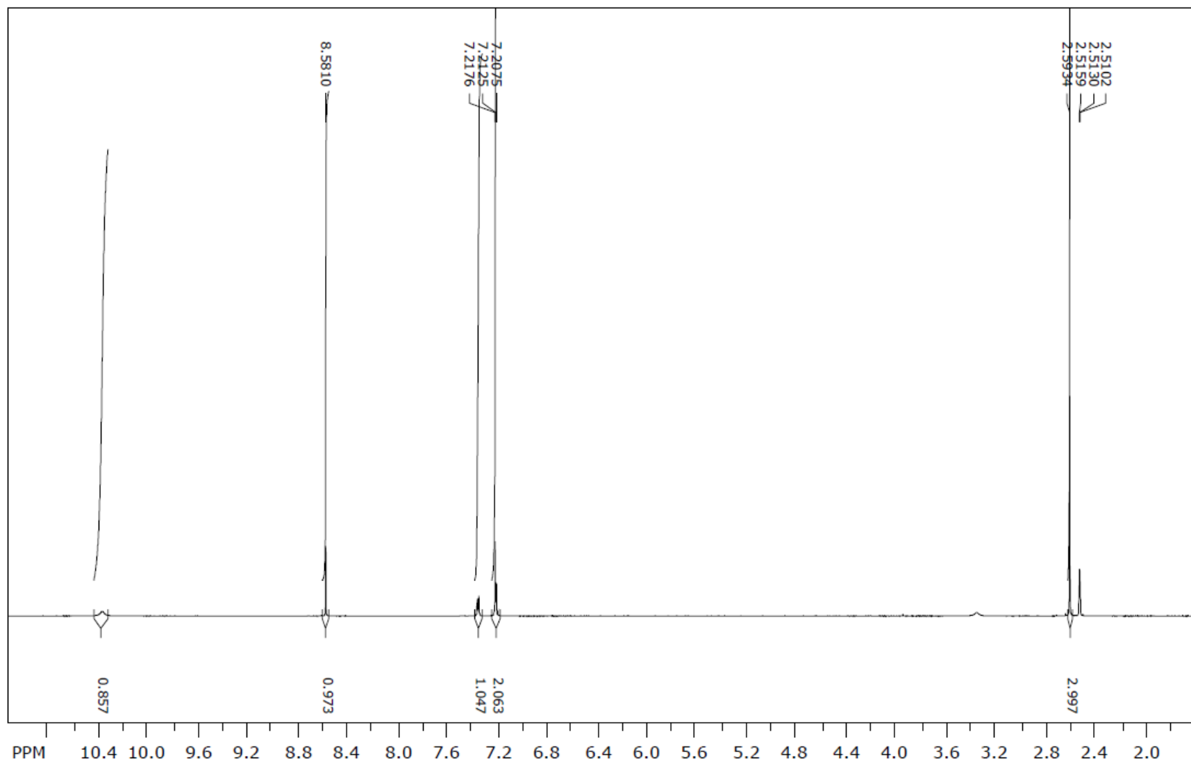
1 H NMR spektar (5a)
