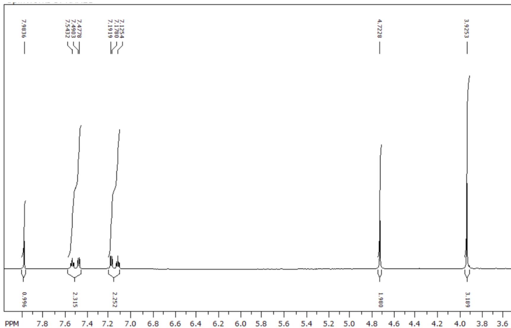
1 H NMR spektr (8j)
