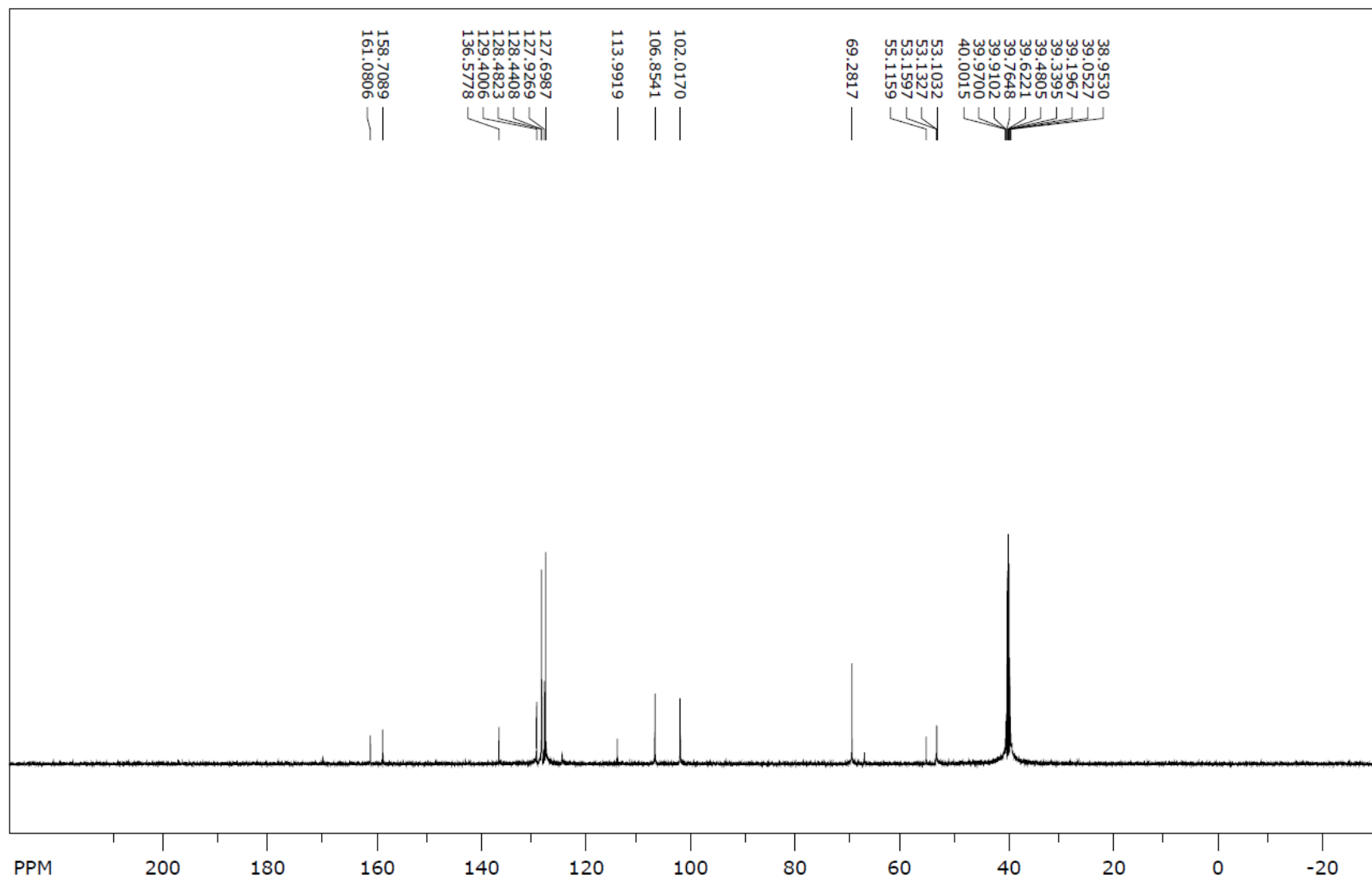
13 C NMR spektr (9o)
