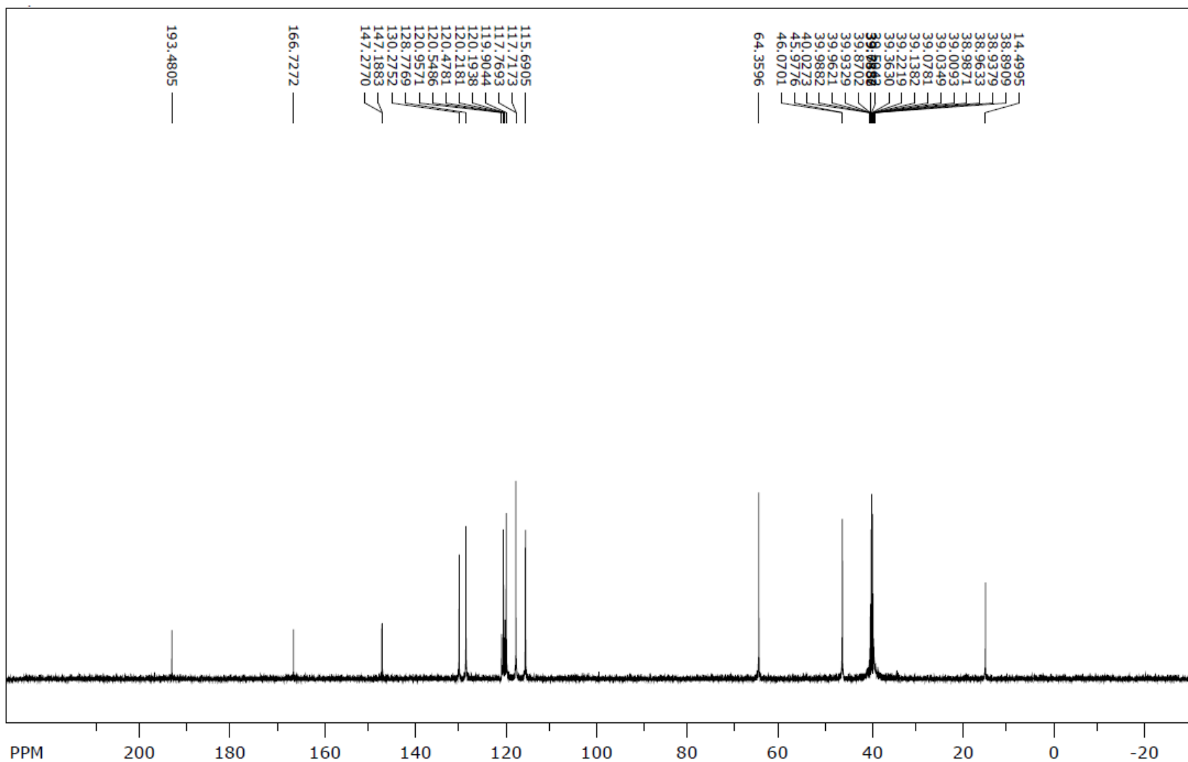
13 C NMR spektr (6e)
