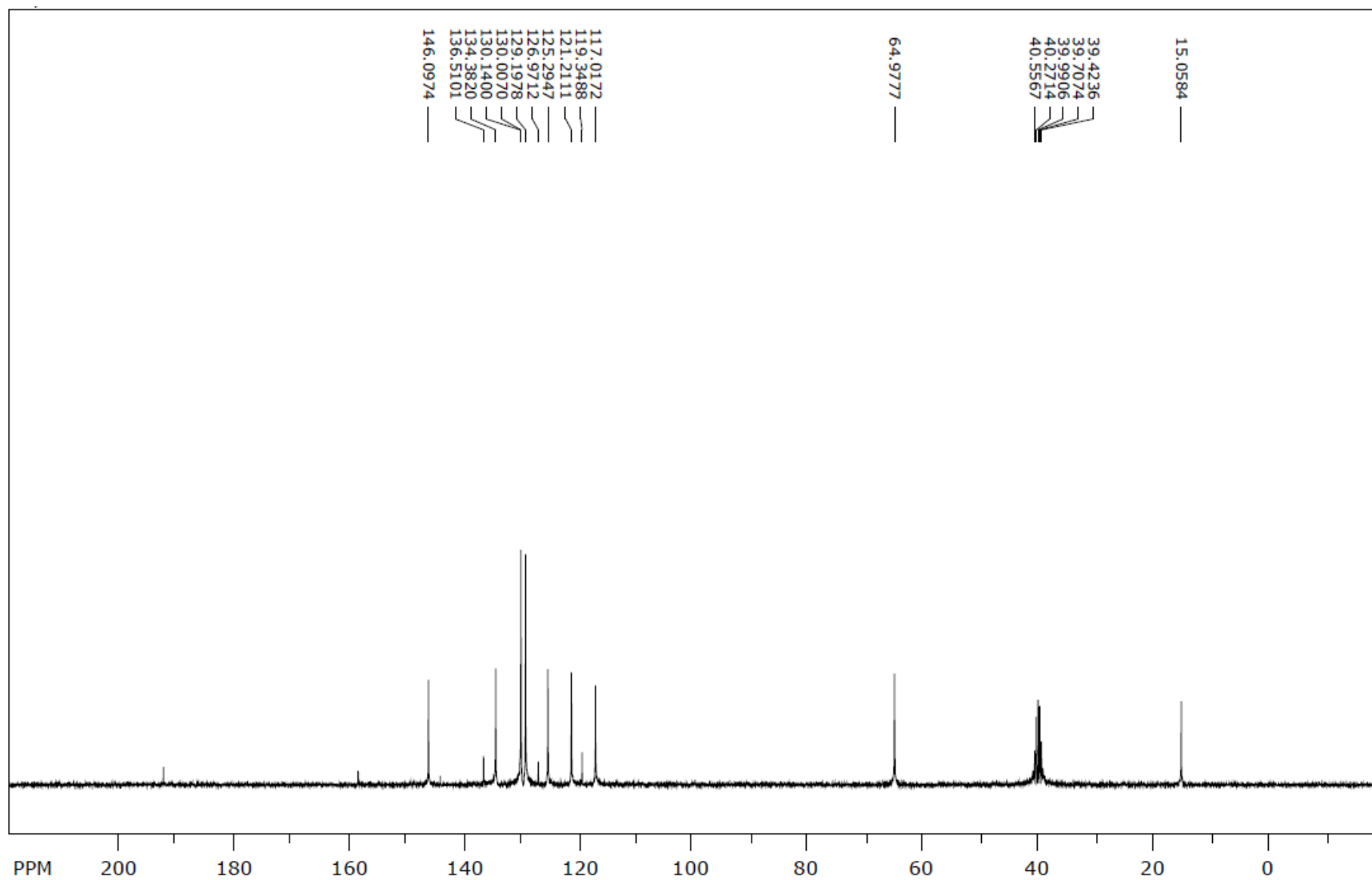
13 C NMR spektr (3e)
