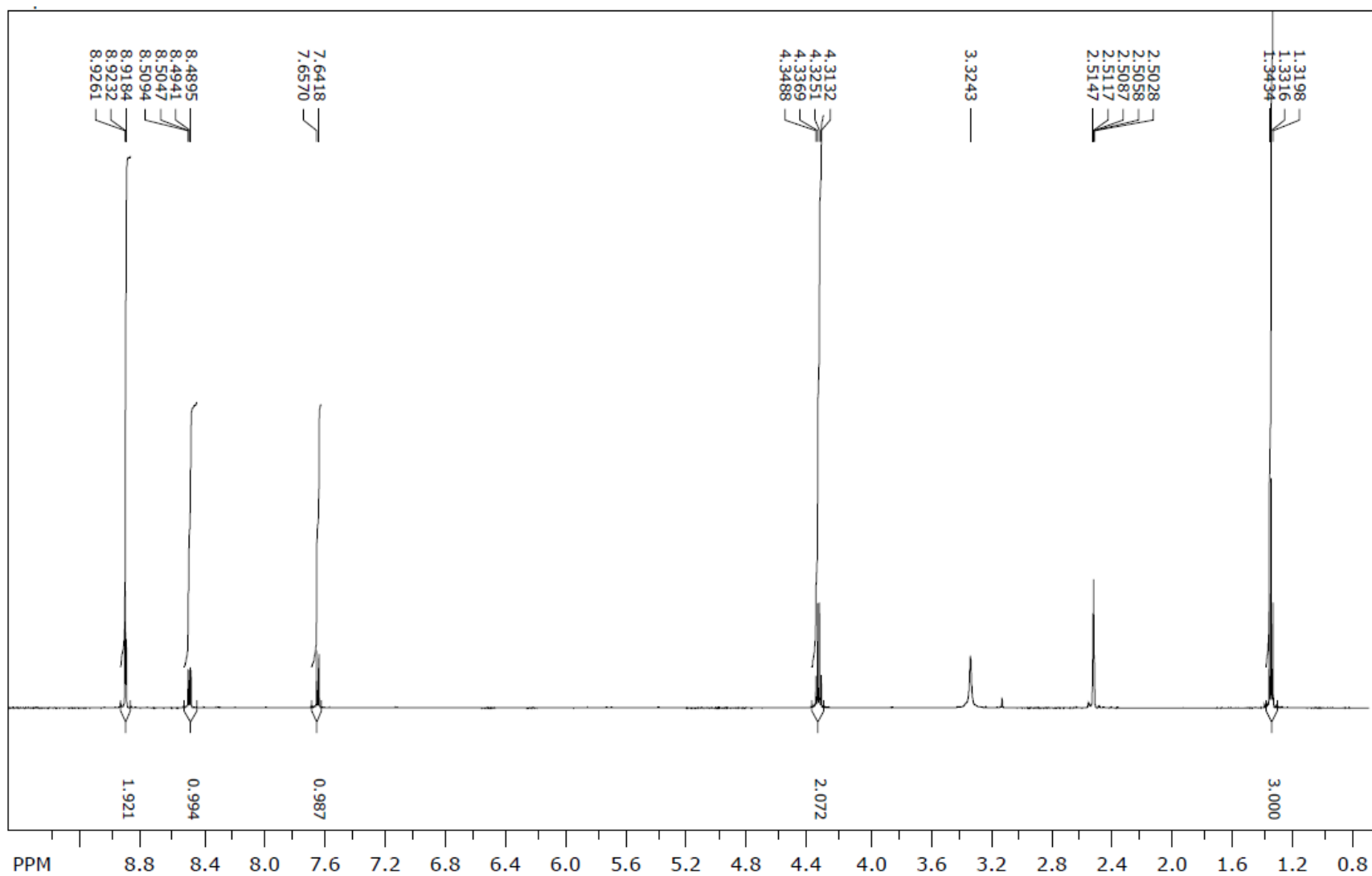
1 H NMR spektr (2f)
