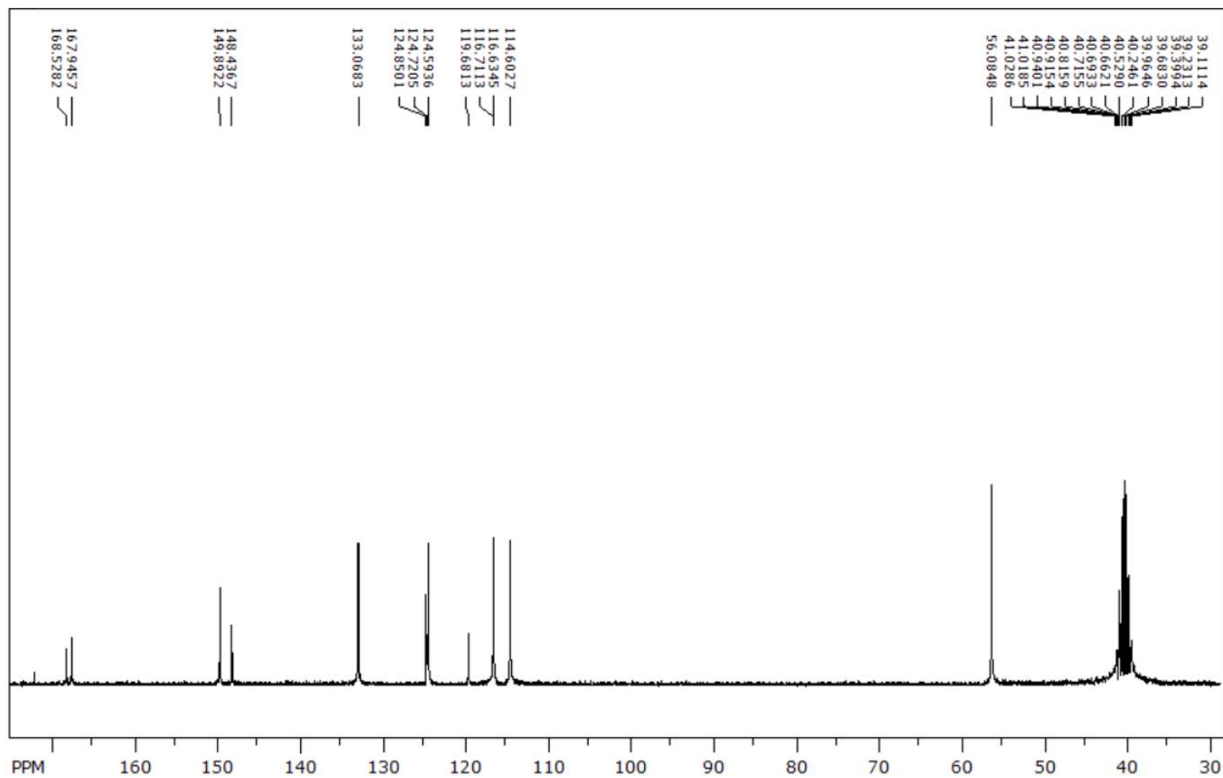
13 C NMR spektr (9b)
