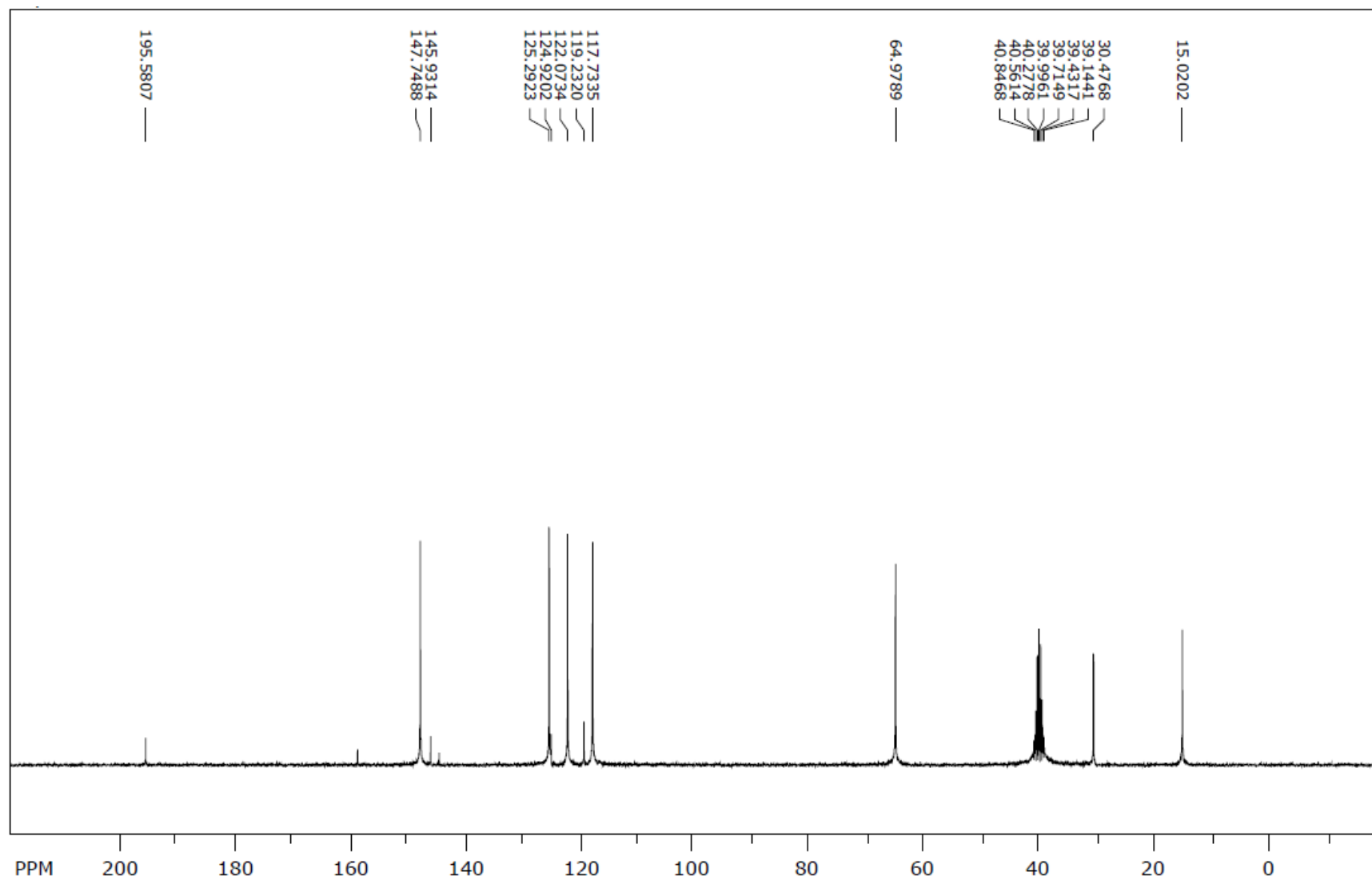
13 C NMR spektr (5f)
