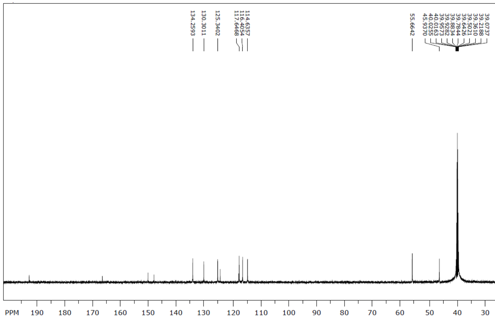
13 C NMR spektr (6c)
