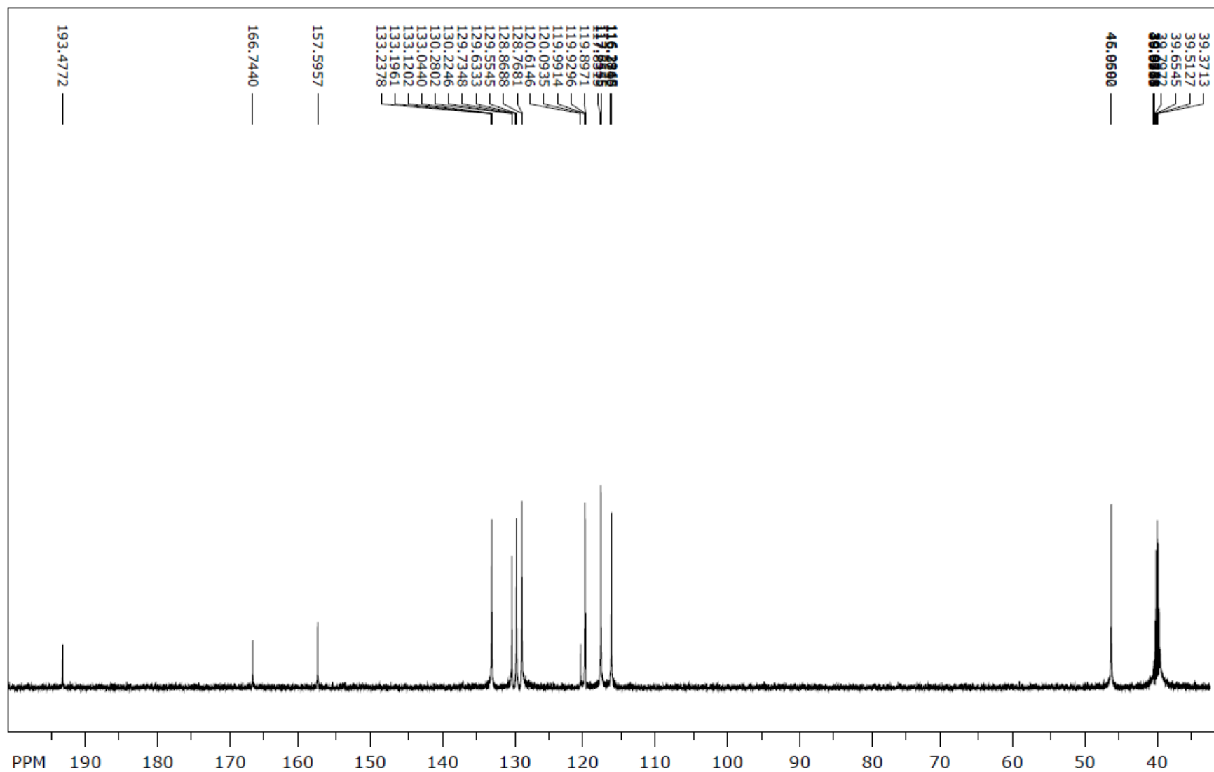
13 C NMR spektr (6a)
