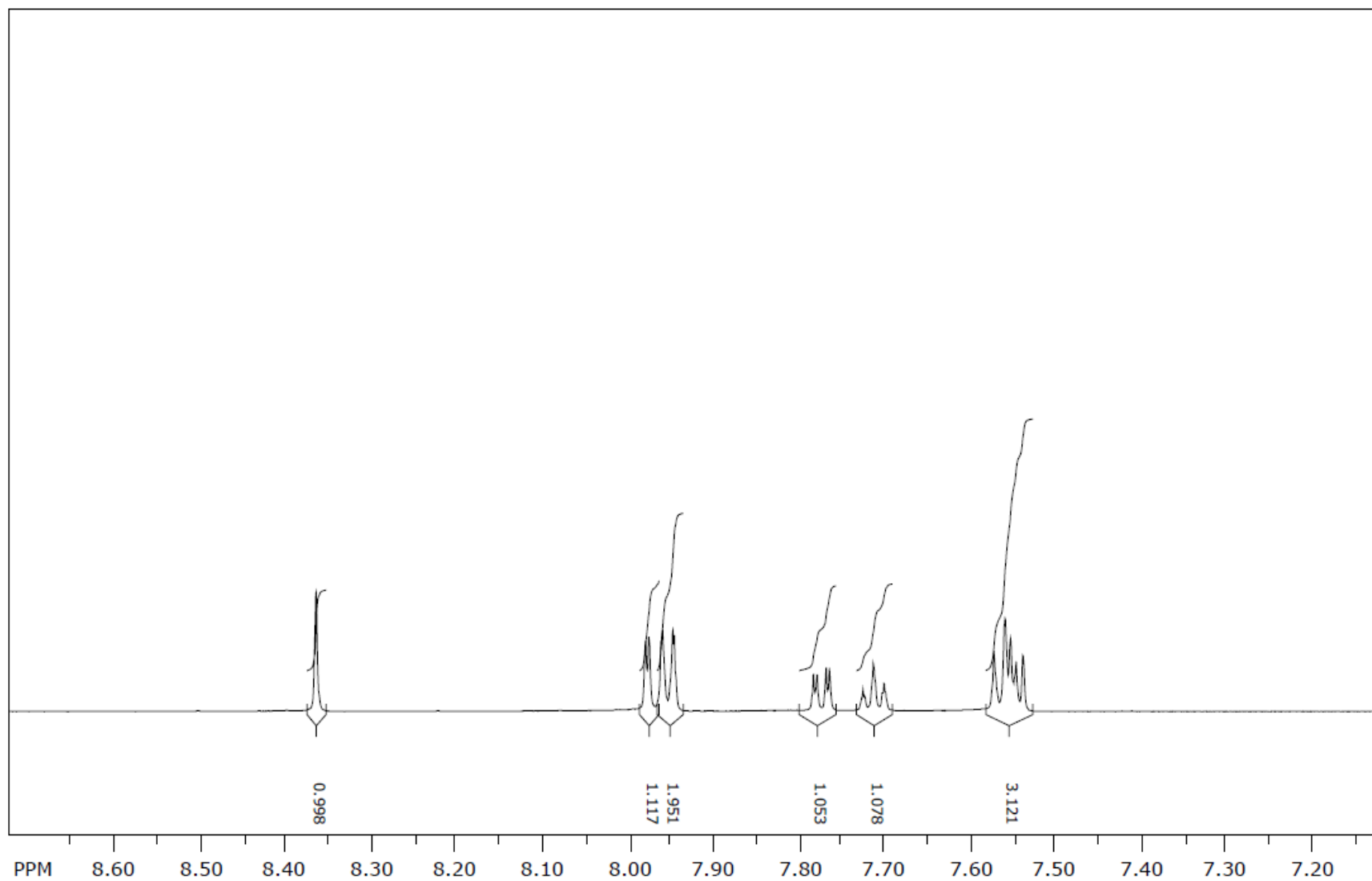
1 H NMR spektr (3f)
