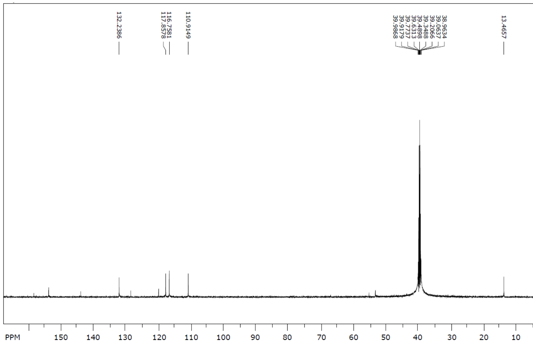
^{13}\text{C} NMR spektr (9c)
