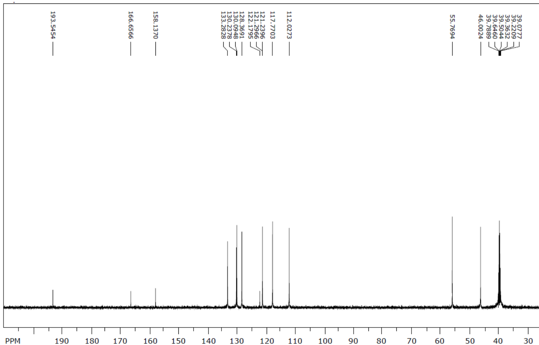
^{13}\text{C} NMR spektr (6o)
