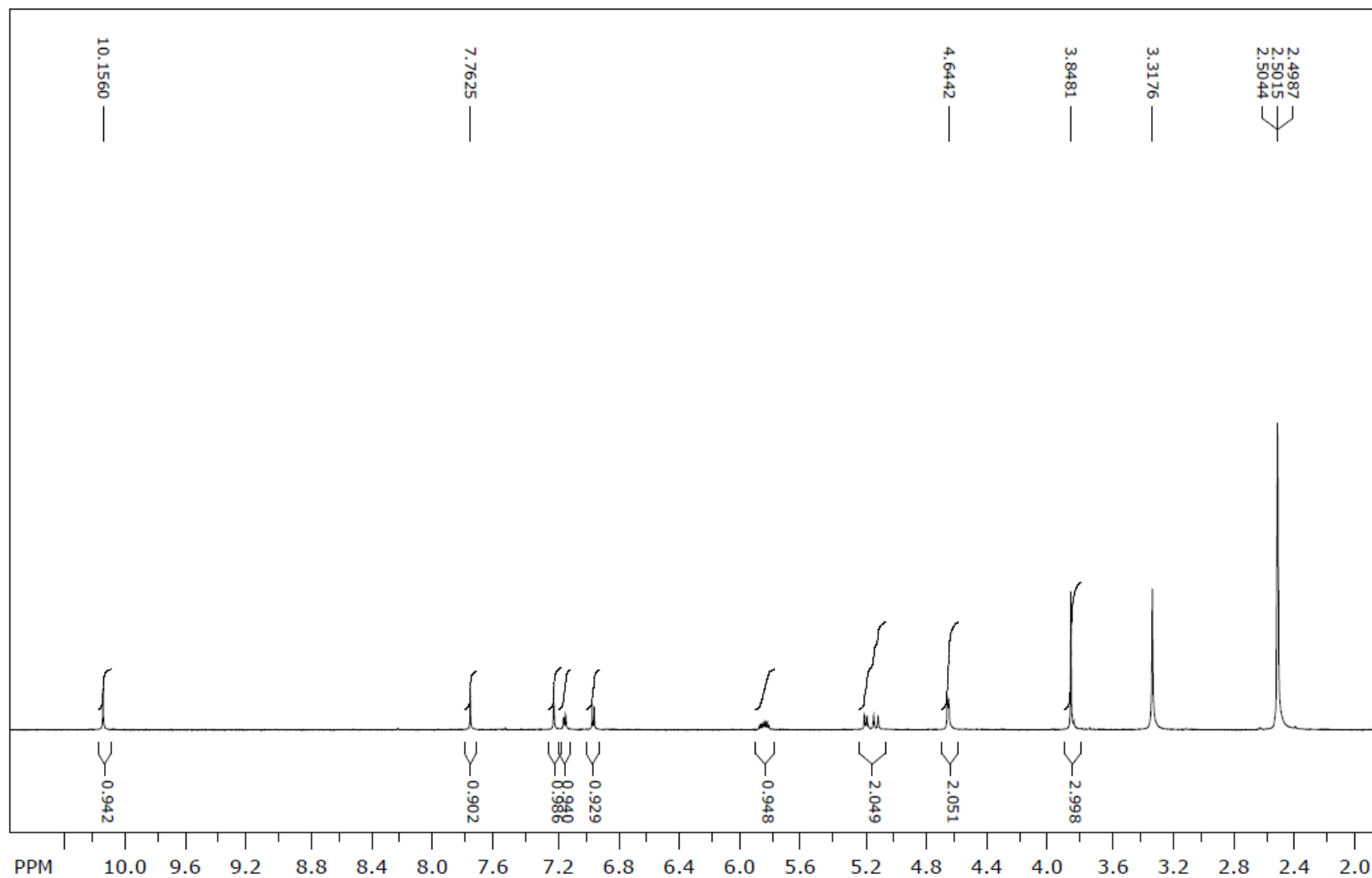
1 H NMR spektr (6c)
