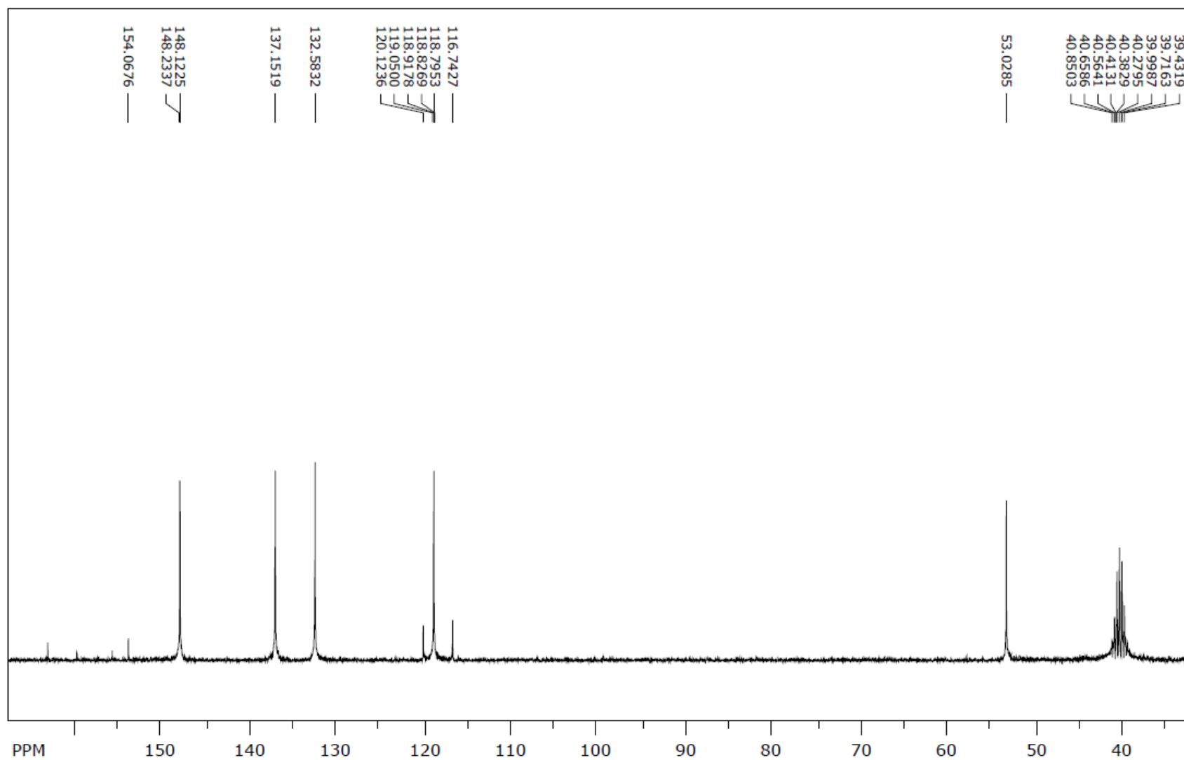
13 C NMR spektr (1b)
