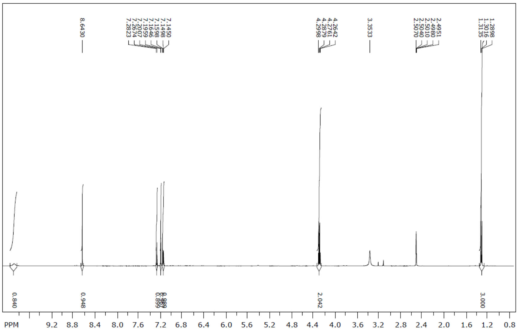
1 H NMR spektar (2c)
