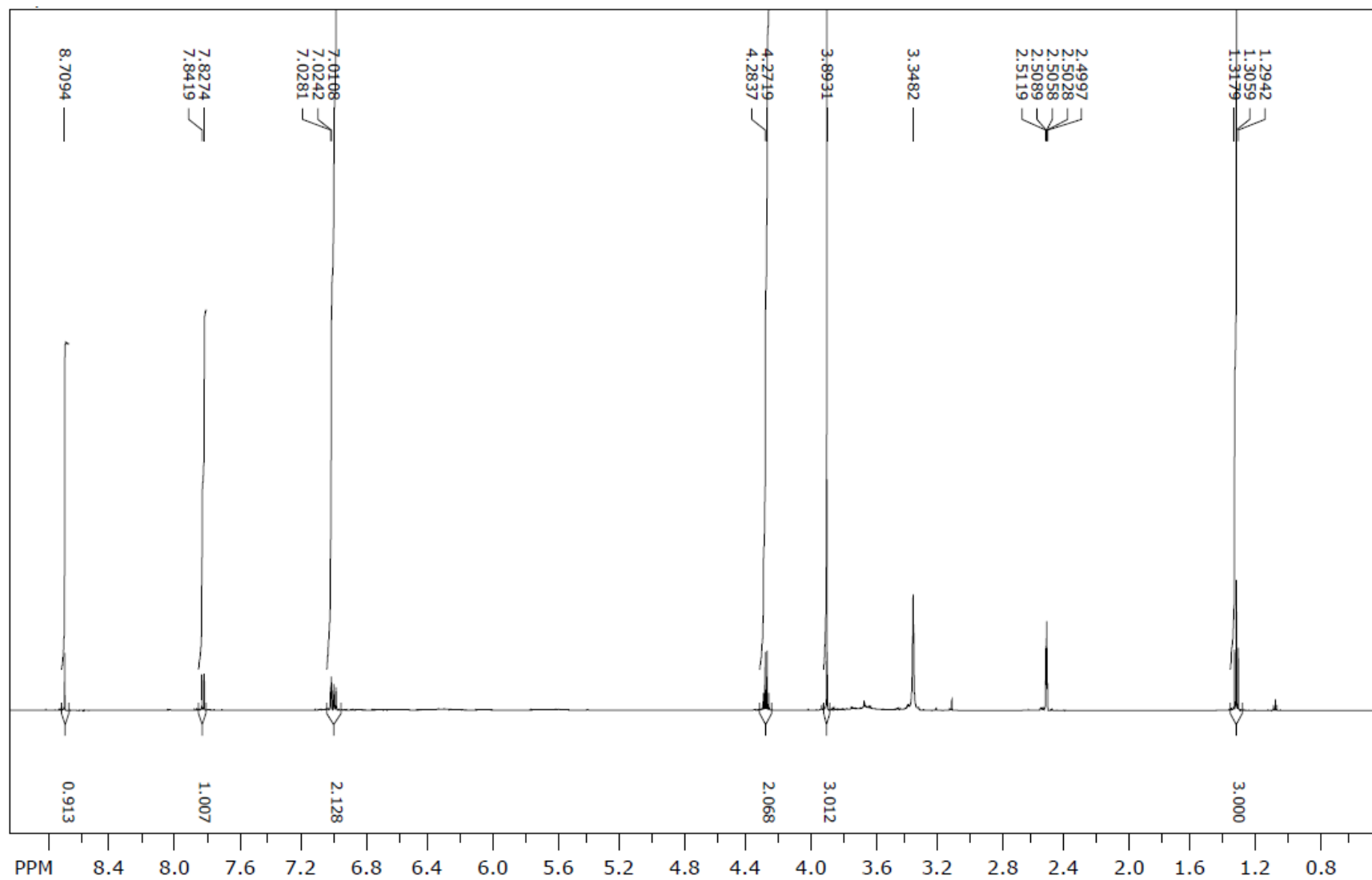
1 H NMR spektr (2d)
