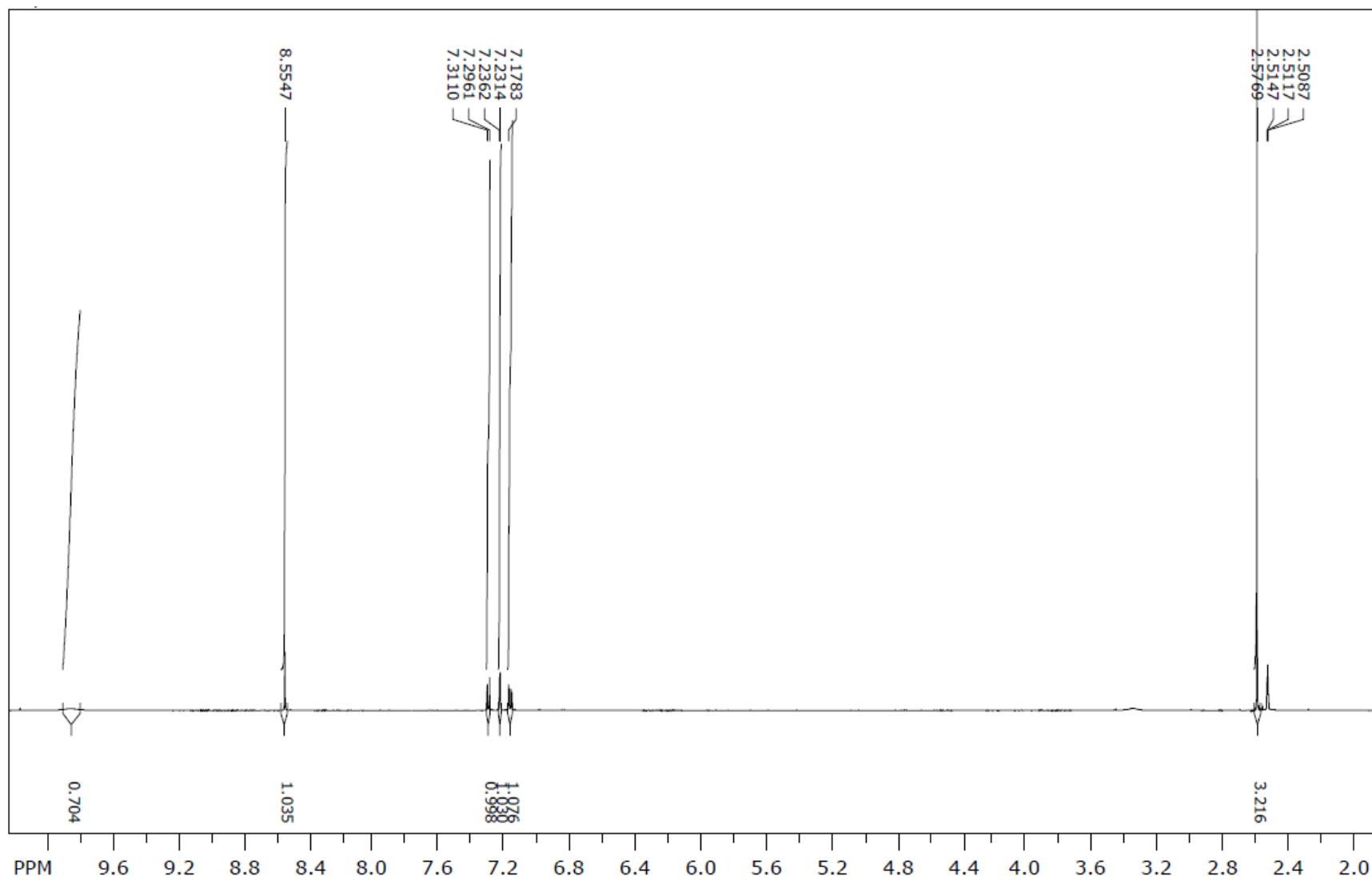
1 H NMR spektr (5c)
