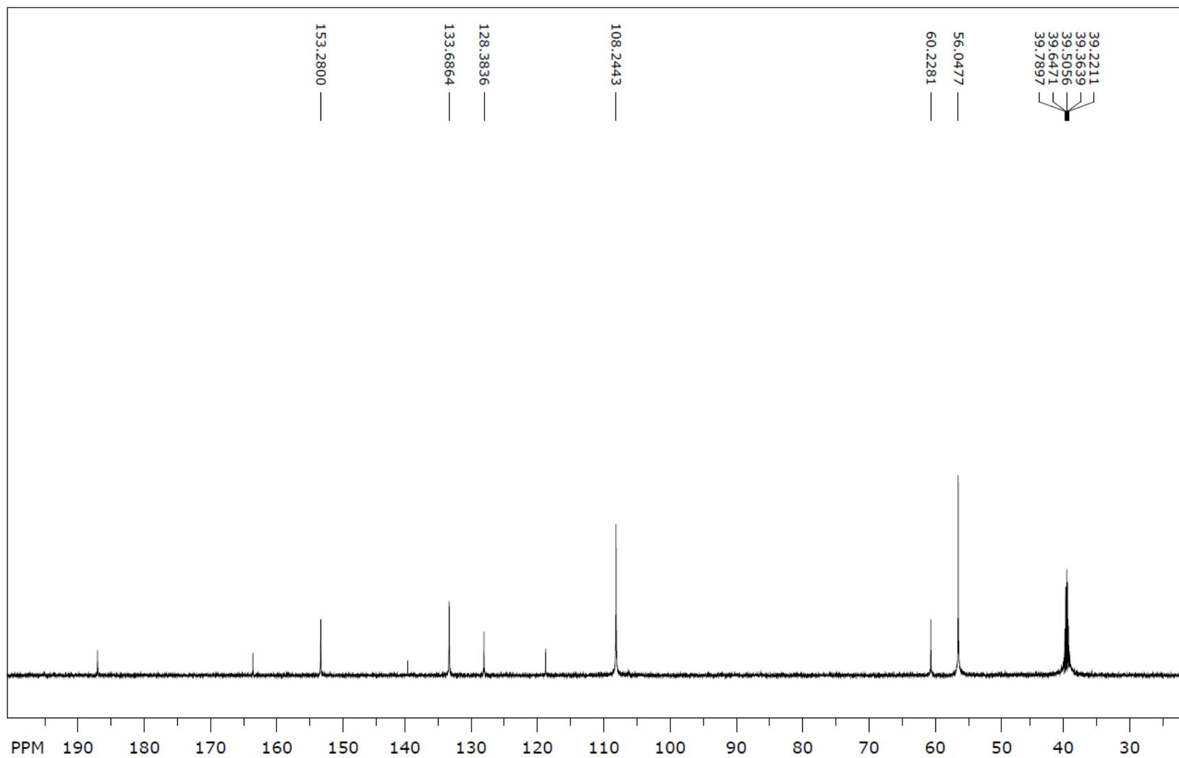
^{13}\text{C} NMR spektr (7i)
