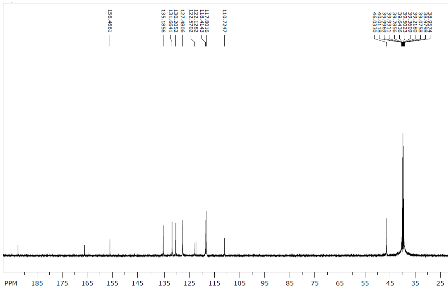
13 C NMR spektr (6b)
