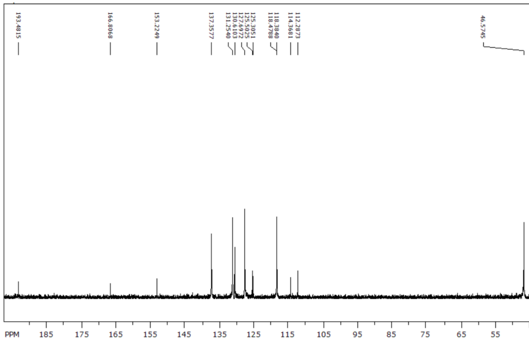
13 C NMR spektr (6l)
