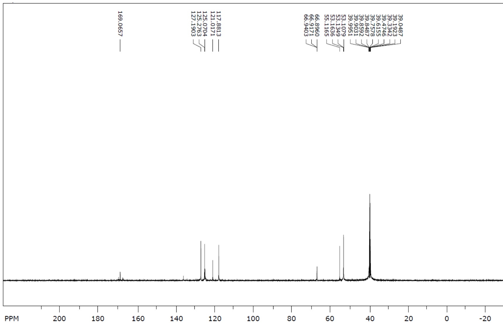
^{13}\text{C} NMR spektr (9j)
