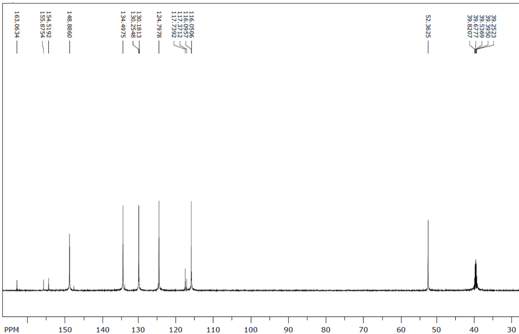
^{13}\text{C} NMR spektr (1a)
