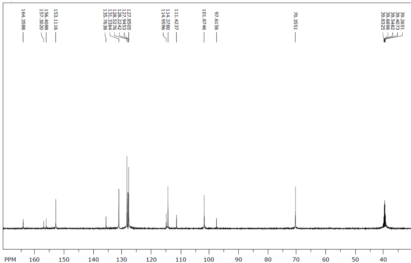
^{13}\text{C} NMR spektr (4b)
