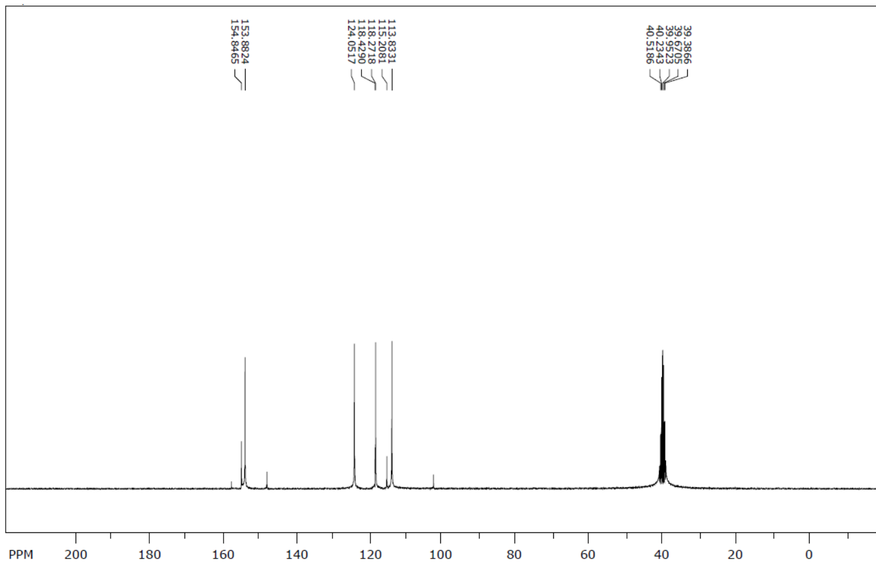
^{13}\text{C} NMR spektr (4e)
