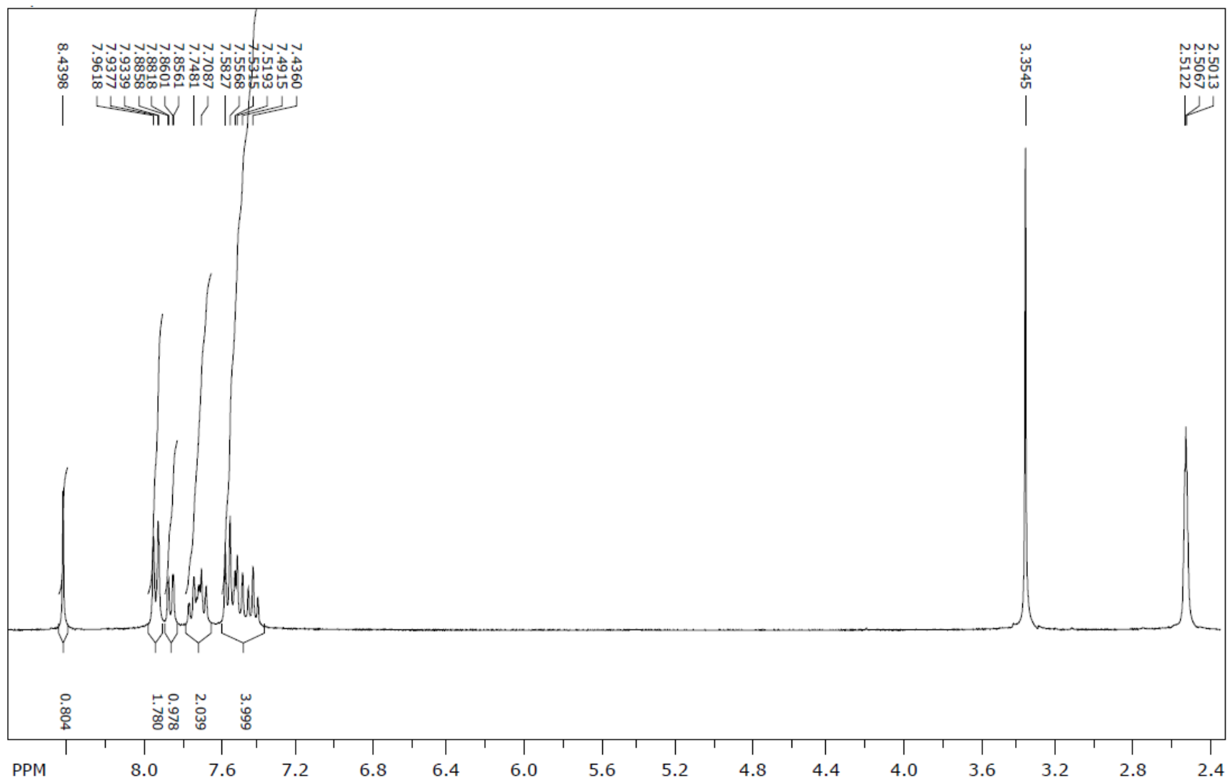
1 H NMR spektr (3a)
