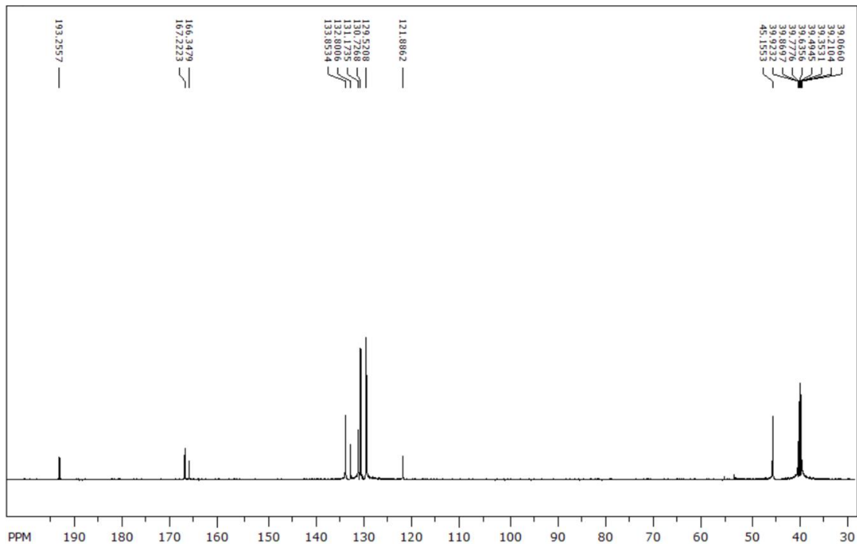
13 C NMR spektar (8o)
