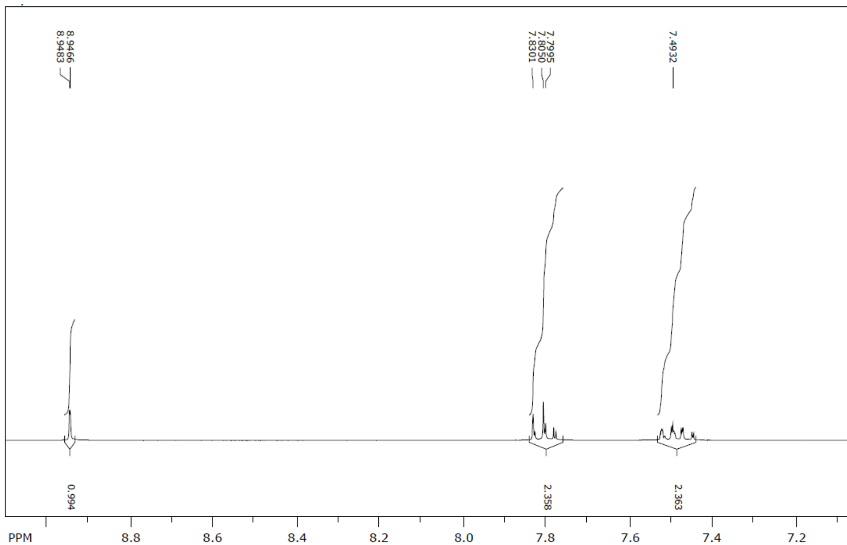
1 H NMR spektr (4a)
