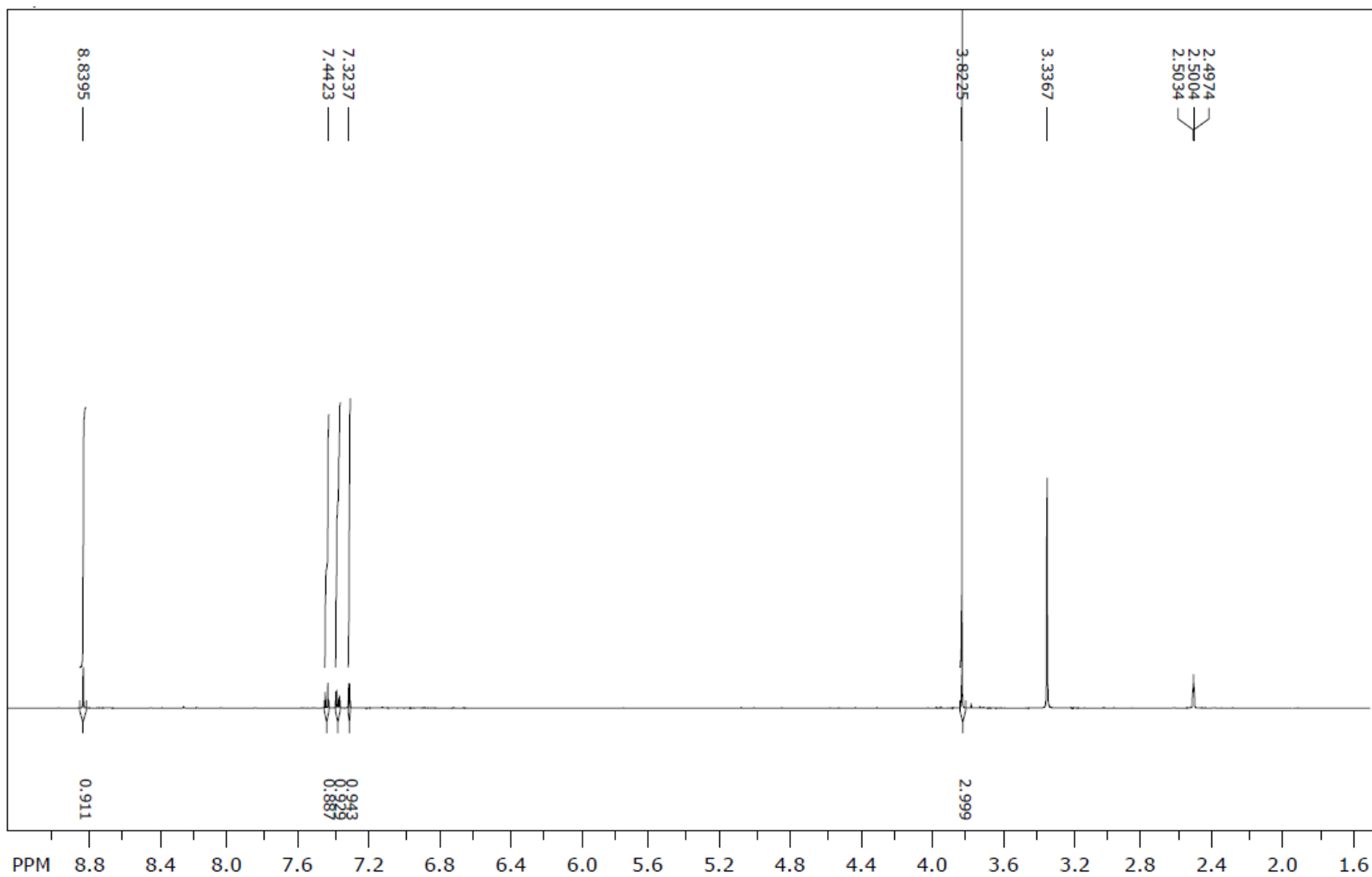
1 H NMR spektr (4f)
