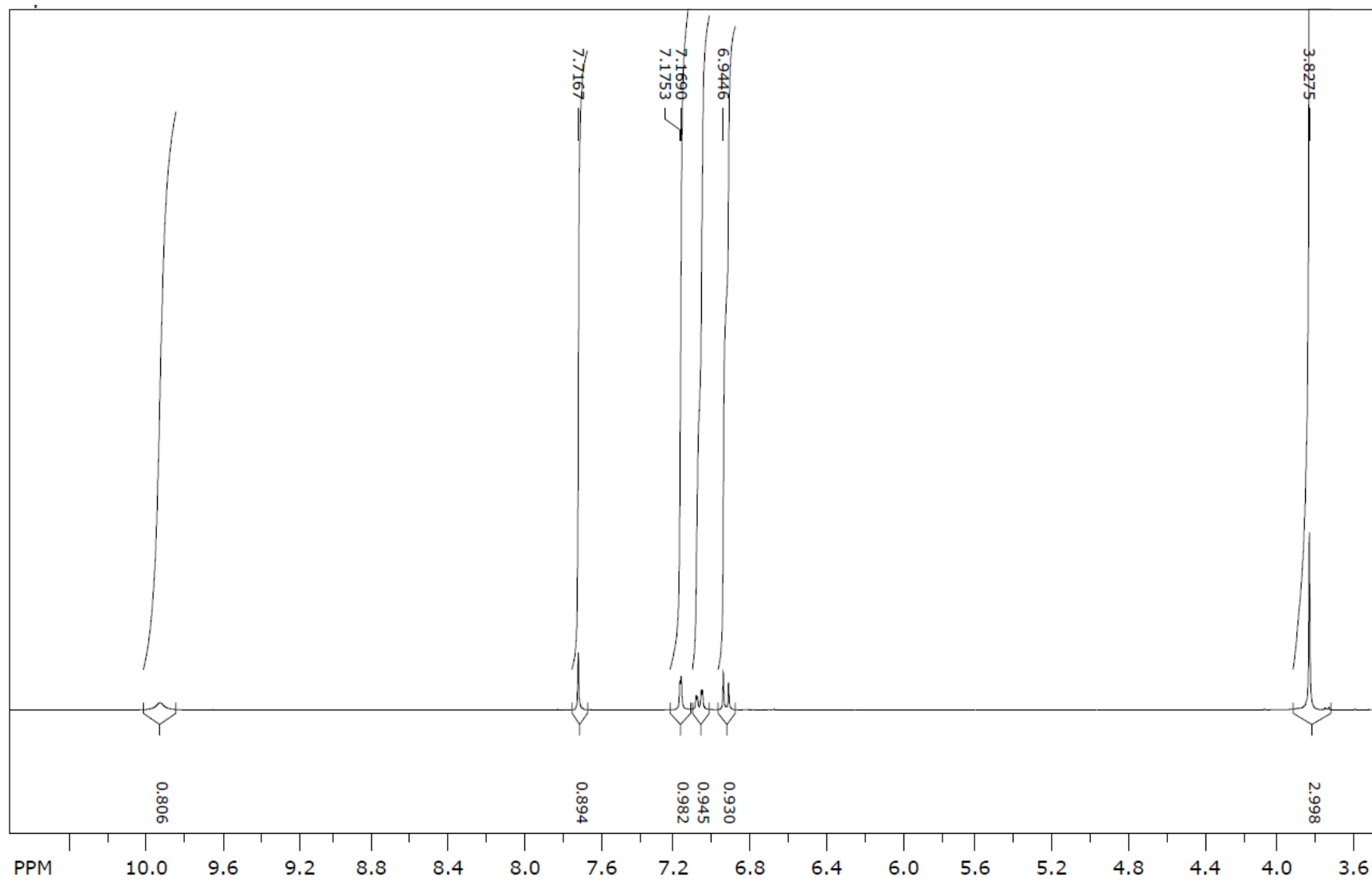
1 H NMR spektr (9b)
