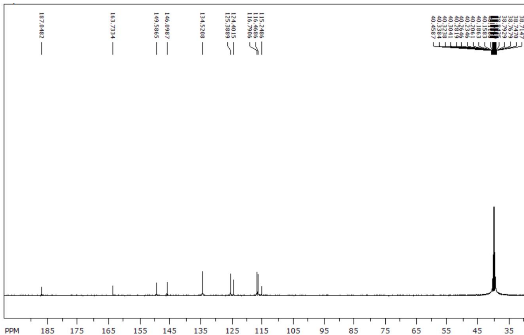
13 C NMR spektar (7h)
