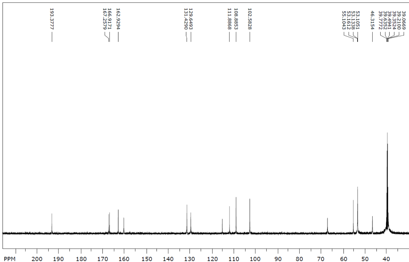
^{13}\text{C} NMR spektr (8a)
