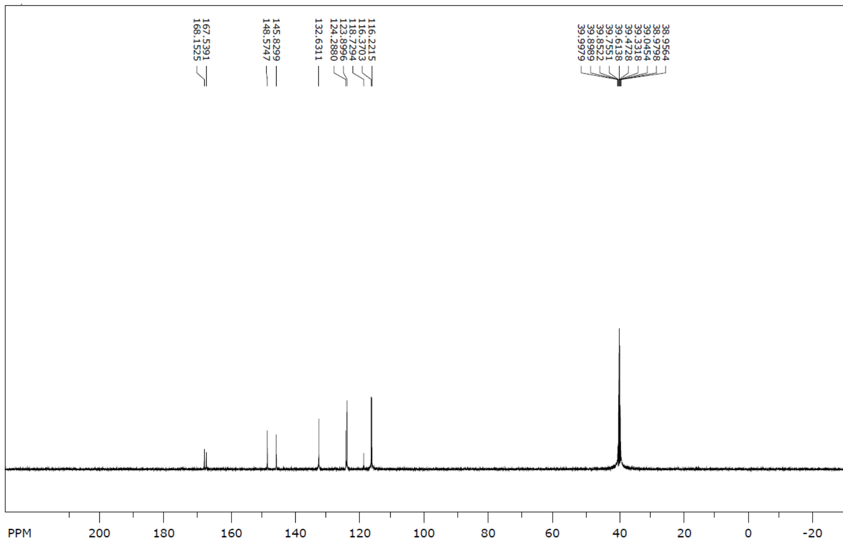
^{13}\text{C} NMR spektr (9f)
