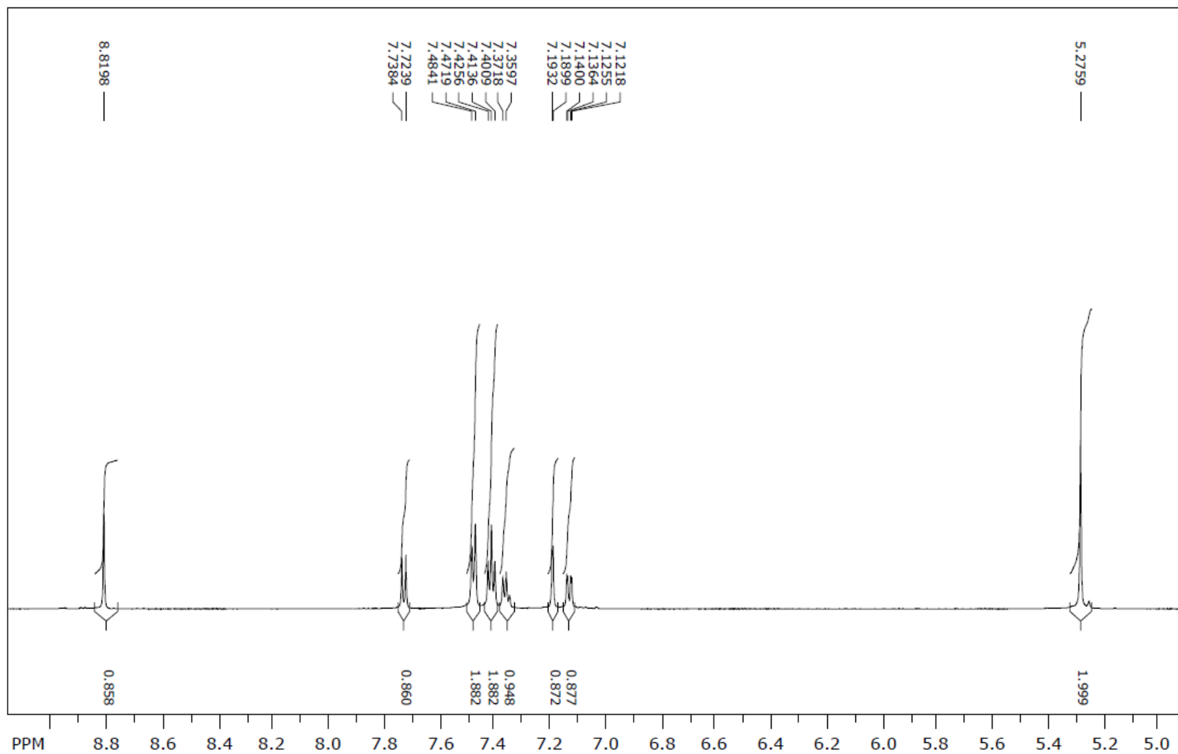
1 H NMR spektar (4b)
