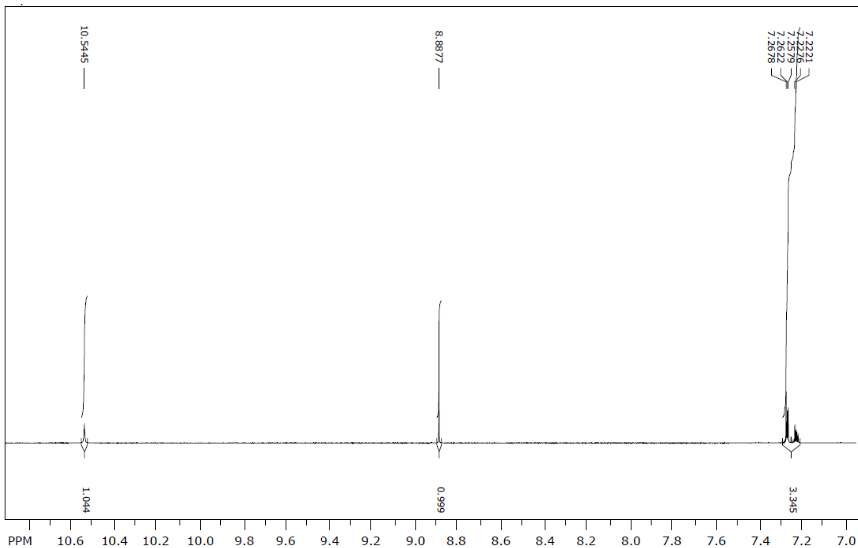
1 H NMR spektr (4c)
