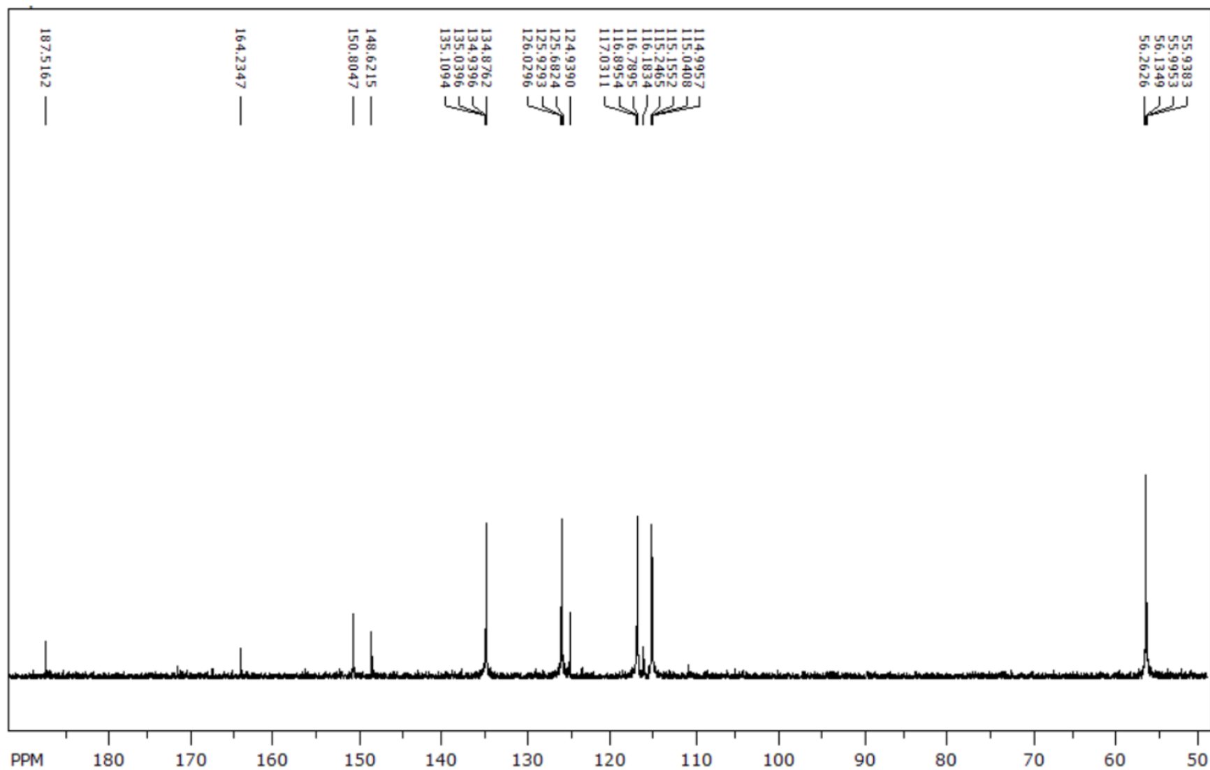
13 C NMR spektr (7a)
