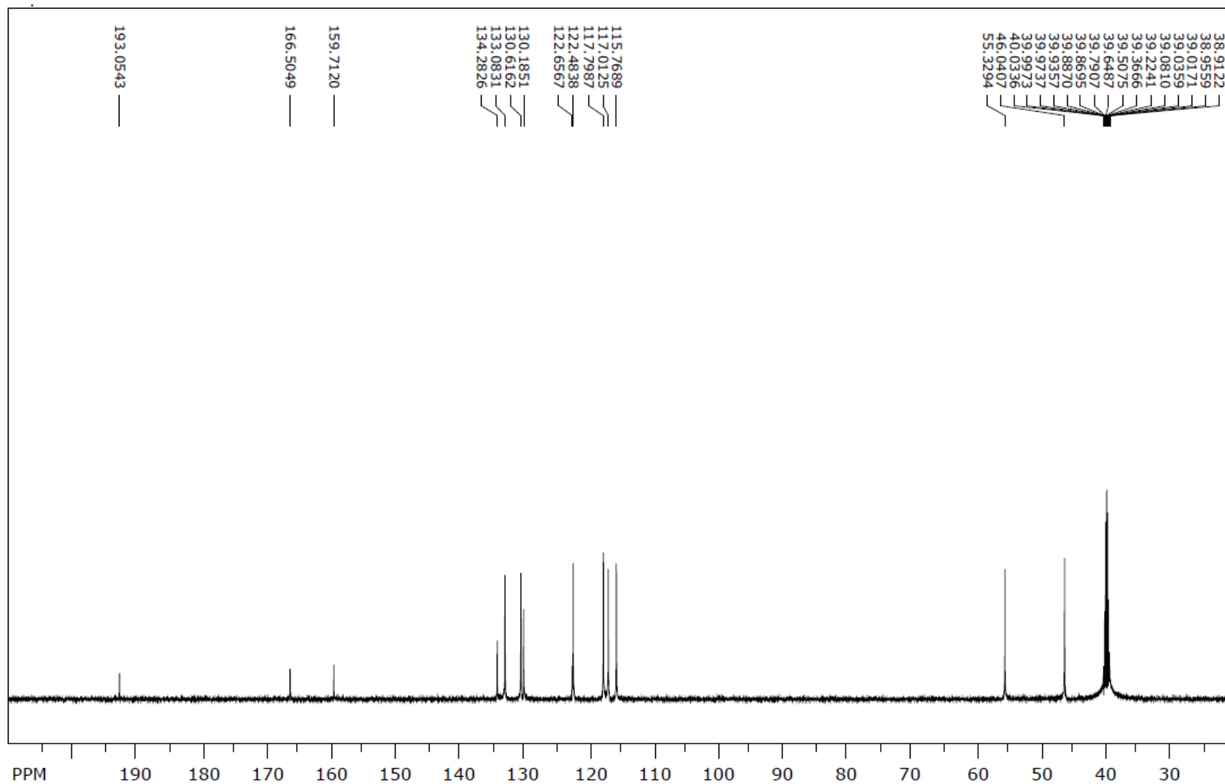
13 C NMR spektr (6f)
