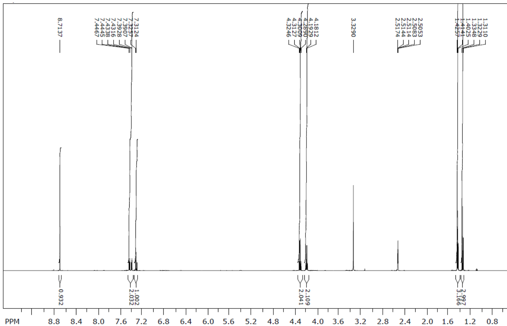
1 H NMR spektr (2e)
