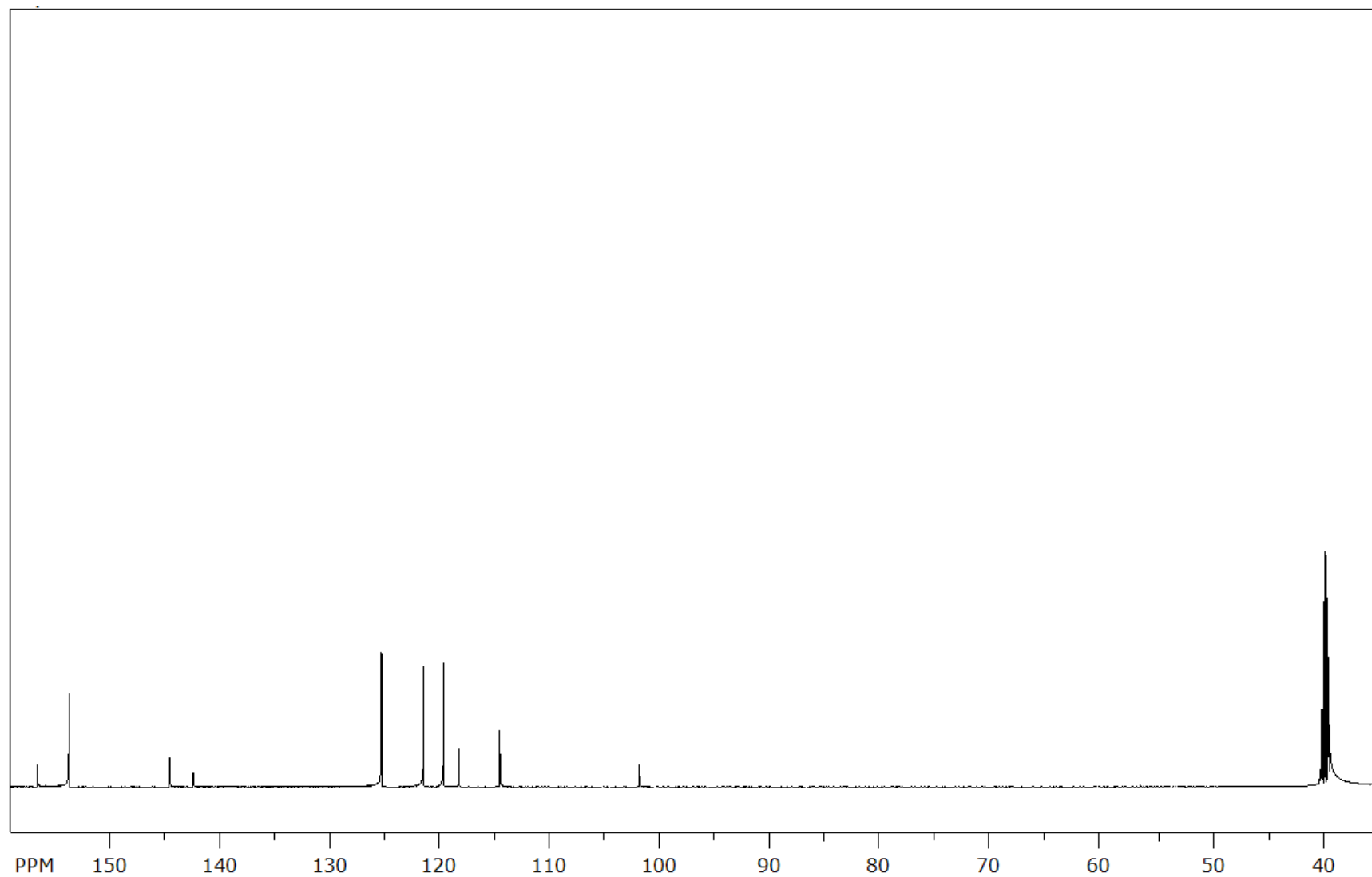
^{13}\text{C} NMR spektr (4c)
