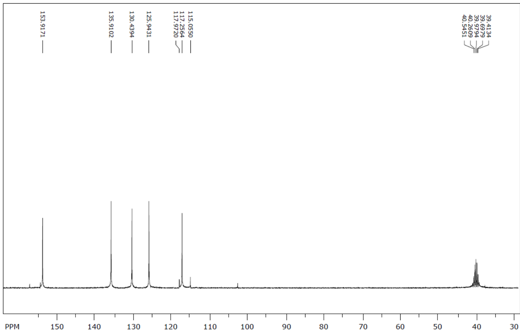
^{13}\text{C} NMR spektr (4a)
