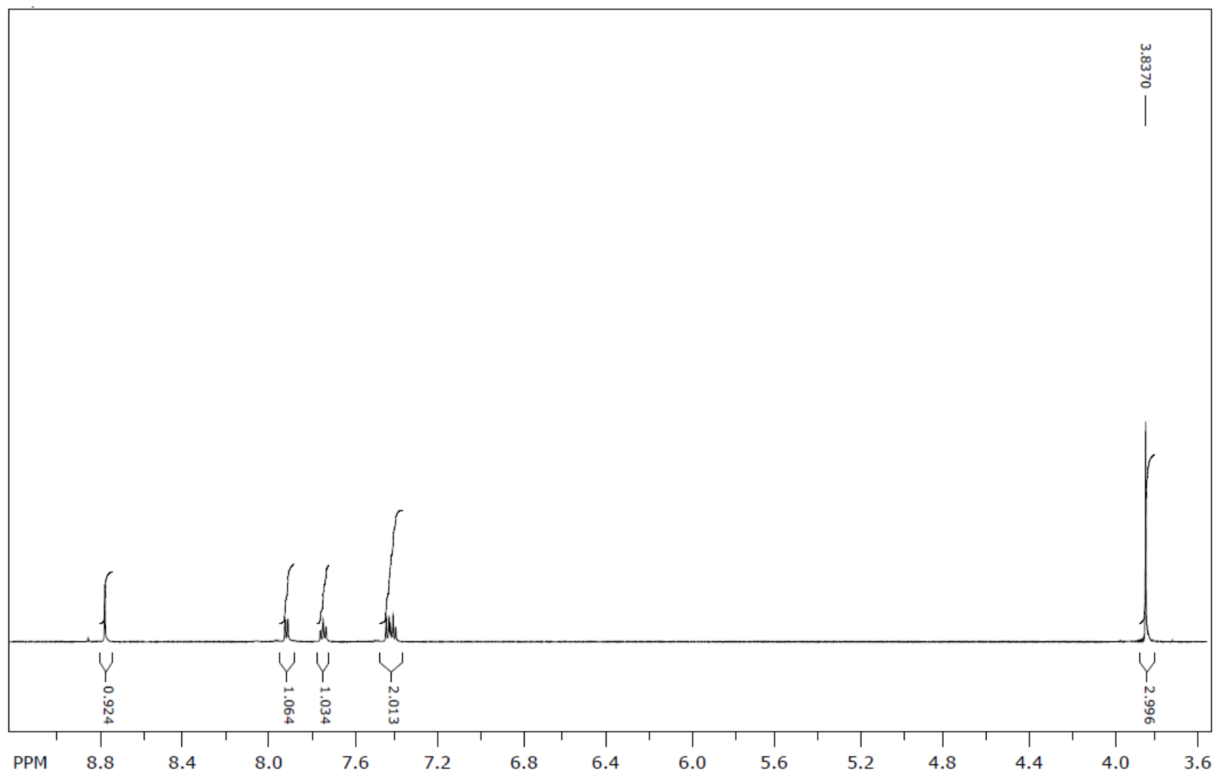
1 H NMR spektr (1a)
