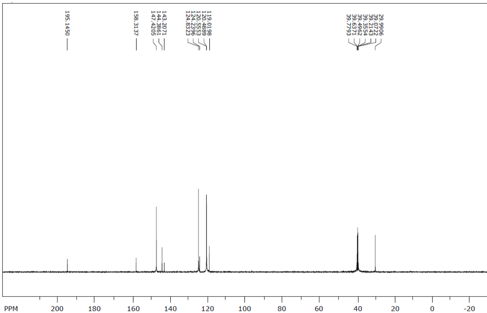
^{13}\text{C} NMR spektr (5a)
