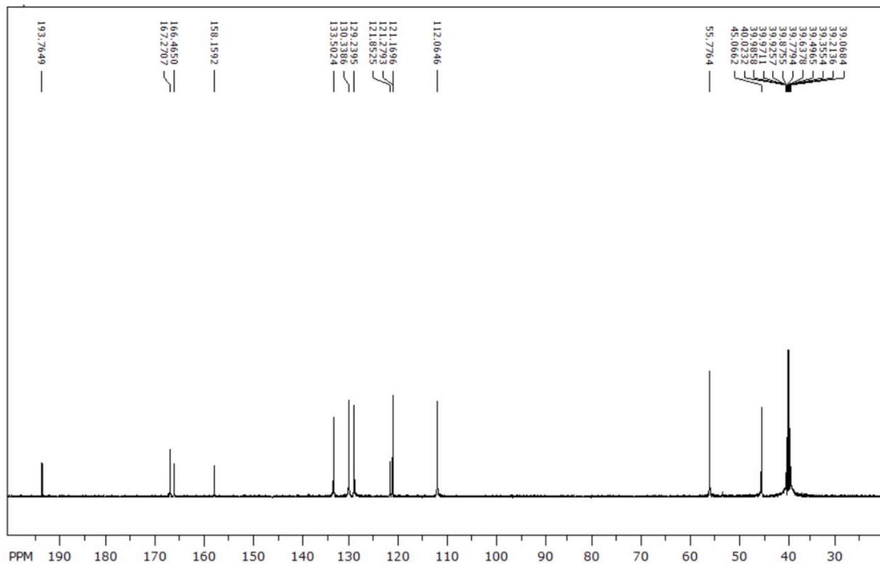
13 C NMR spektar (8j)
