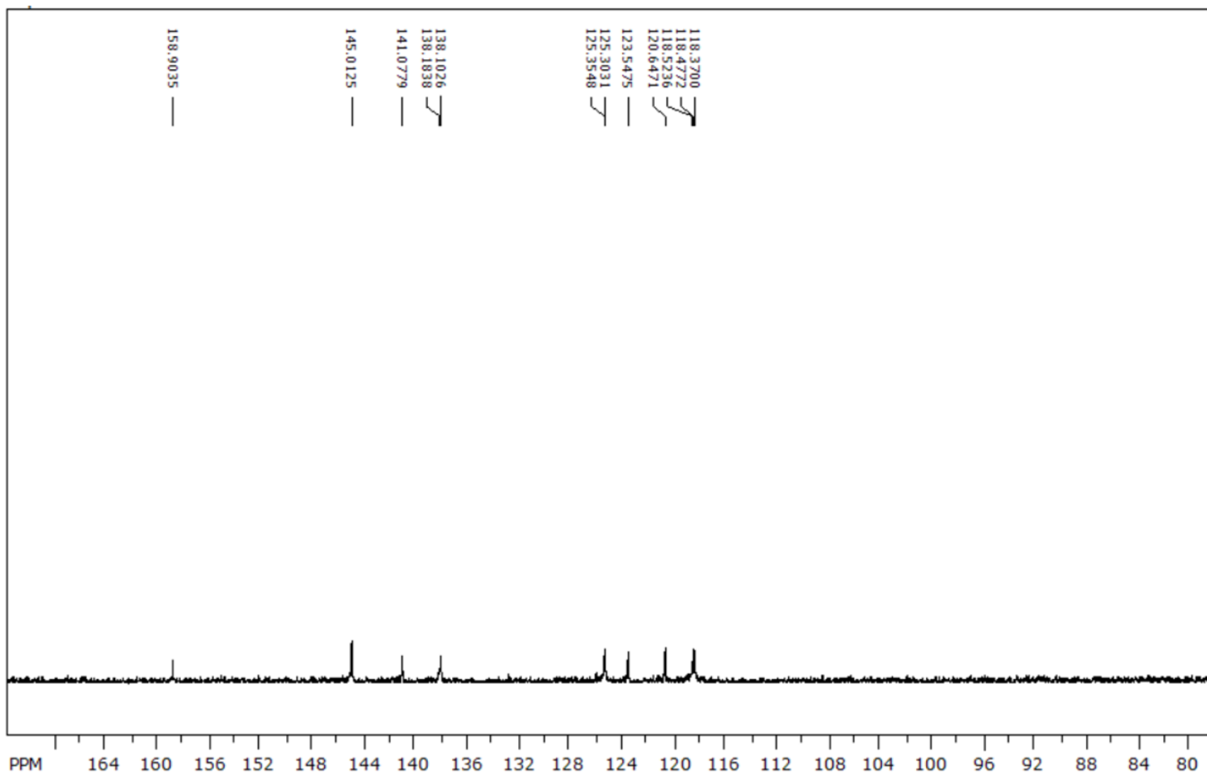
13 C NMR spektr (7b)
