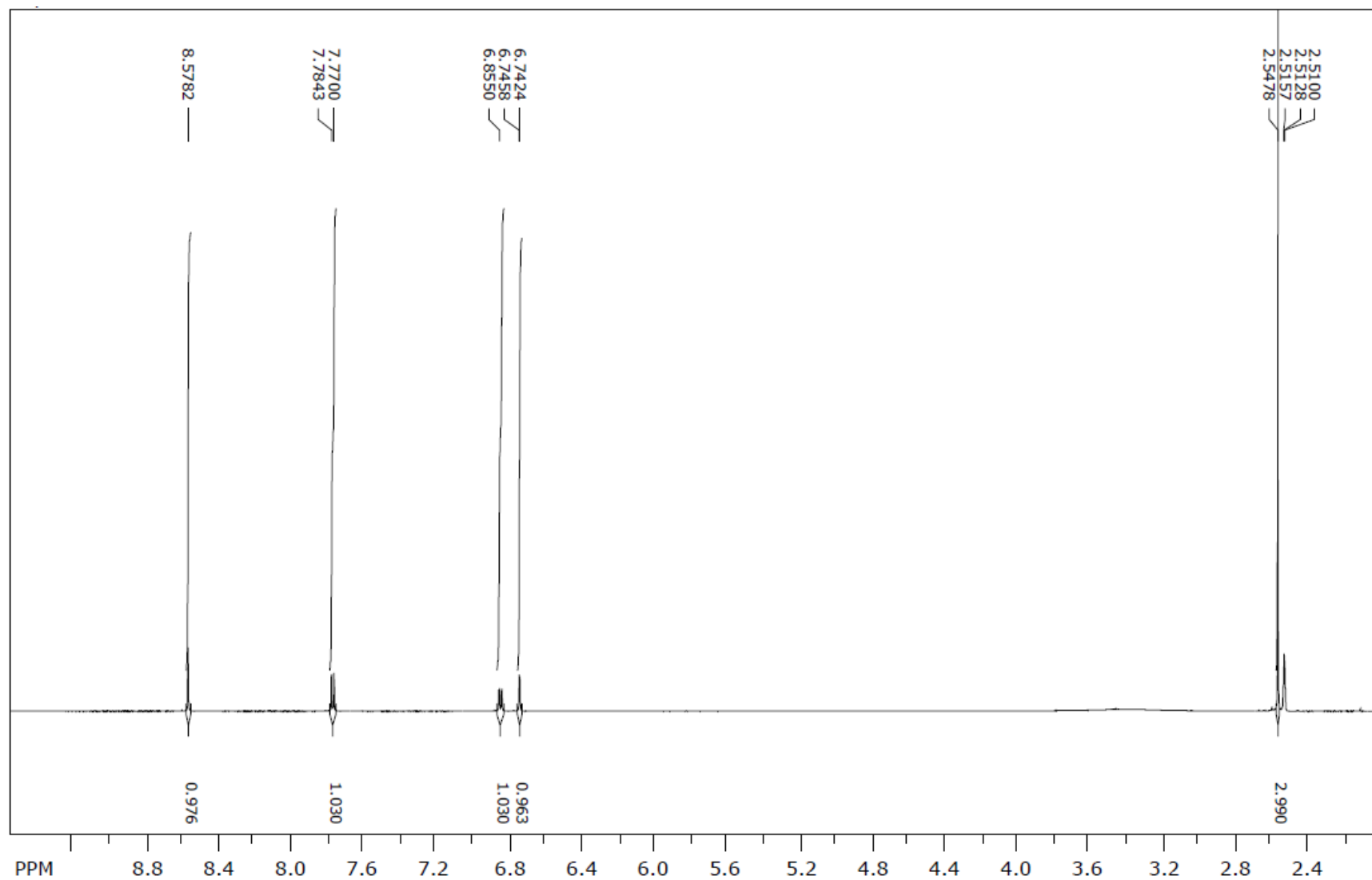
1 H NMR spektr (5b)
