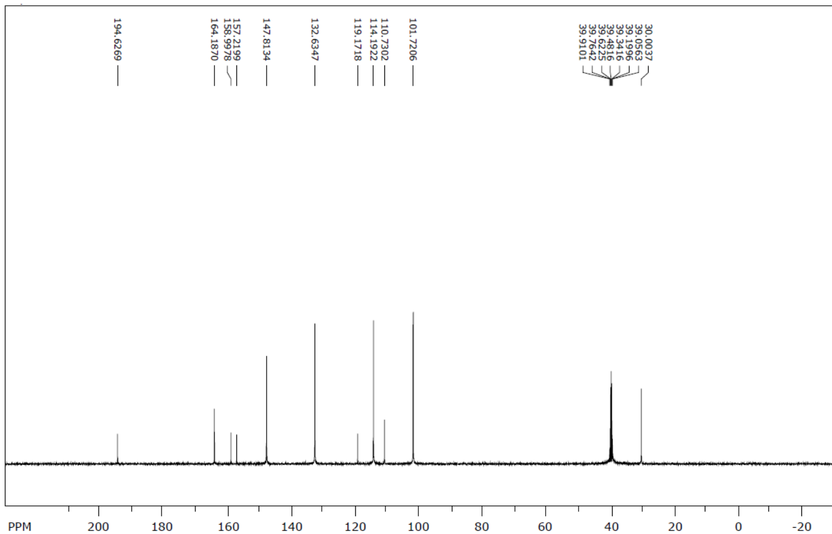
^{13}\text{C} NMR spektr (5b)
