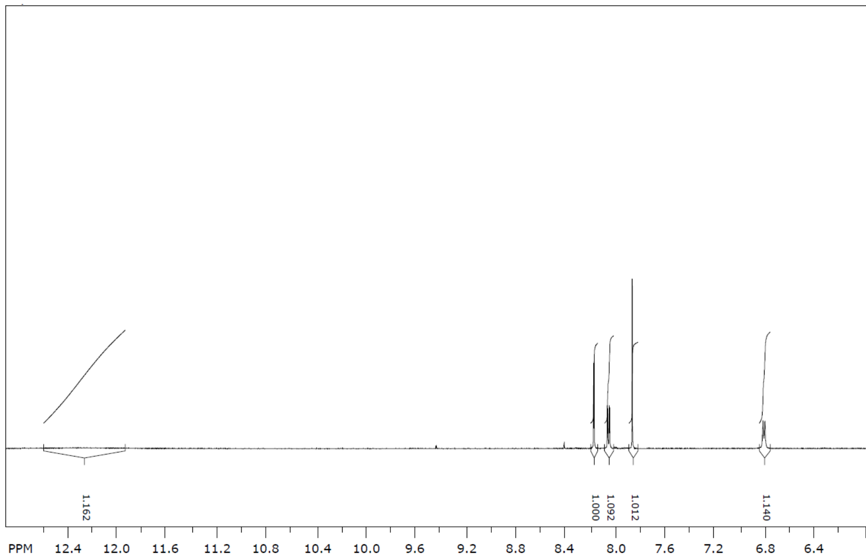
1 H NMR spektr (9j)
