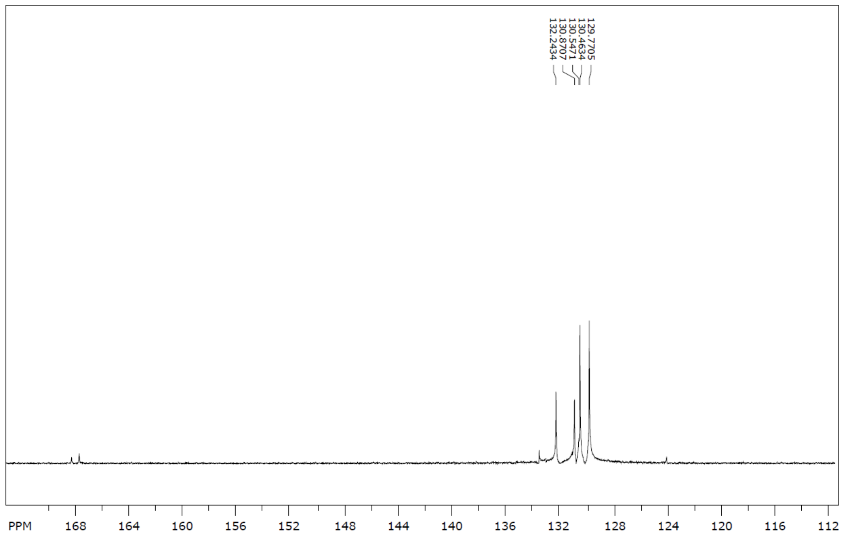
^{13}\text{C} NMR spektr (9r)
