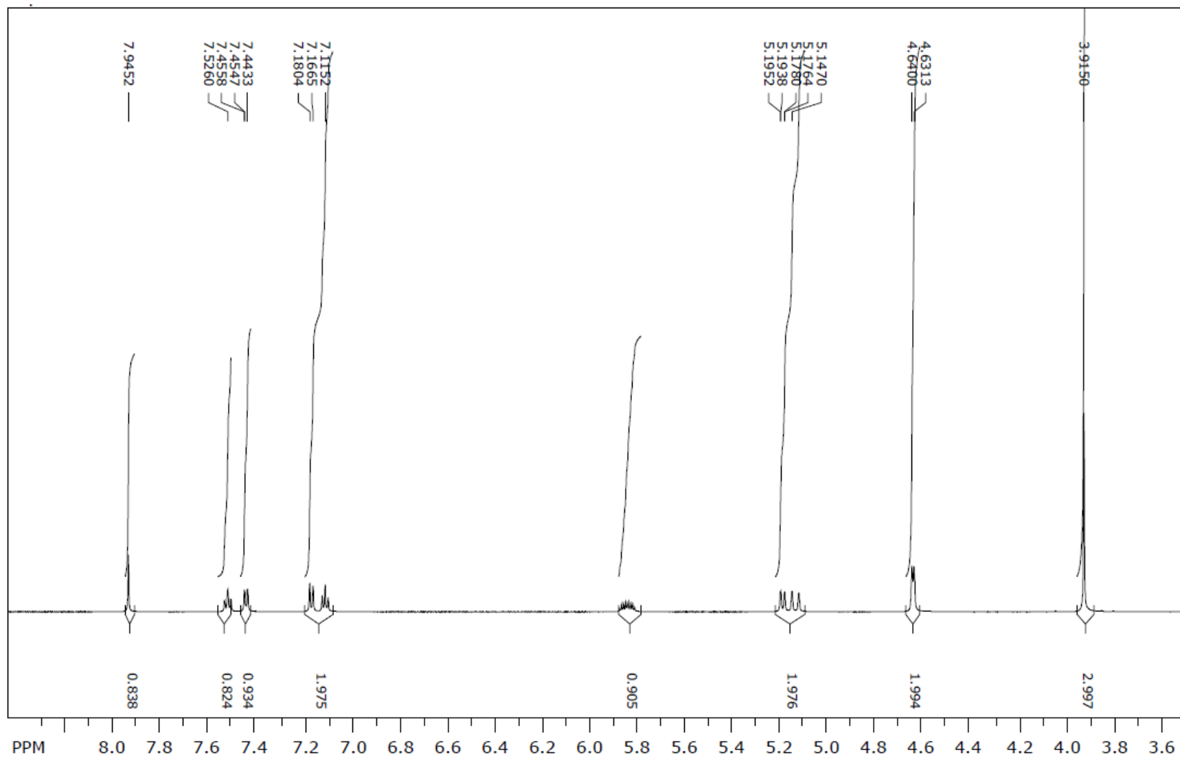
1 H NMR spektr (6o)
