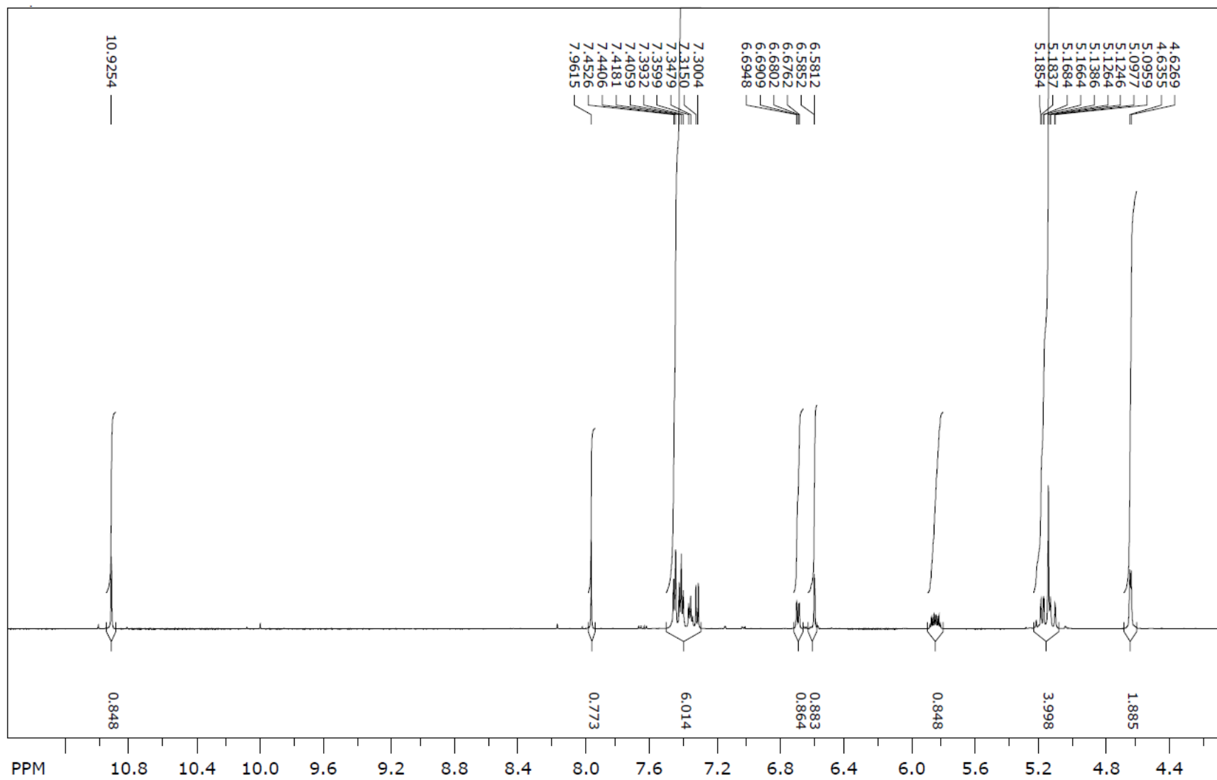
1 H NMR spektr (6t)
