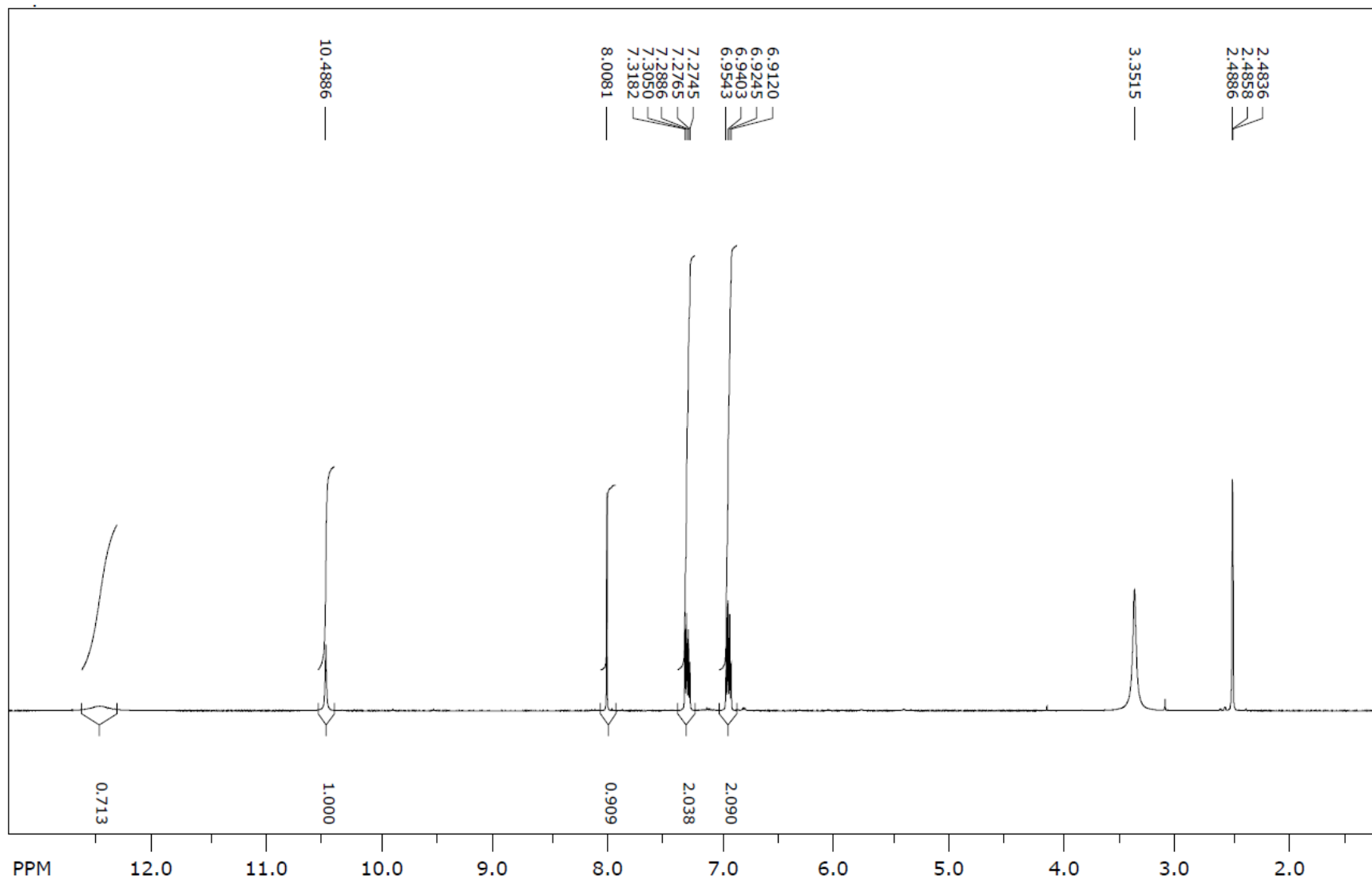
1 H NMR spektr (9a)
