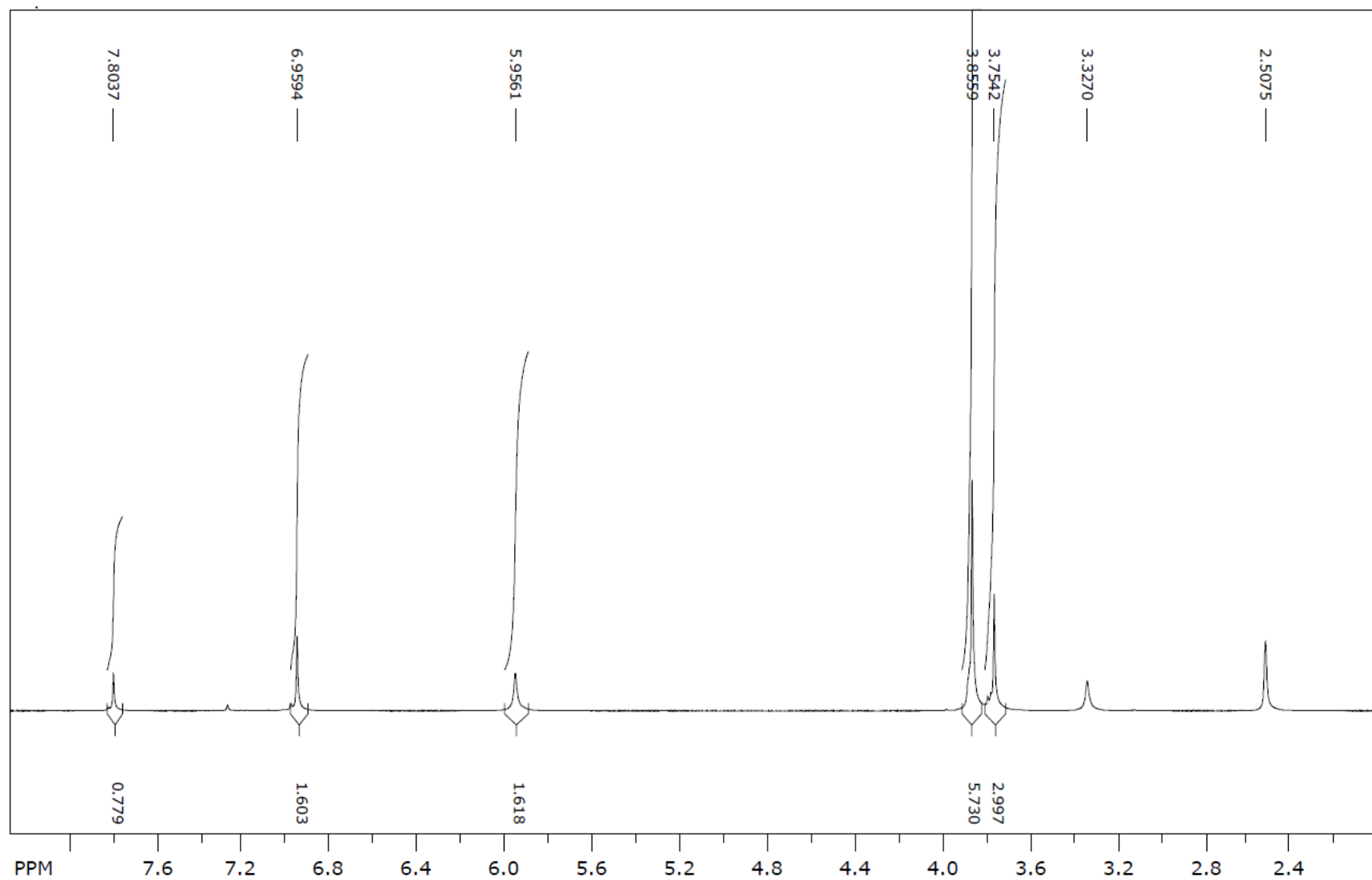
1 H NMR spektr (7i)
