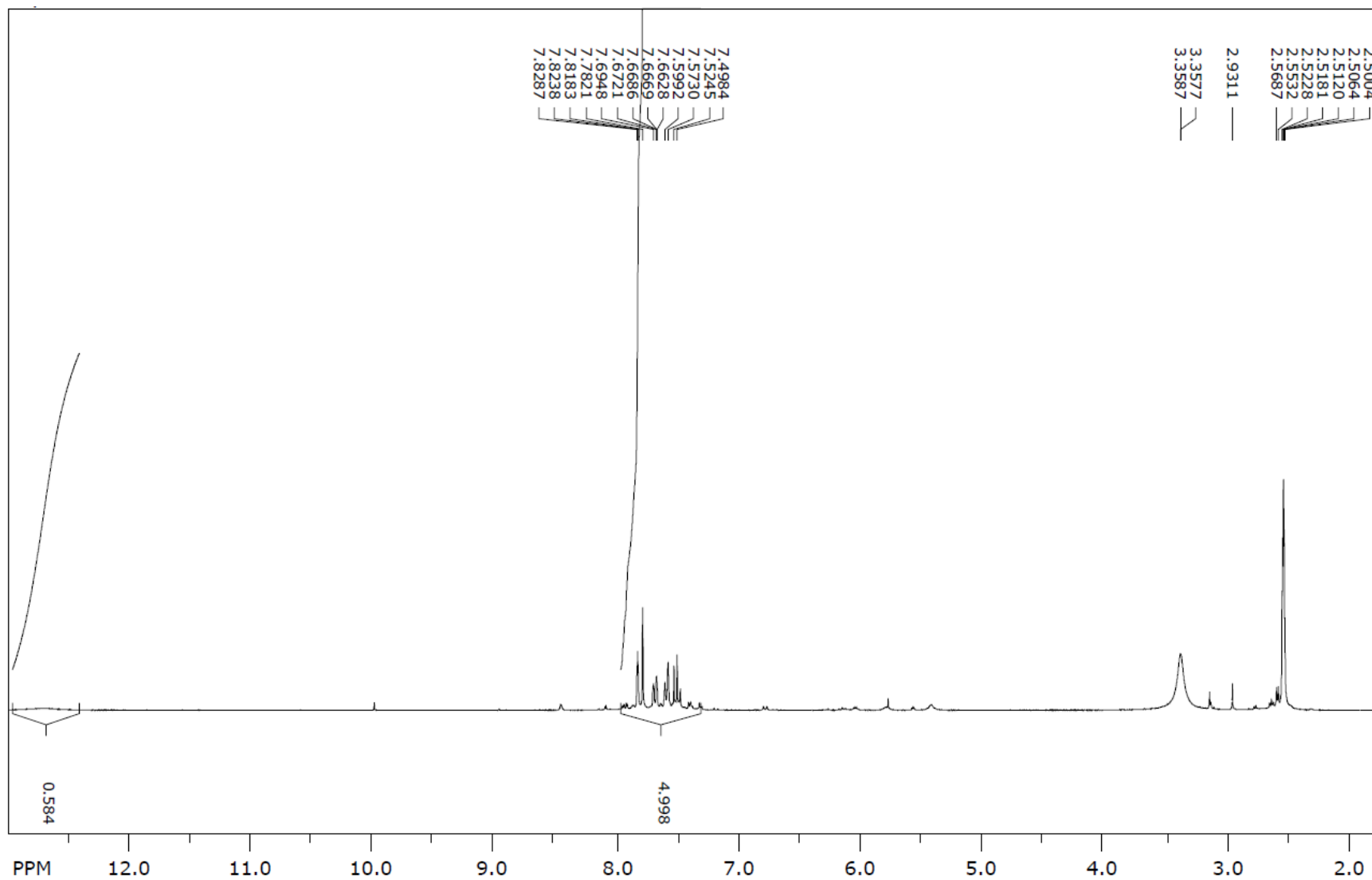
1 H NMR spektr (9i)
