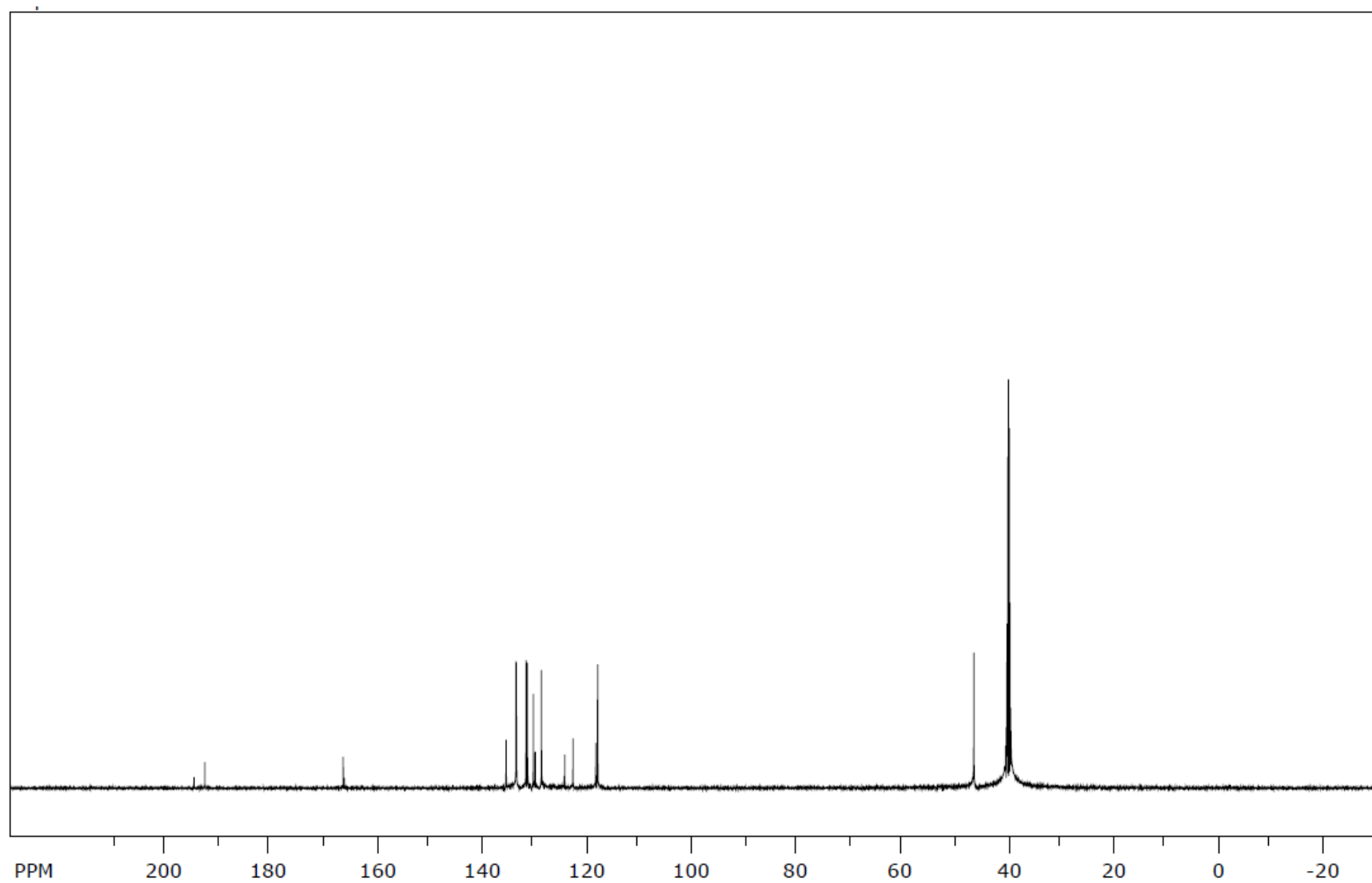
^{13}\text{C} NMR spektr (6j)
