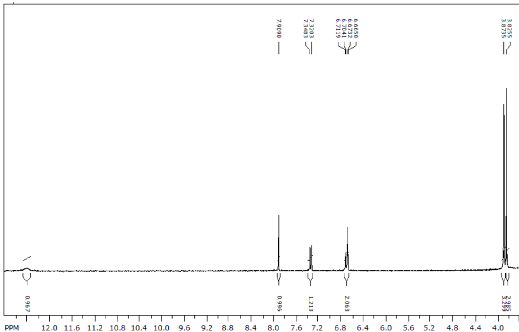
1 H NMR spektr (9q)
