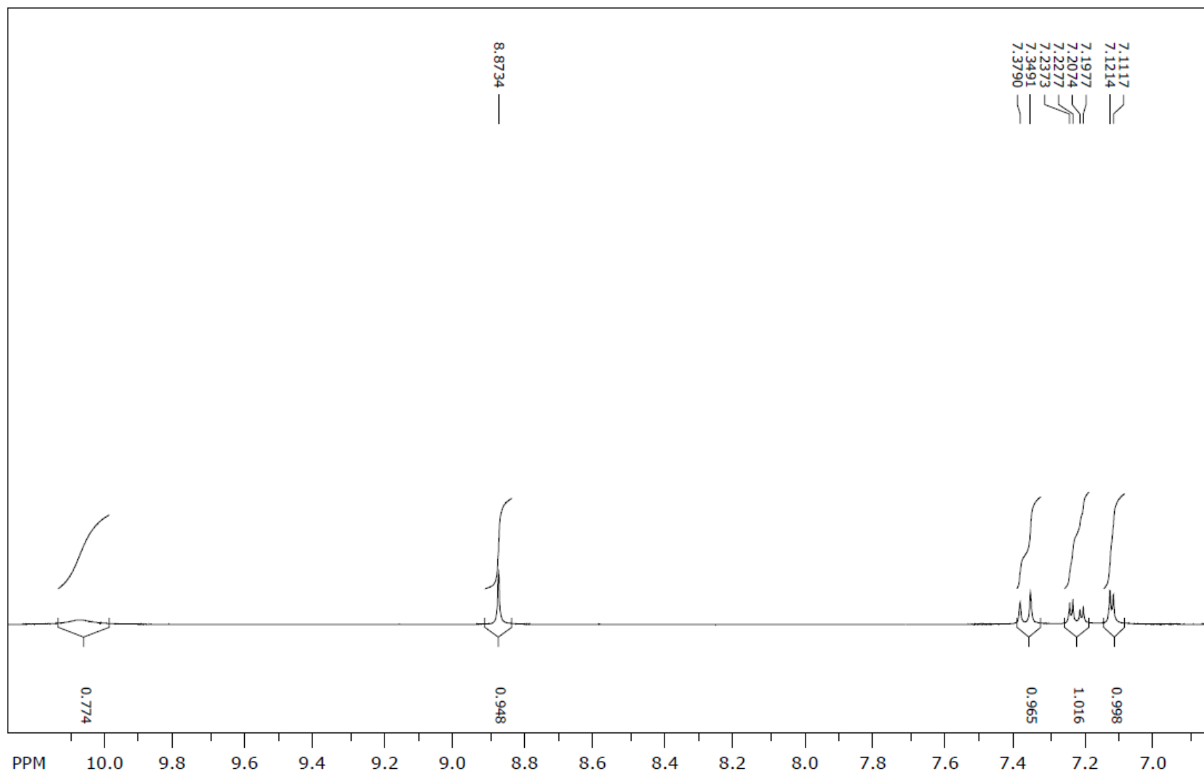
1 H NMR spektr (4e)
