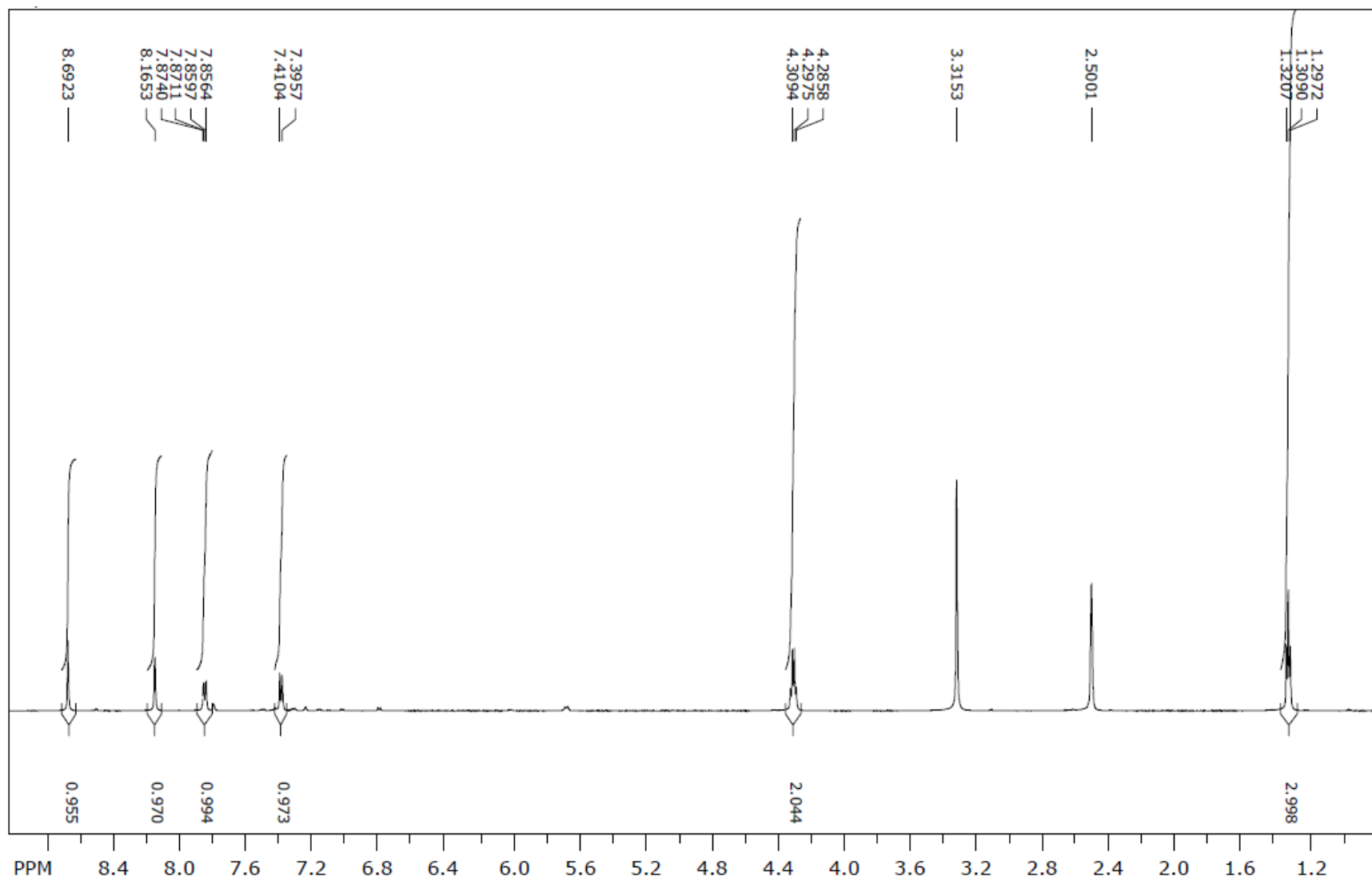
1 H NMR spektr (2b)
