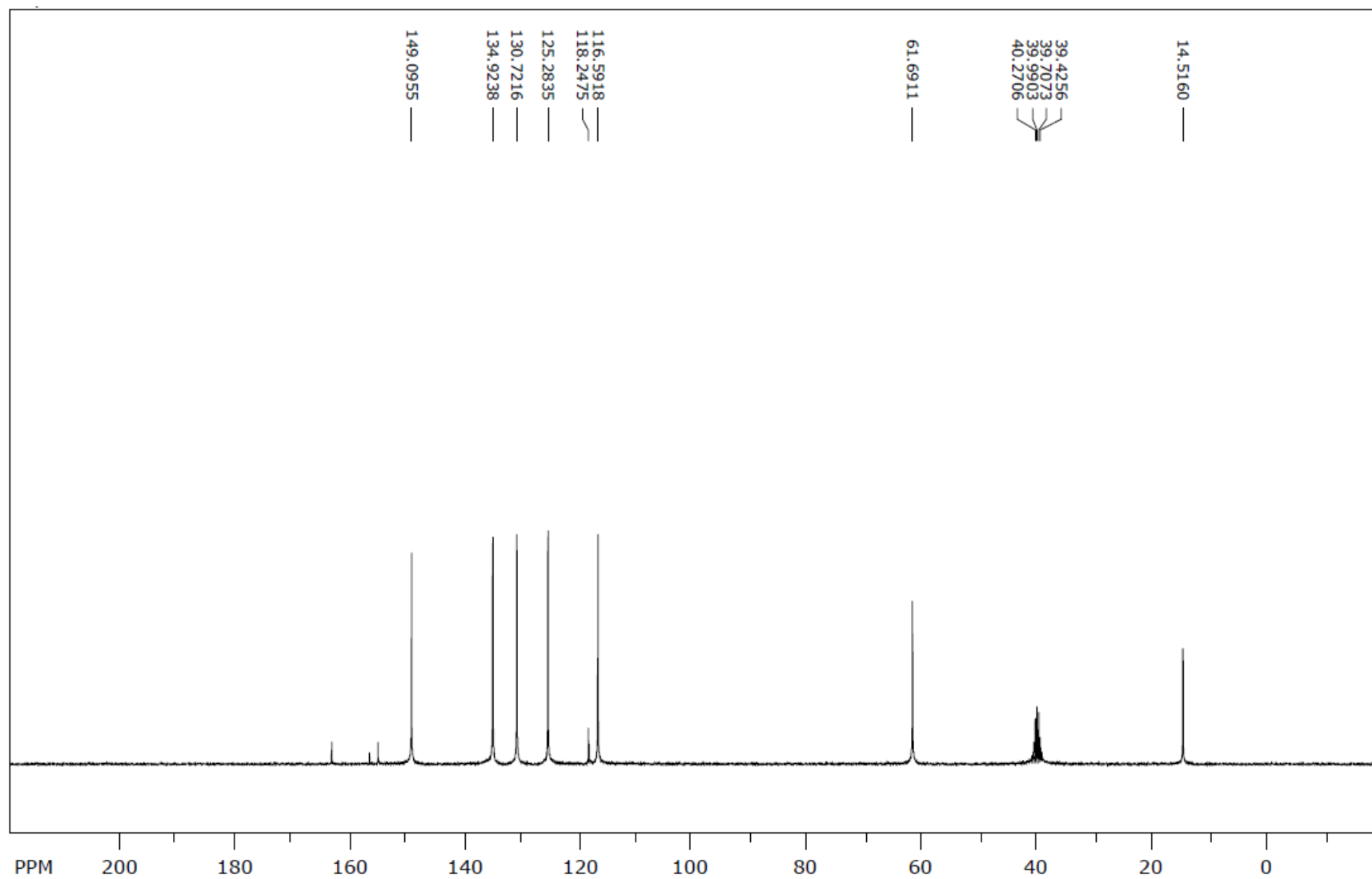
^{13}\text{C} NMR spektr (2a)
