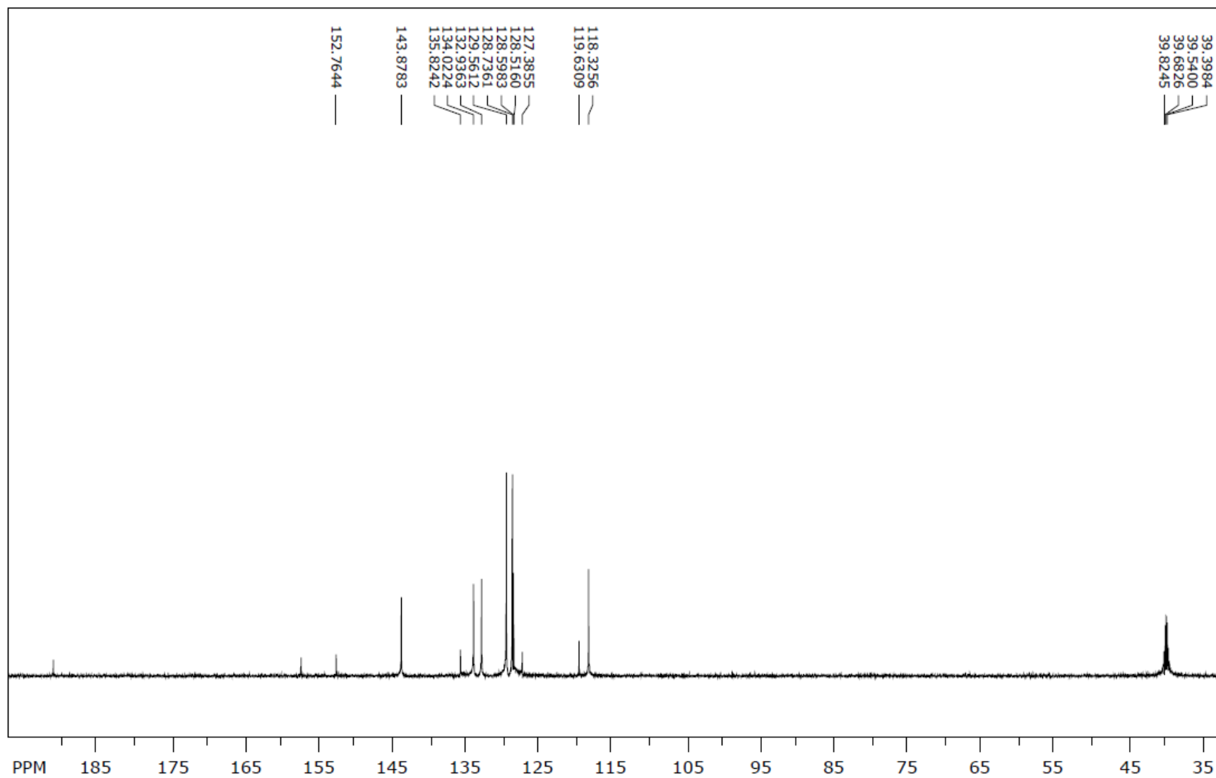
13 C NMR spektr (3f)
