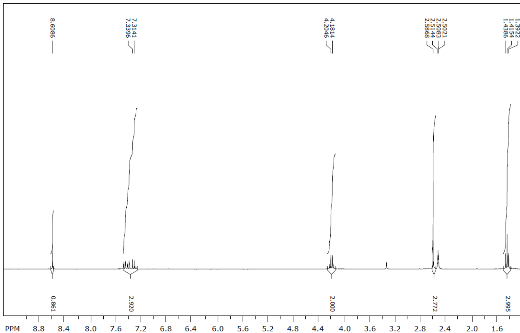
1 H NMR spektr (5f)
