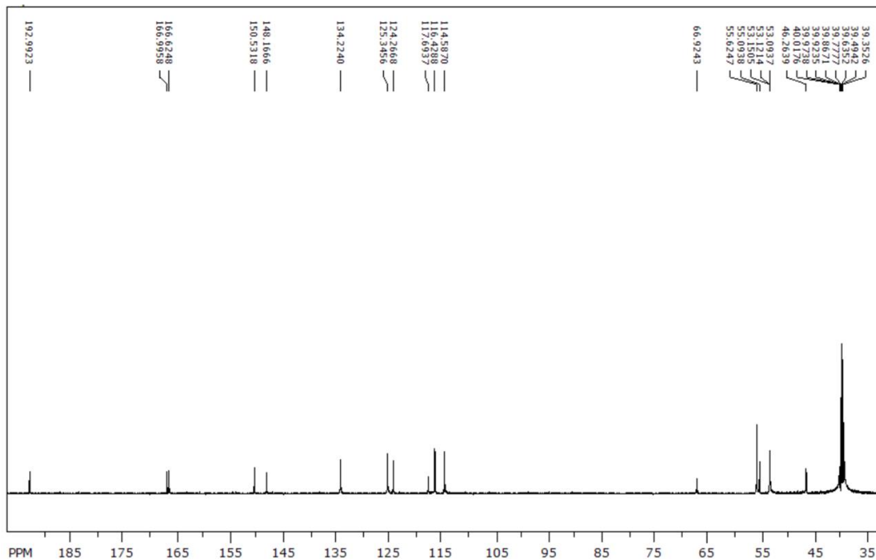
13 C NMR spektr (8b)
