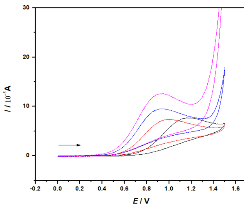
Slika 27 Ciklički voltamogrami vitamina C koncentracije 10 -3 M (pH=2—, pH=4 —, pH=6 — i pH=8 —) dobiveni uz eksperimentalne uvjete iz Tablice 4
