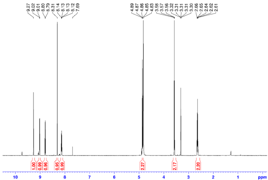
Slika 15 1 H NMR spektar spoja 1
