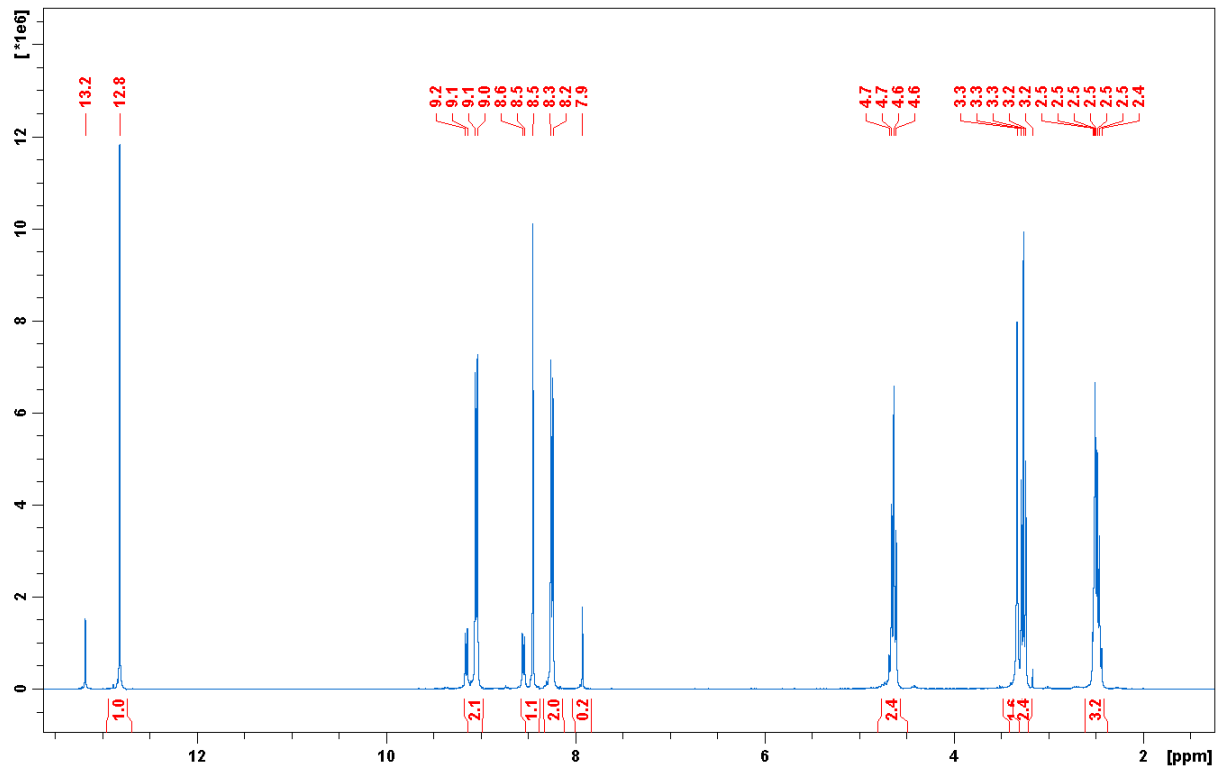
Slika 28 ^1\text{H} NMR spektar spoja 6
