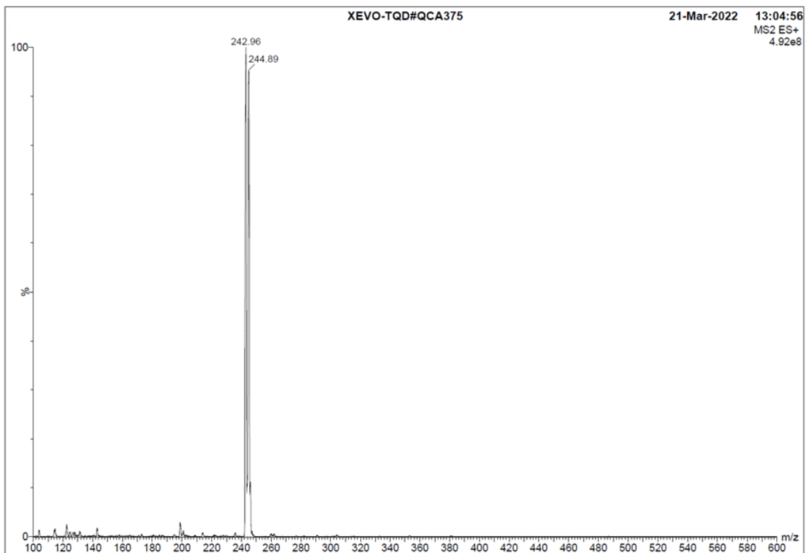
Slika 17 Maseni spektar spoja 1
