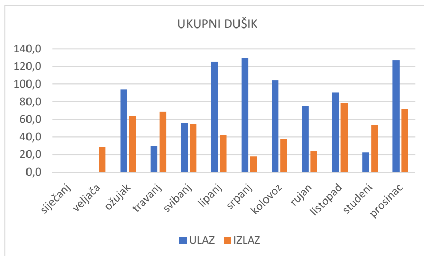
Slika 44 Mjesečne vrijednosti koncentracije ukupnog dušika (mg N/L) u ulaznoj otpadnoj vodi i izlaznoj pročišćenju na UPOV Podravske Sesvete tijekom 2022. godine
