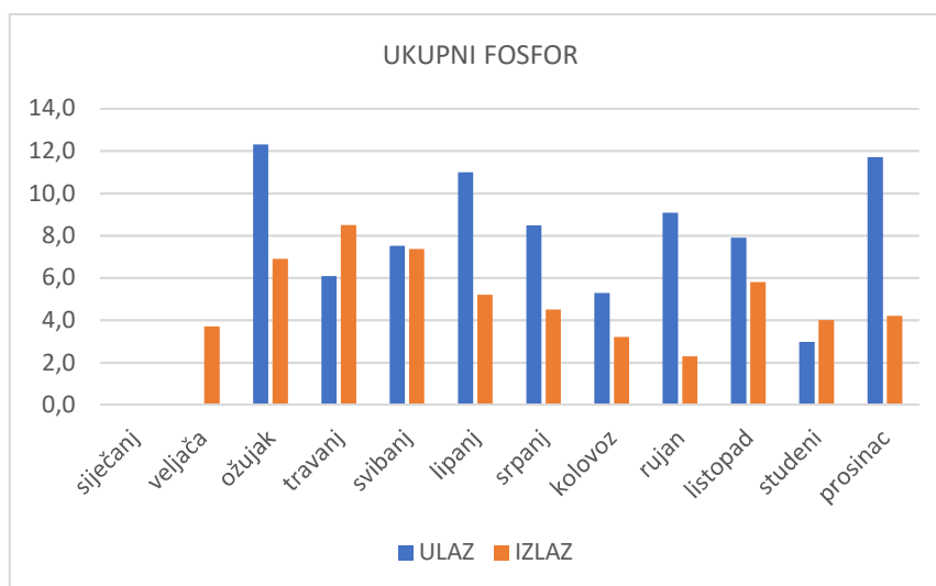
Slika 45 Mjesečne vrijednosti koncentracije ukupnog fosfora (mg P/L) u ulaznoj otpadnoj vodi i izlaznoj pročišćenju na UPOV Podravske Sesvete tijekom 2022. godine
