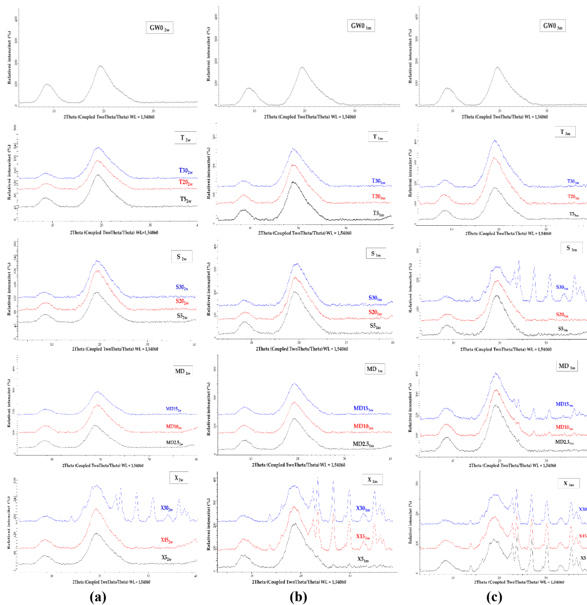
Slika 42 XRPD difraktogrami za sve MC nakon ubranog starenja tijekom: (a) 2 tjedna, (b) 1 mjeseca i (c) 3 mjeseca.
