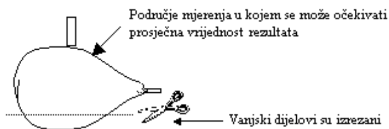
Slika 13 Prikaz mjerenja čvrstoće tj. teksture ploda kruške
