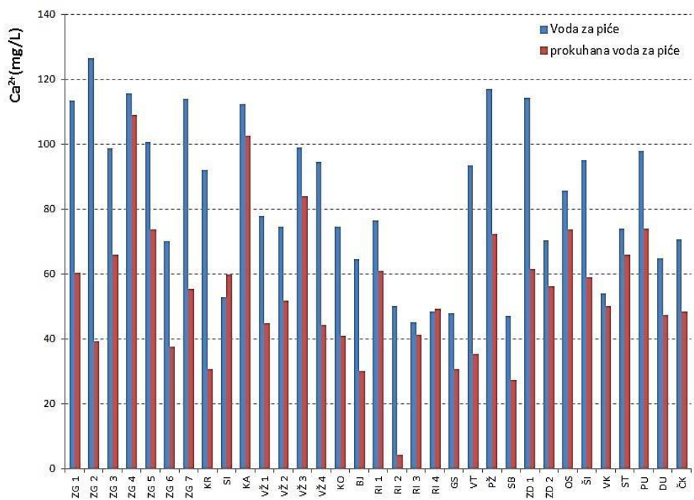
Slika 9 Grafički prikaz rezultata analize uzoraka vode za ljudsku potrošnju za kalcij
