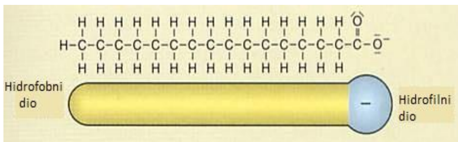
Slika 4. Molekula emulgatora
