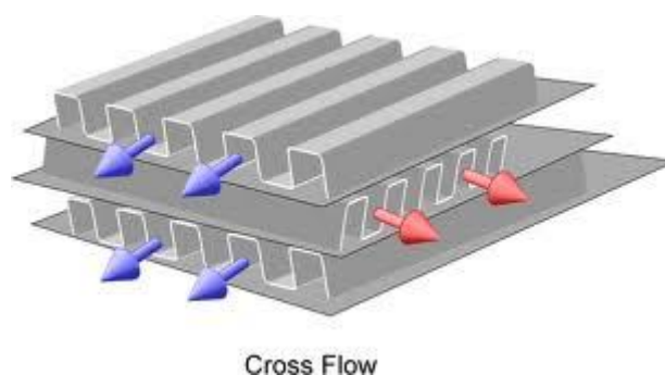
Slika 5 Unakrsni tok kod izmjenjivača topline ( ECS, 2013)
