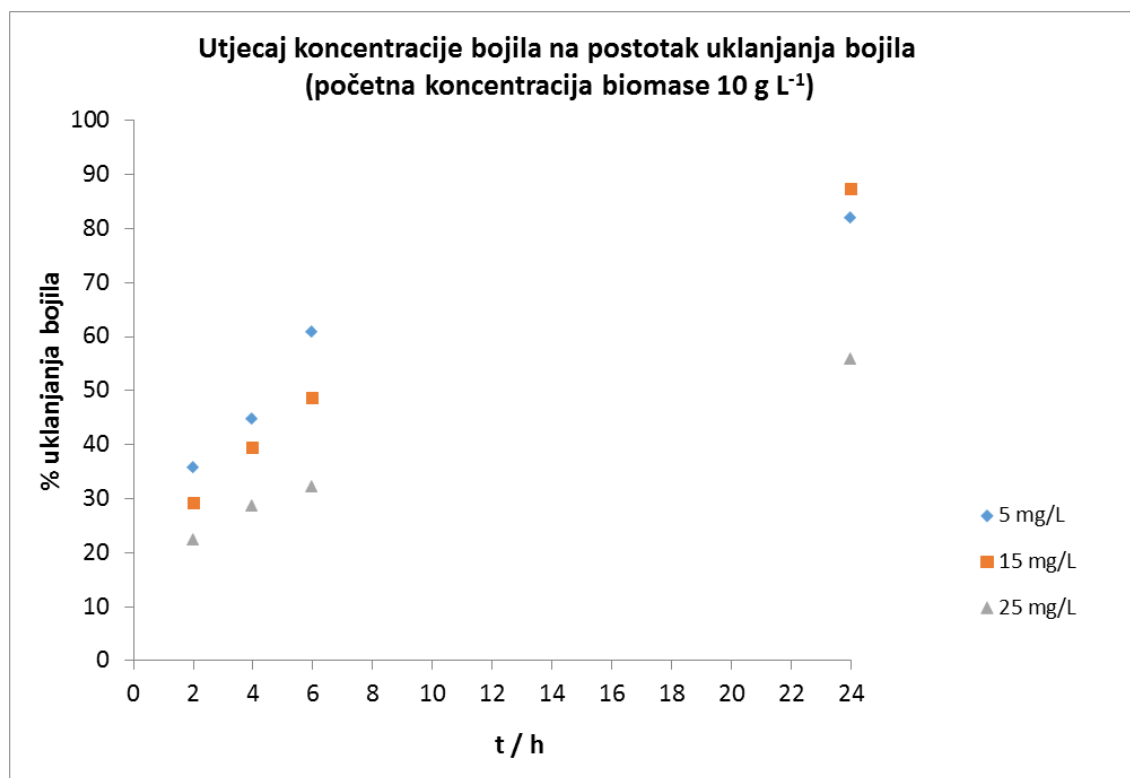
Slika 4.2. Utjecaj koncentracije bojila na postotak uklanjanja bojila ( T = 25 \text{ }^{\circ} \text{C} , n = 120 \text{ okr min}^{-1} , \gamma_{\text{biomasa}} = 10 \text{ g L}^{-1} )
