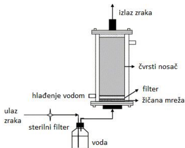
Slika 2 Shematski prikaz bioreaktora s nasutim slojem (prema Rodríguez Couto i Sanromán, 2006.)
