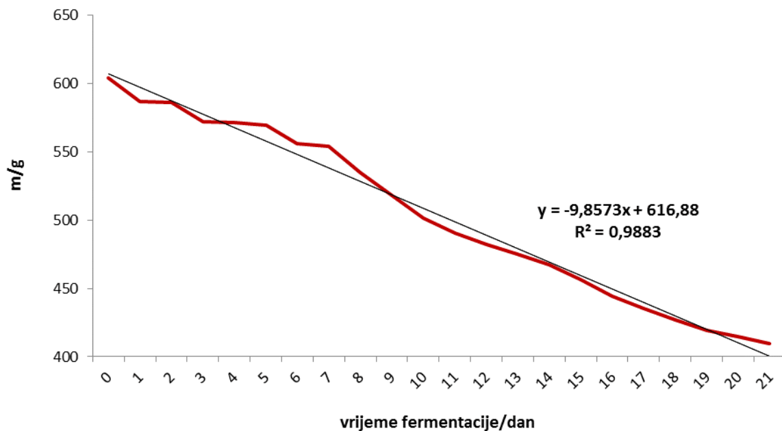
Slika 21 Promjena mase pivskog tropa obojenog kongo crvenilom tijekom fermentacije u laboratorijskom bioreктору
