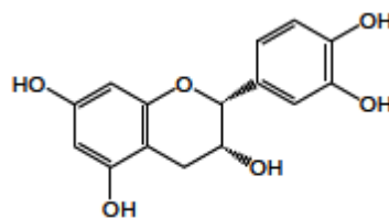
Epikatehin
