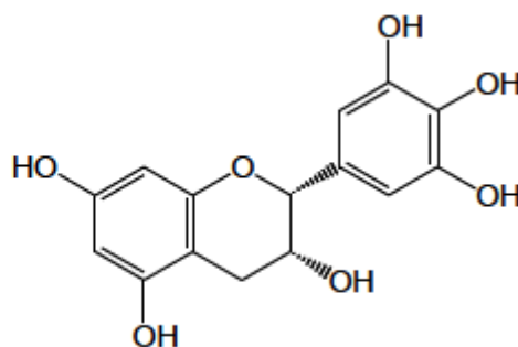
Epigalokatehin
