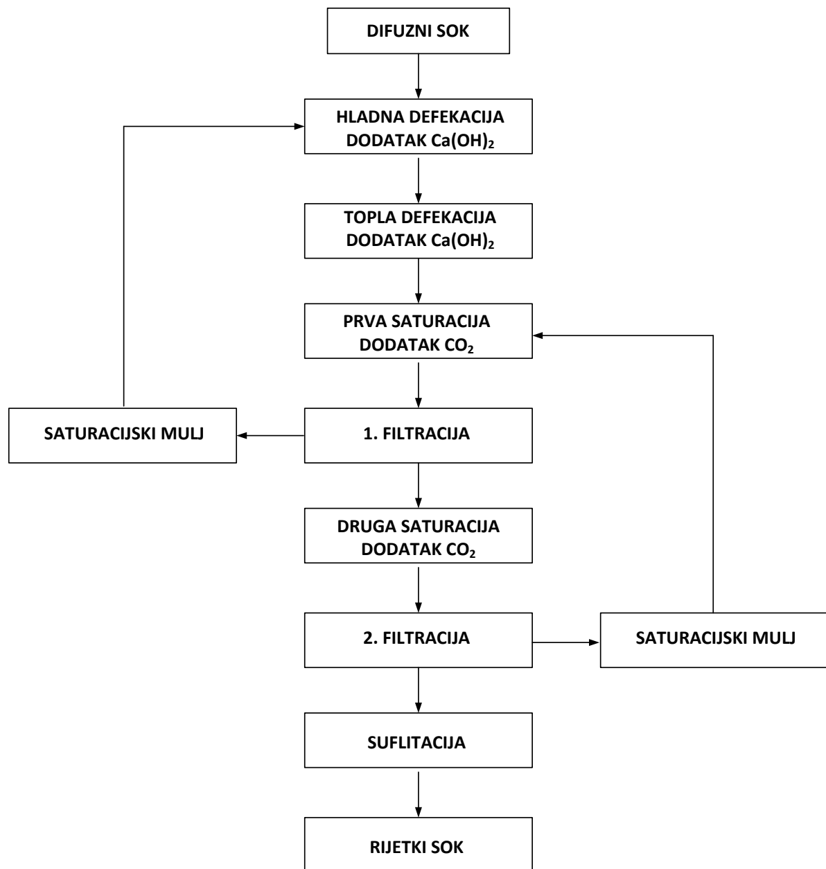
Slika 2 Tehnološka shema čišćenja difuznog soka
