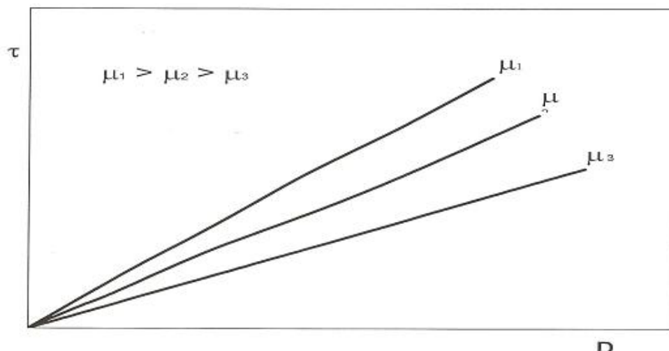
Slika 2. Newtonske tekućine
