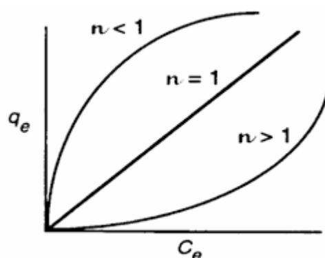
Slika 2 Freundlichova adsorpcijska izoterma pri različitim vrijednostima konstante n
