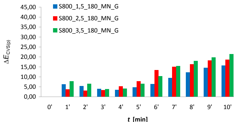
Slika 3 Ukupna promjena boje površine čajnog peciva pri temperaturi pečenja 180 °C i šećerom granulacije <800 μm
