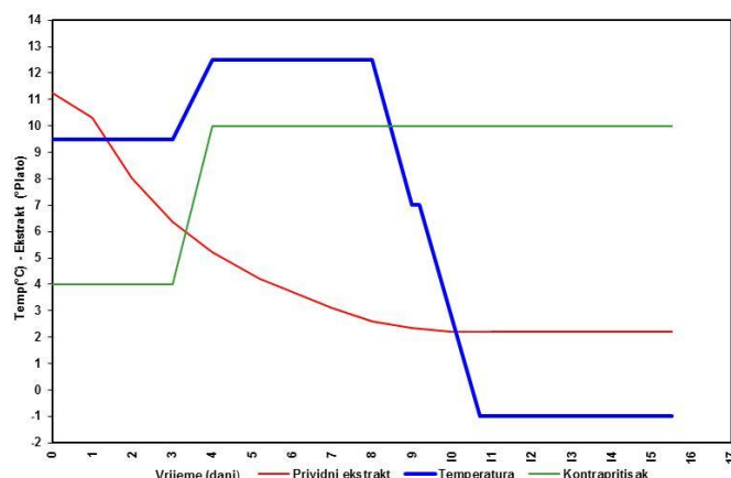
Slika 3 Diagram hladnoga vrenja i toplog dozrijevanja (ispitivano pivo)
