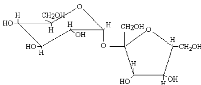
Slika 3 Strukturalni prikaz molekule saharoze (Šubarić i sur., 2011.)
