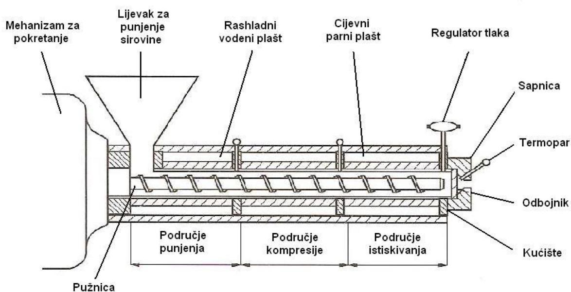
Slika 1 Princip rada jedнопužnog ekstrudera s odgovarajućim zonama (Jozinović, 2015)
