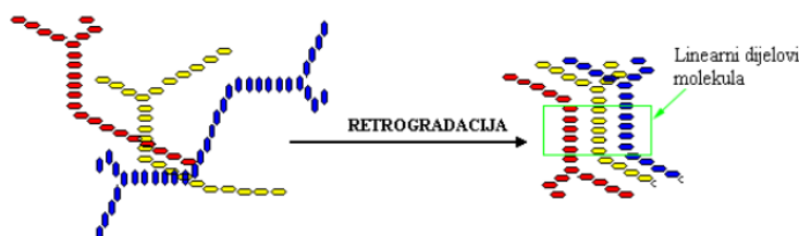
Slika 11 Retrogradacija otopljenih molekula škroba (Babić, 2011.)
