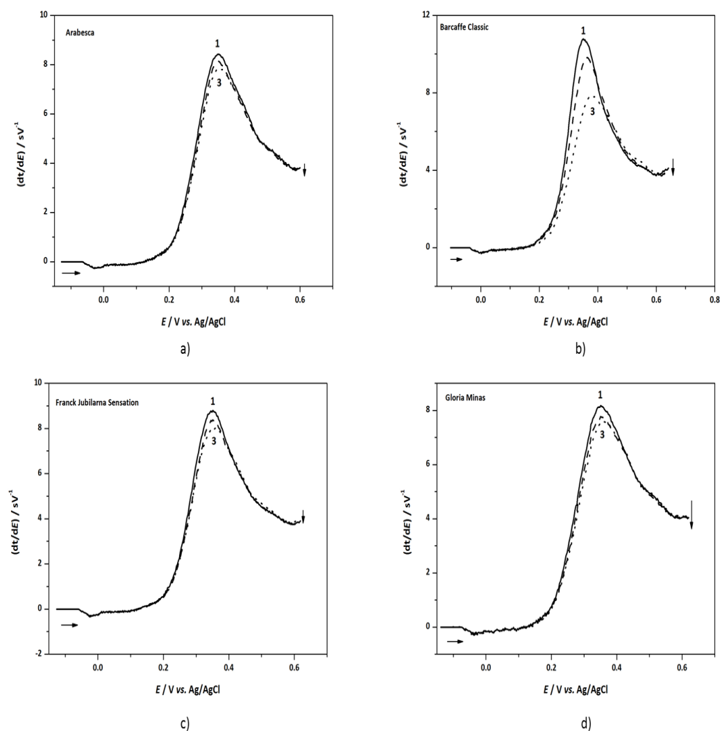
Slika 21 Utjecaj višestruke uzastopne polarizacije na FTS kronopotenciograme mljevene kave, (a) Arabesca, (b) Barcaffé Classic, (c) Franck Jubilarna Sensation i (d) Gloria Minas, (DF = 50), (DF = 50), u 0,1 \text{ mol L}^{-1} PBS pH 7,0. Eksperimentalni uvjeti kao u Tablici 2 (Eksperimentalni dio).
