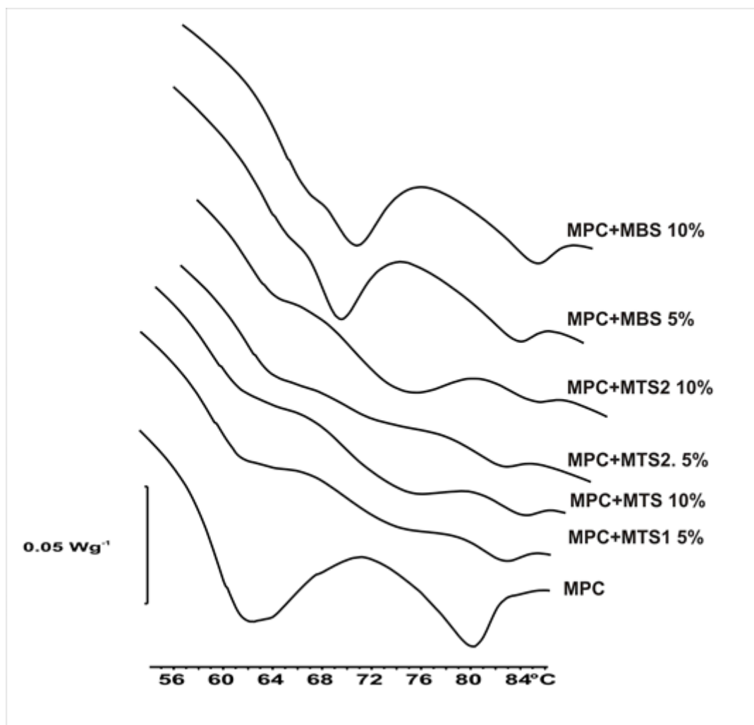
Slika 18 DMK termogrammi pilećeg surimija (MPC) s dodatkom modificiranih škrobova izoliranih iz tapioke (MTS1 i MTS2) i ječma (MBS), masenog udjela 5 i 10 %, nakon 30 dana skladištenja u zamrznutom stanju pri -30 °C
