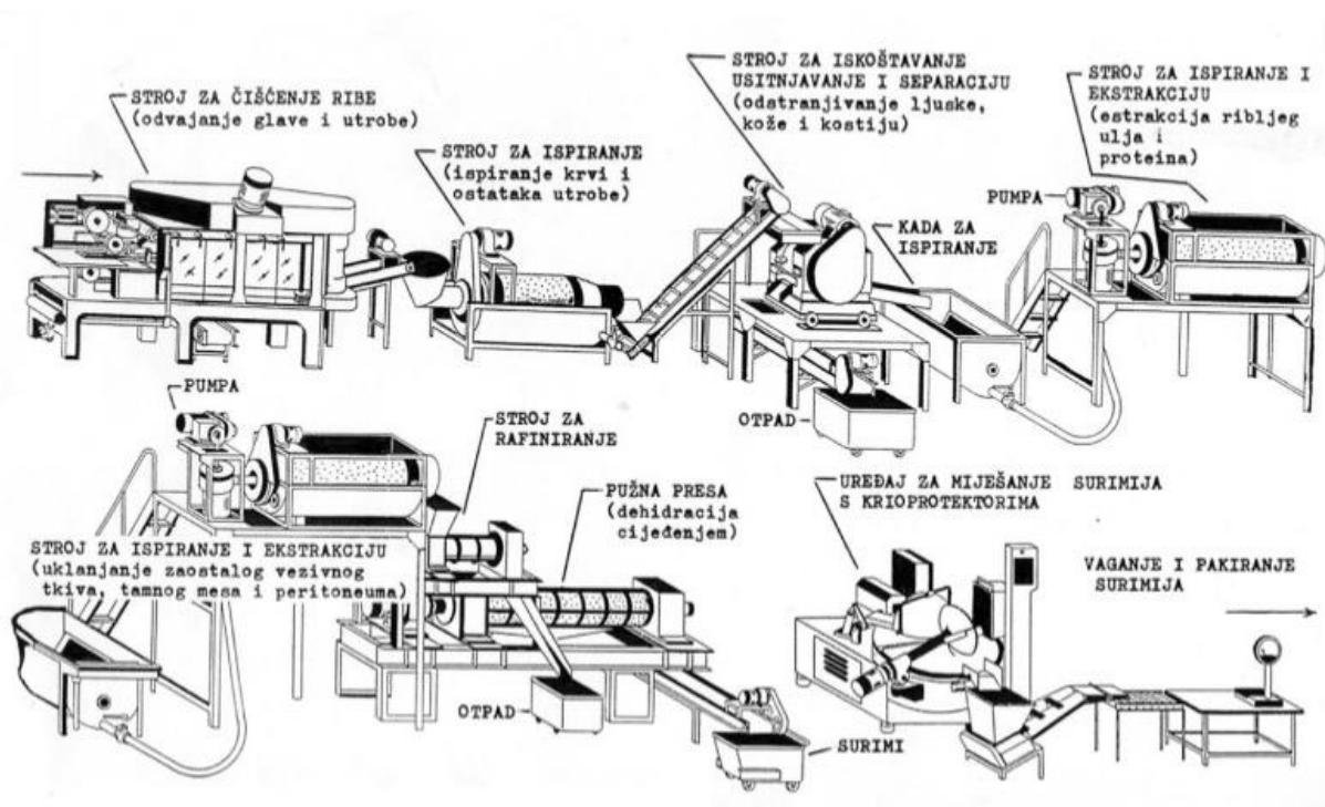
Slika 3 Tehnološka shema proizvodnje surimija (Kovačević, 2001.)
