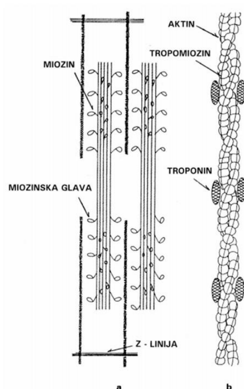
Slika 2 Shematski prikaz građe miofilamenata (a - građa miofibrila, b - građa tankih filamenata) (Karlson, 1998.)
